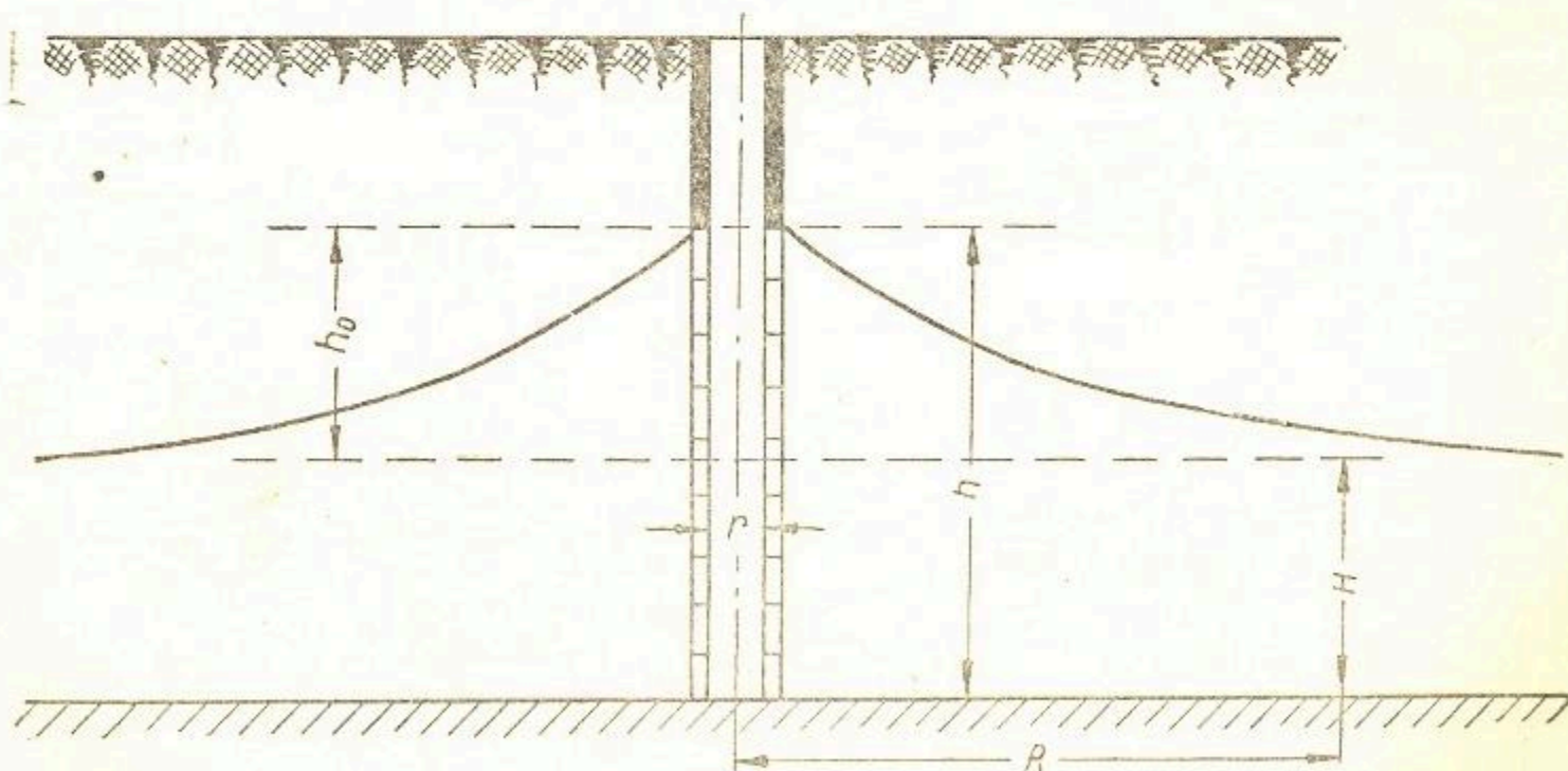
Рис. V — 93. Поглощающий колодец:
