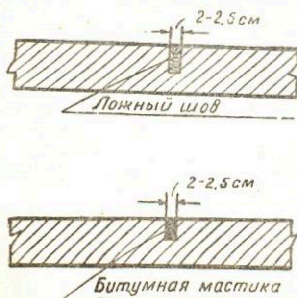
Рис. V—44. Ложные швы
