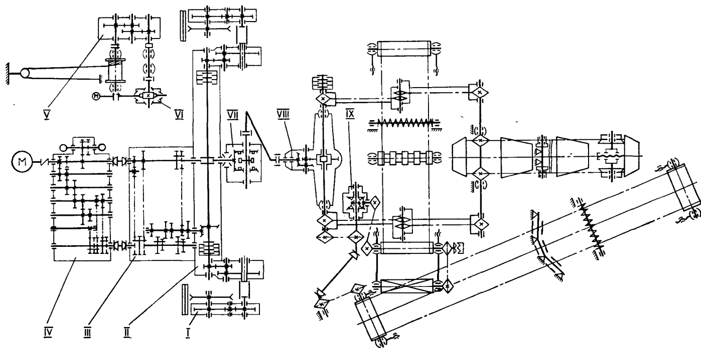
Рис. 120. Кинематическая схема экскаватора-дреноукладчика Д-659А
