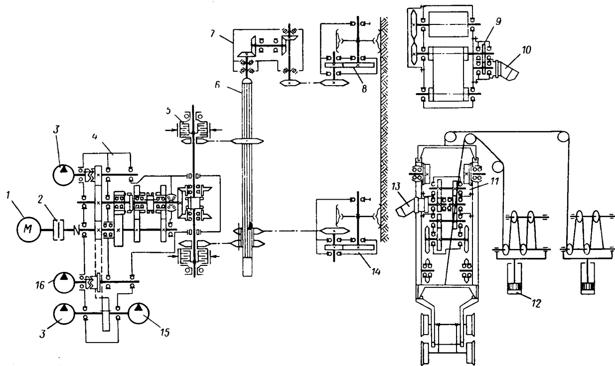
Рис. 127. Кинематическая схема экскаватора ЭМ-152Б
