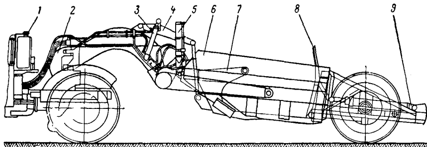
Рис. 54. Скрепер ДЗ-74
