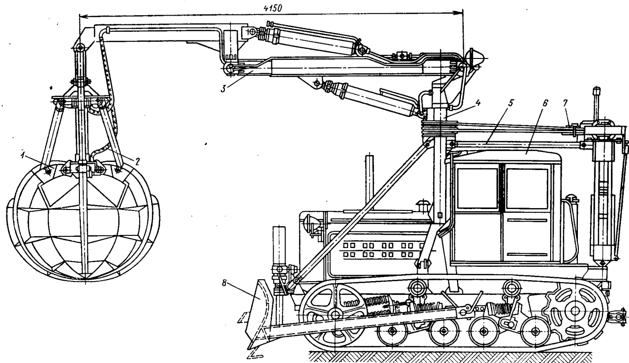
Рис. 19. Погрузчик МТТ-12(КТТ-1А)
