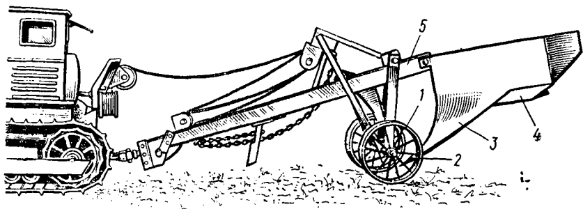
Рис. 94. Прицепной плужный каналокопатель Д-267А
