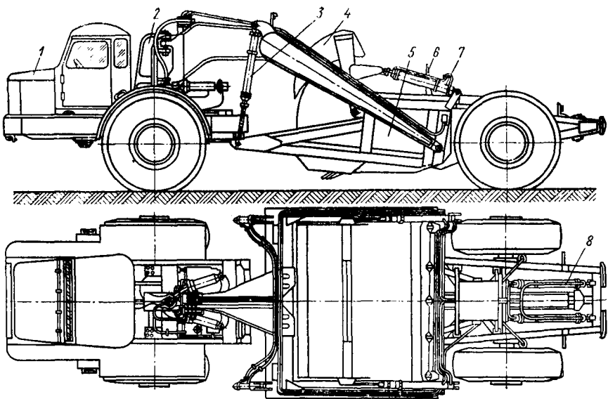
Рис. 55. Самоходный скрепер ДЗ-11 (Д-357М)
