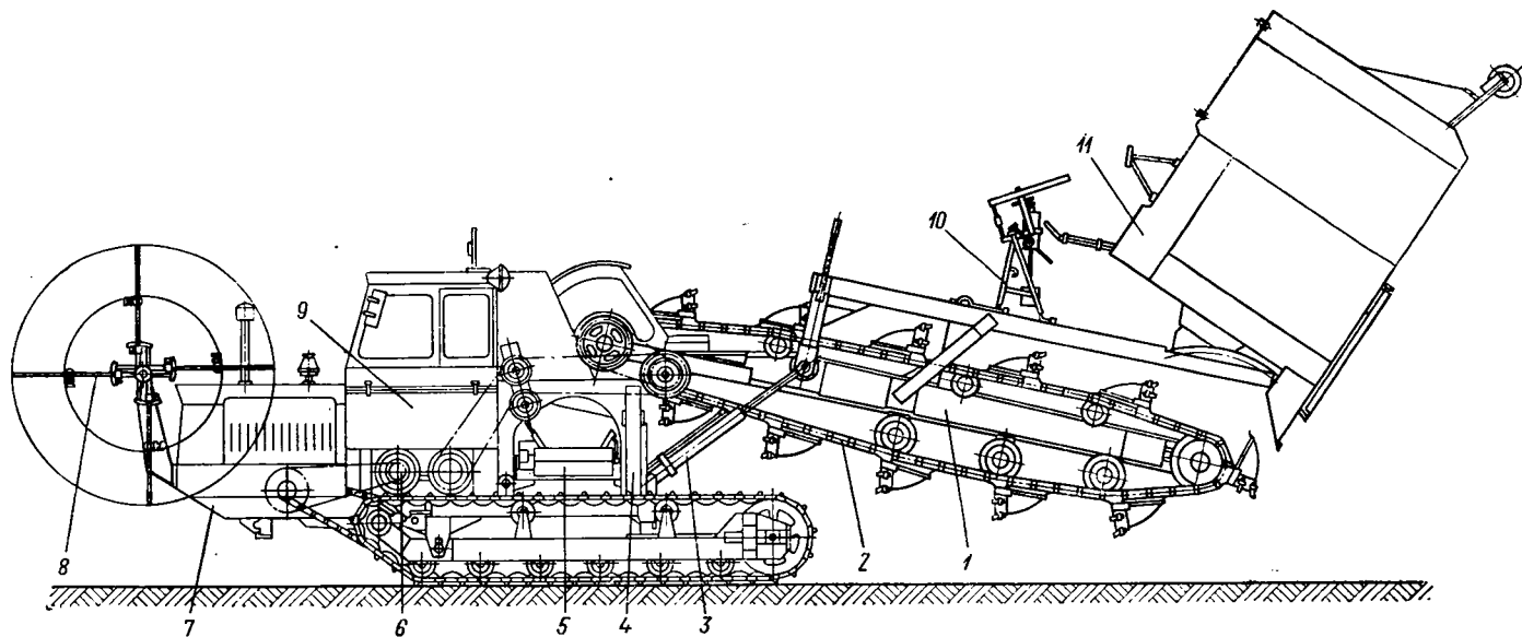
Рис. 110. Экскаватор-дреноукладчик ЭТЦ-202А
