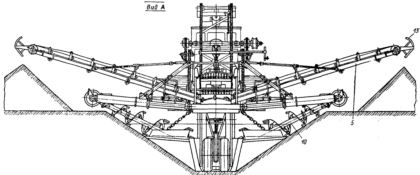
Рис. 100. Шнекороторный экскаватор ЭТР-201Б
