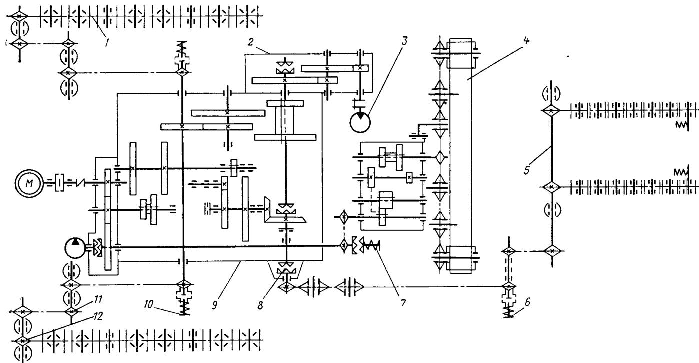
Рис. 111. Кинематическая схема экскаваторов-дреноукладчиков ЭТЦ-202 и ЭТЦ-202А
