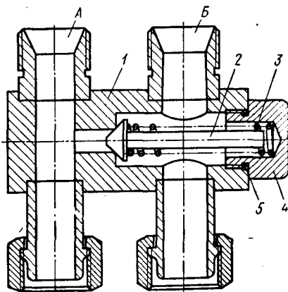
Рис. 62. Предохранительный клапан:
