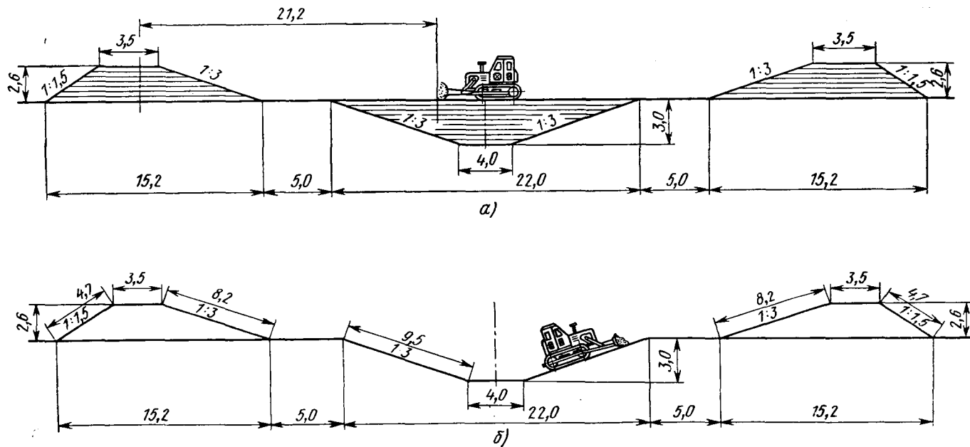
Рис. 23. Технологическая схема производства земляных работ по строительству канала оросительной сети: а — схема производства работ по открытию канала; б — схема планировочных работ
