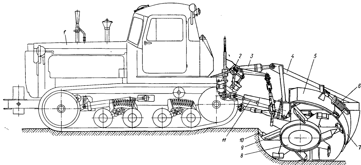
Рис. 96. Плужно-роторный каналокопатель МК-17
