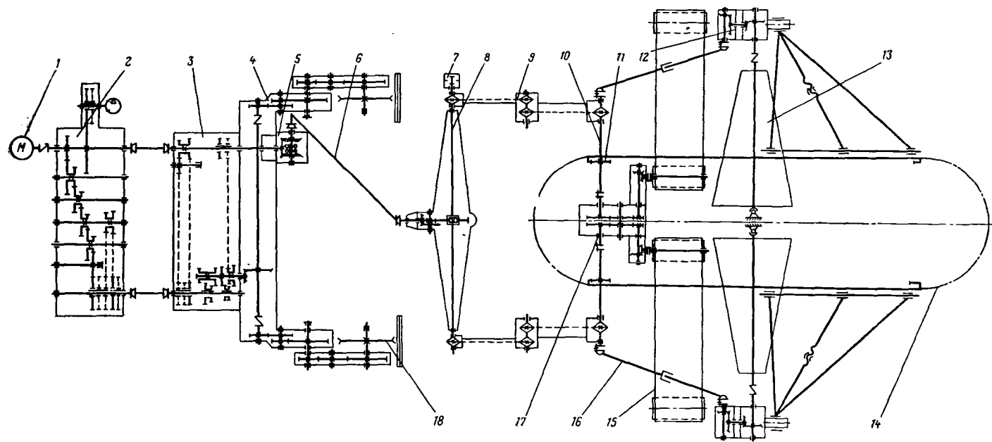
Рис. 101. Кинематическая схема экскаватора ЭТР-201Б
