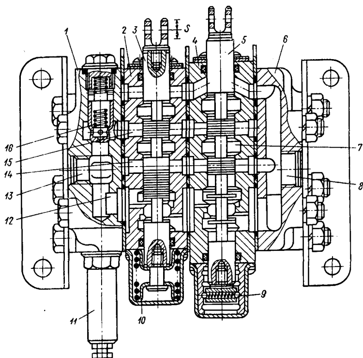
Рис. 150. Многосекционный распределитель
