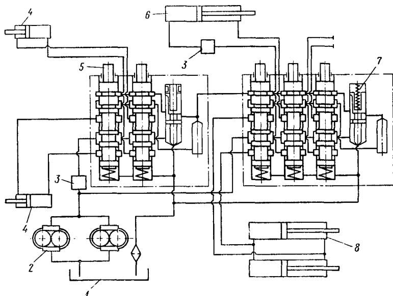
Рис. 37. Гидравлическая схема бульдозера-кавалероуразнителя Д-694А
