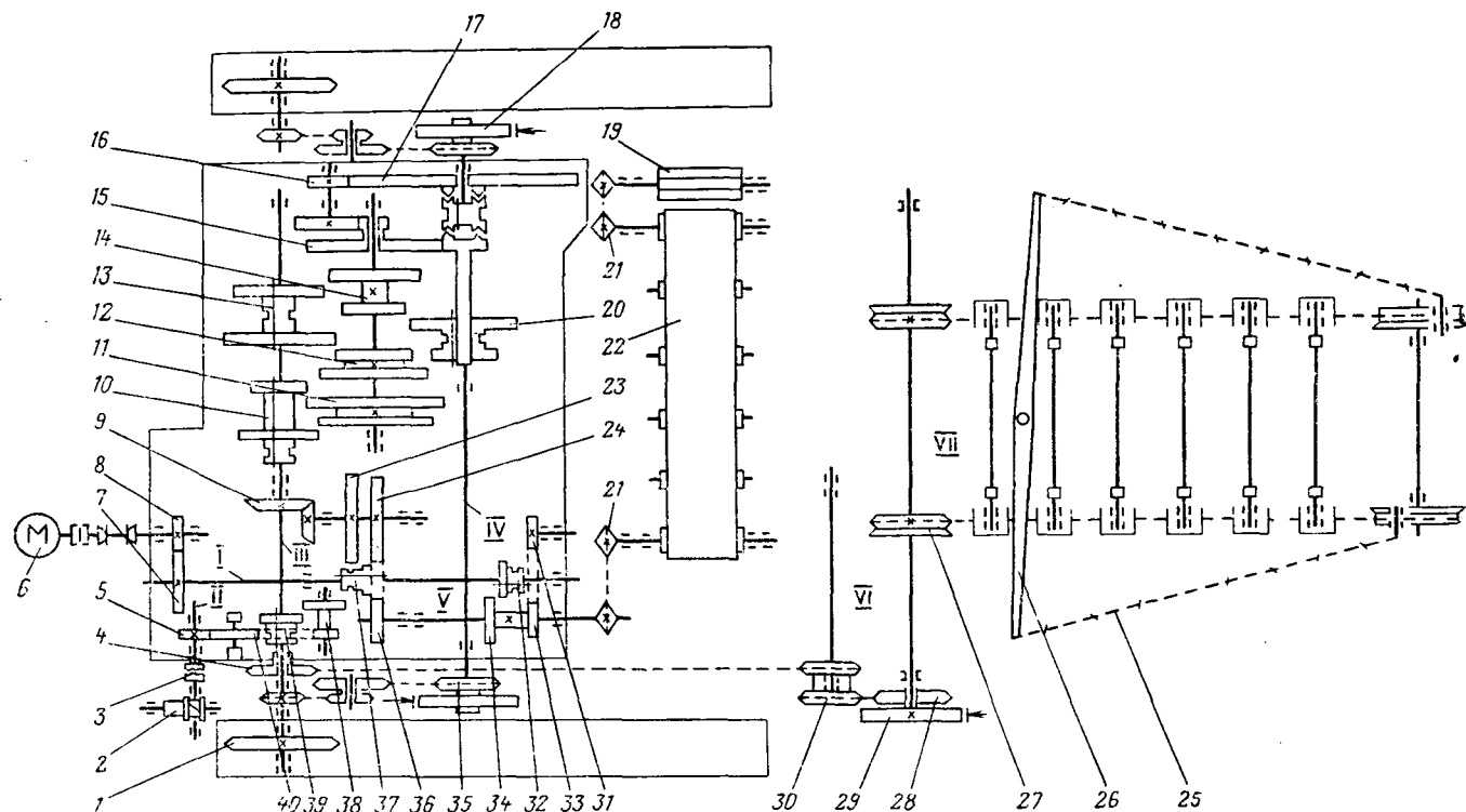
Рис. 107. Кинематическая схема экскаватора ЭТУ-354А:
