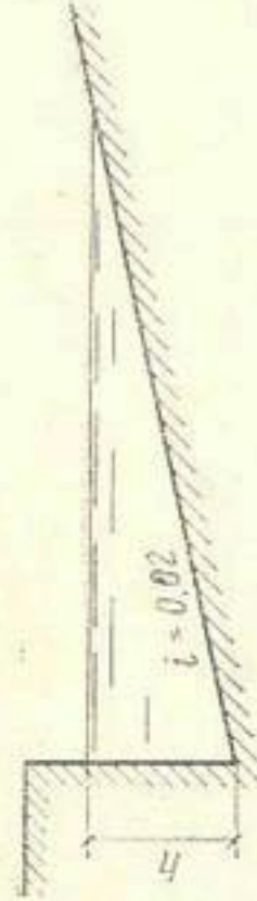
ЗНАЧЕНИЯ ГИДРАВЛИЧЕСКОГО РАДИУСА, М, МОДУЛЕЙ РАСХОДА, Л/С, СКОРОСТИ, М/С, ДЛЯ ТРЕУГОЛЬНОГО ЛОТКА
