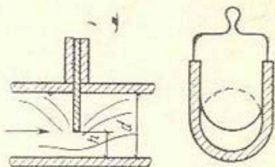
Рис. 19. Схема задвижки
