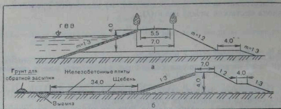
Рис. 11. Поперечные профили дамб:
