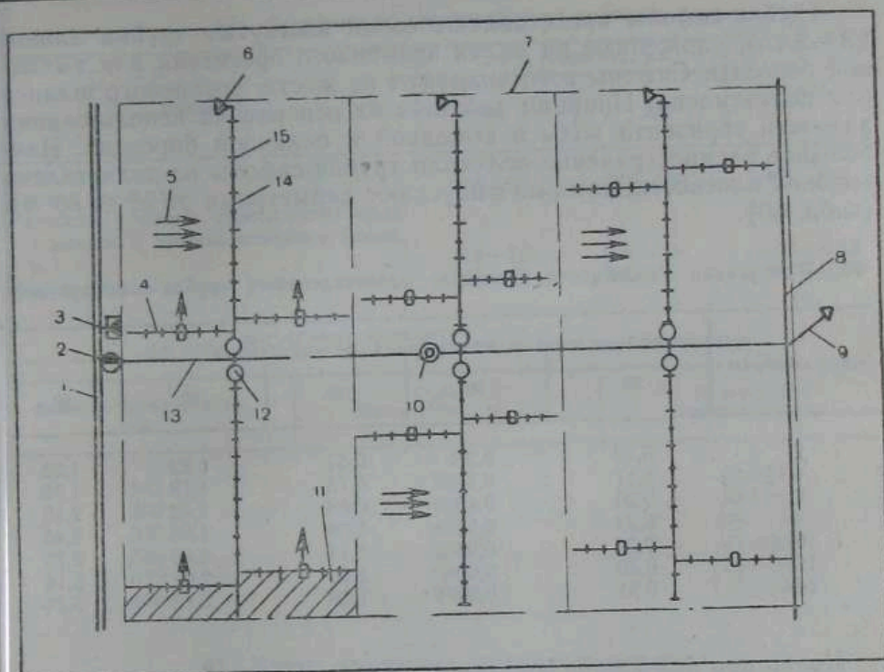
Рис. 20. Организация территории и схема оросительной сети с применением поливного колесного трубопровода ТКП-90:
