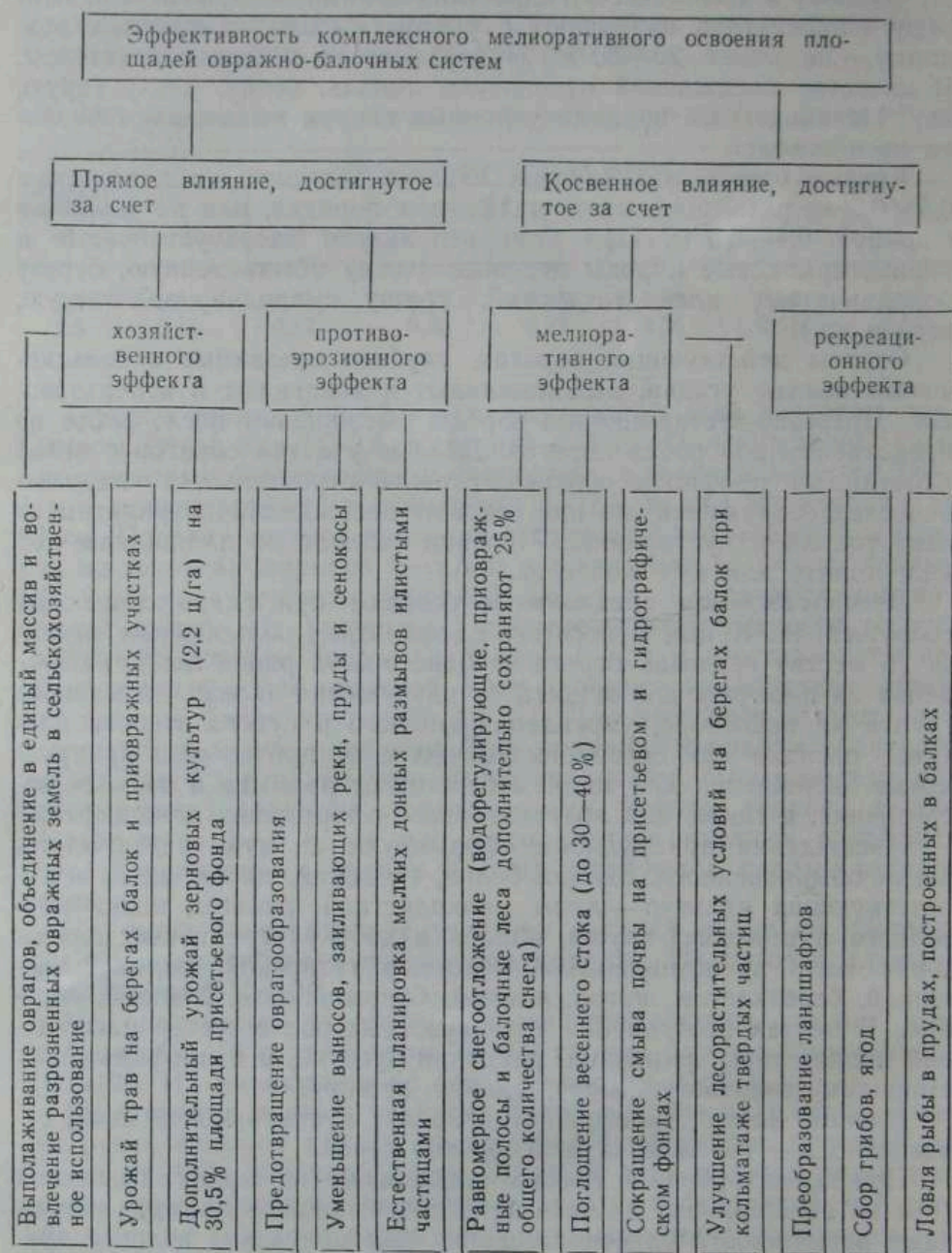
Рис. 51. Схема учета основных факторов эффективности мелиорации овражно-балочных земель
