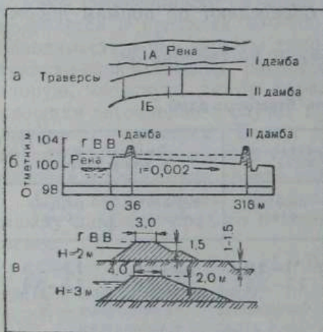
Рис. 11. Поперечные профили дамб:
