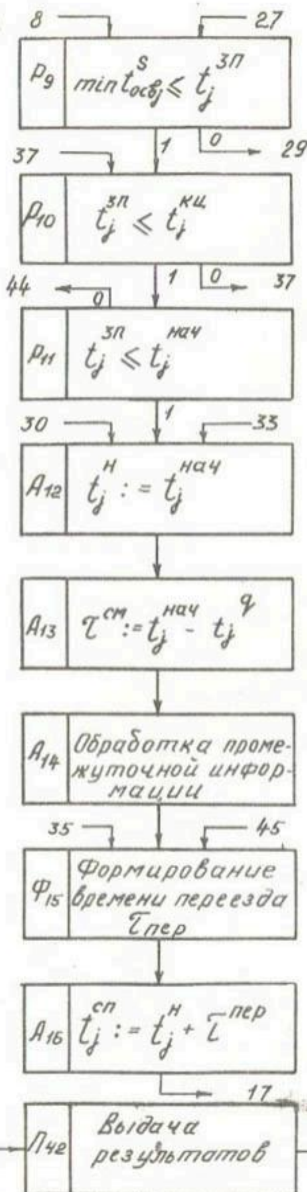
Схема алгоритма моделирования восстановления оборудования СВД.
