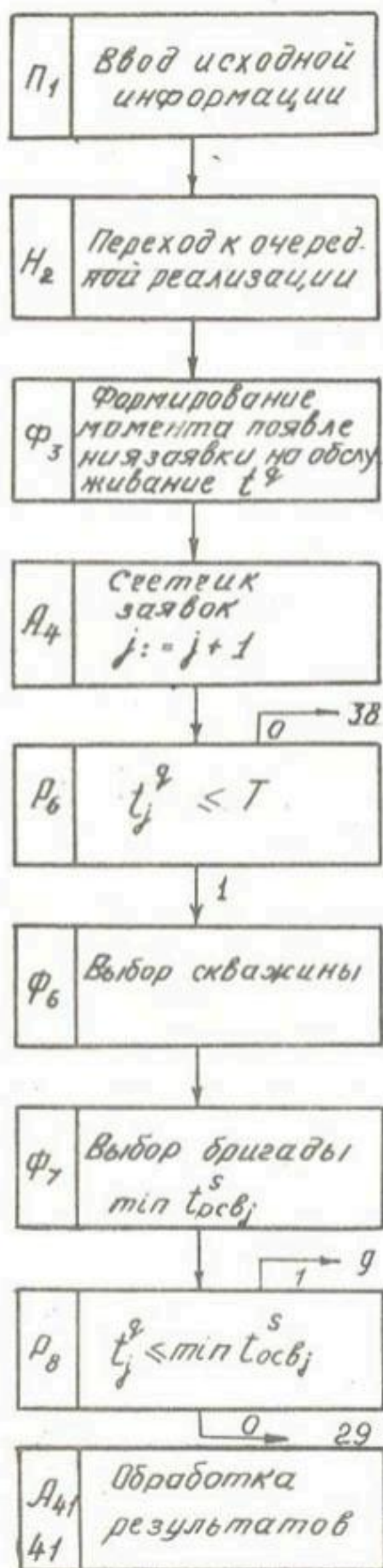
Схема алгоритма моделирования восстановления оборудования СВД.
