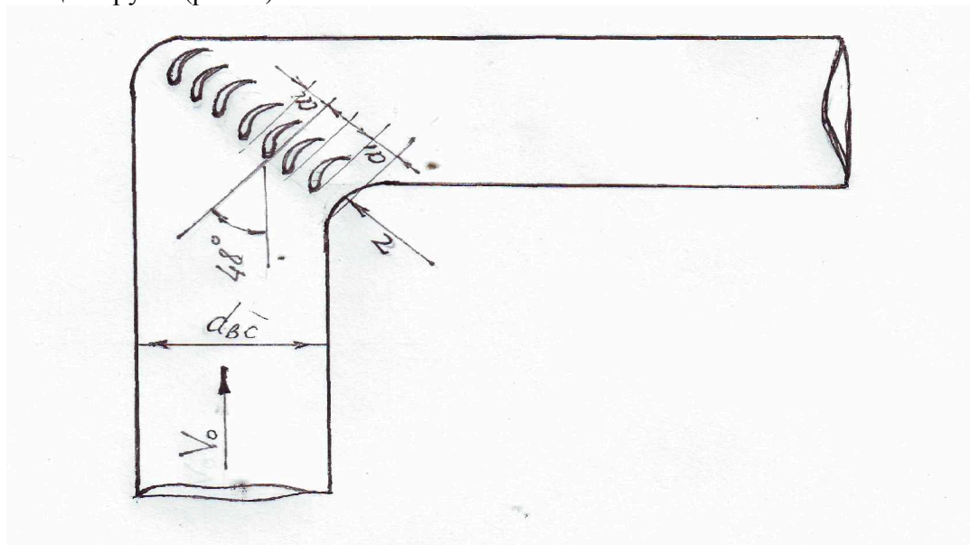
Рис. 2 - Колено вертикального всасывающего трубопровода с направляющими лопатками.
