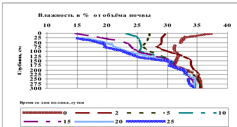
Рис. 2 - Режим влажности легкосуглинистой почвы при близких грунтовых водах. (Данные режимных наблюдений института «Средазгипроводхлопок»)
