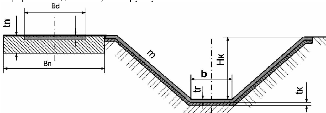
Рис. 1 - Конструкция противофильтрационного экрана из местных материалов b -ширина по дну канала; t k - толщина противофильтрационного экрана; H k - строительная глубина канала; t n - толщина уплотненного по периметру канала грунта; B d -ширина инспекторской дороги; m - коэффициент заложения откоса
