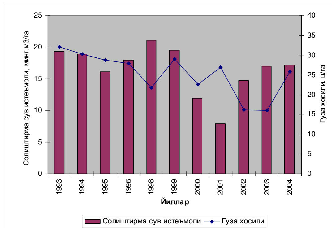
4 расм - Солиштира сув истеъмолининг ғўза ҳосилдорлигига боғлиқлиги
