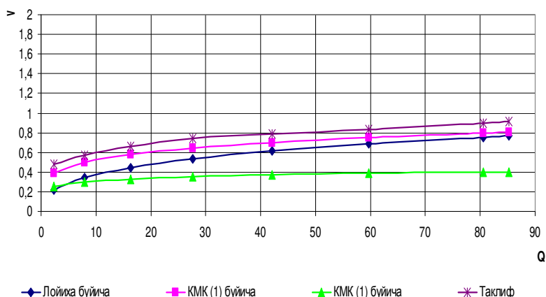
Расм 2 - Канал гидравлик элементларининг сув сарфига боглик равишда узгариши графиги
