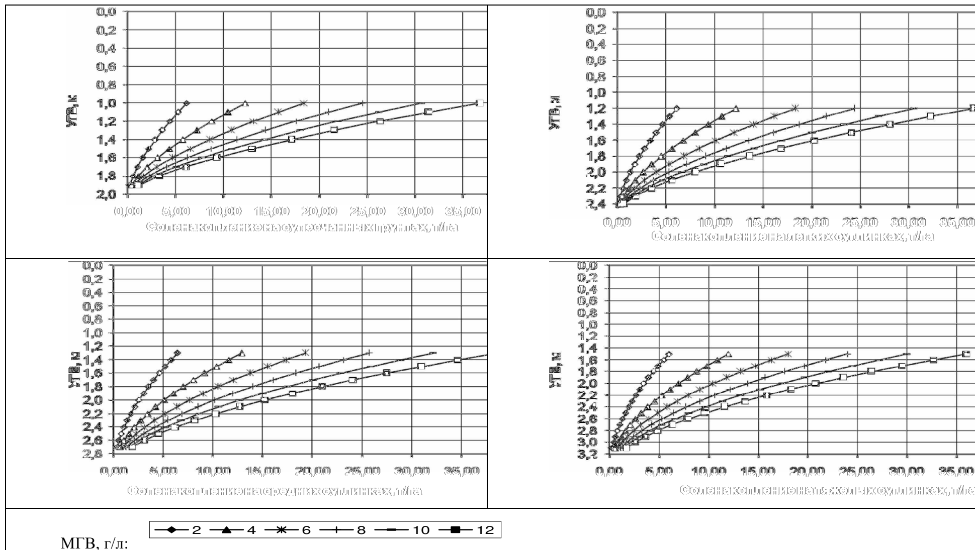
Рис. 1 - Графики соленакопления в зоне аэрации на различных по механическому составу почвогрунтах в зависимости от уровня и минерализации грунтовых вод на примере Сырдарьинской области.
