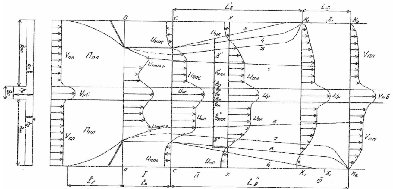
Рис. 1 - Схема растекания потока за поперечными пойменными дамбами ( n_{nl} \neq n_{nn} ), несимметричное растекание)
