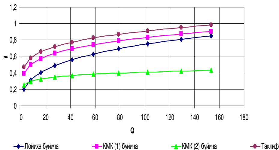
Расм 1 - Канал гидравлик элементларининг сув сарфига боглик равишда узгариши графиги
