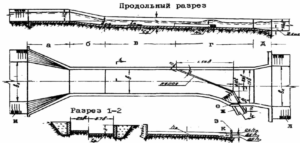
Рис. 2 - Новое устройство для защиты от наносов с донным порогом
