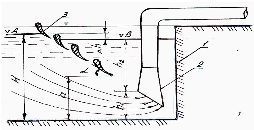
Рис. 1 - Водоприёмная камера с направляющими лопатками: 1-водоприёмная камера; 2-всасывающий трубопровод; 3-направляющие лопатки.
