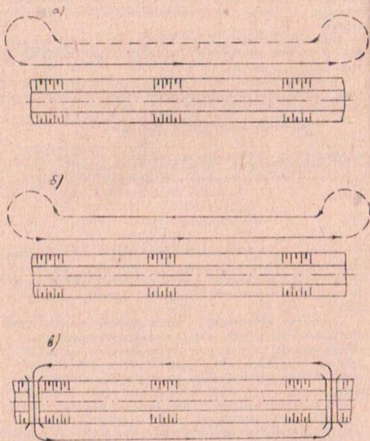
Рис. I. Траектории движения косилки: а — получелночная; б — челночная; в — колебная.
