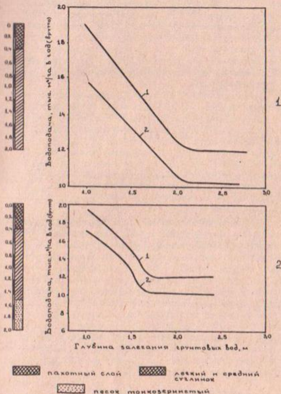
Рис.3. Зависимость вододачи от глубины залегания грунтовых вод при однослойном (1) и двухслойном (2) строении зоны аэрации и различных значениях КЦ внутрихозяйственной сети: 1 - КЦ 0,75 (на ближайшую перспективу); 2 - КЦ 0,88 (на отдаленную перспективу).
