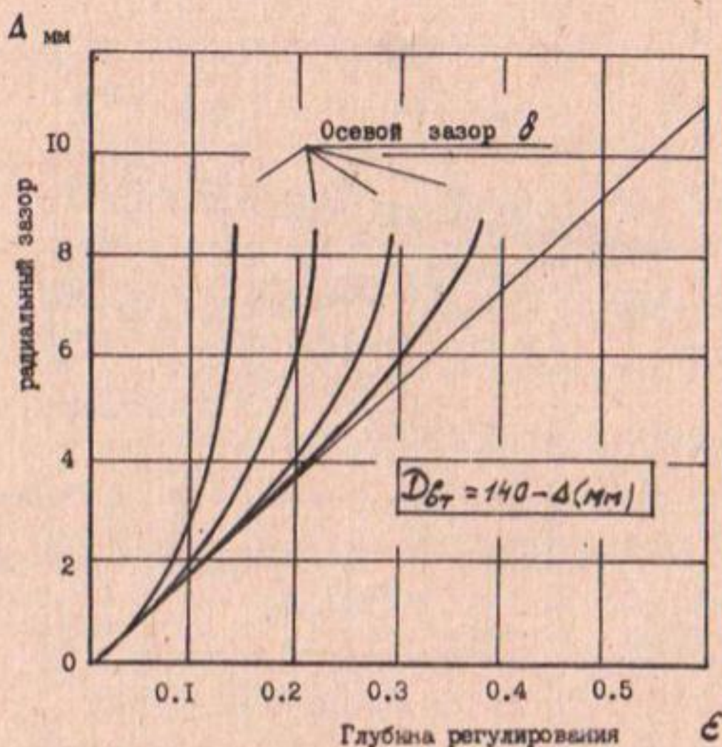
Рис. 4. Номограммы по выбору размера сменной калиброванной втулки осевого зазора между корпусом насоса и колесом для электронасоса 2ЭНВ12-255-30Г.
