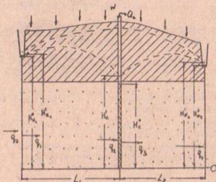
Рис. 2. Схема к расчету вертикального дренажа в условиях дренажного действия коллекторов, расположенных на различных отметках и имеющих разные фильтрационные сопротивления.
