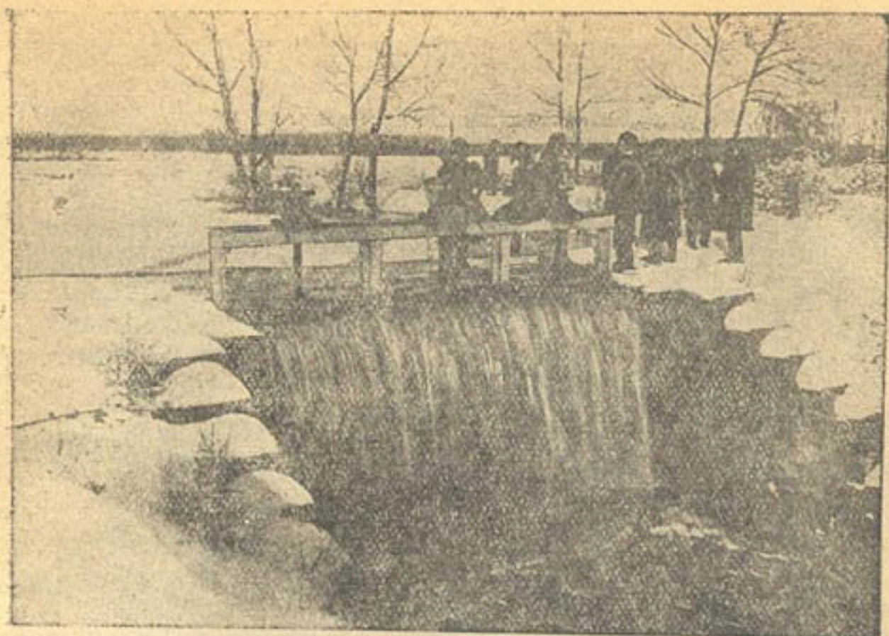
Рис. 2. Перелив воды через щиты головного регулятора АГЭС. Январь, 1935 г. Фото Попова.
