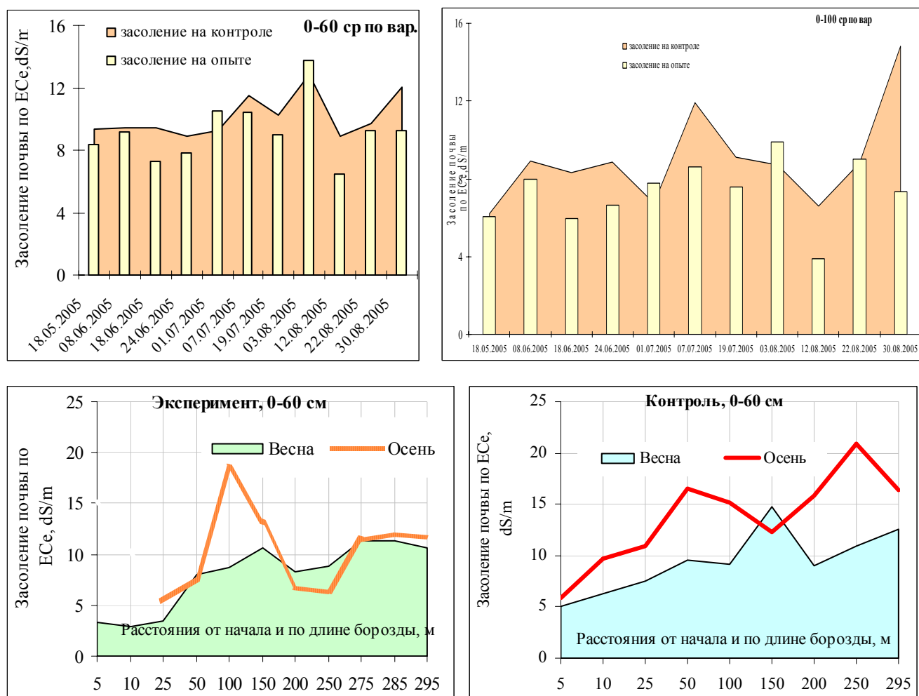
Рисунок 3 - Изменение засоление почвы по периодам наблюдений и по длине поля за вегетацию 2005 года
