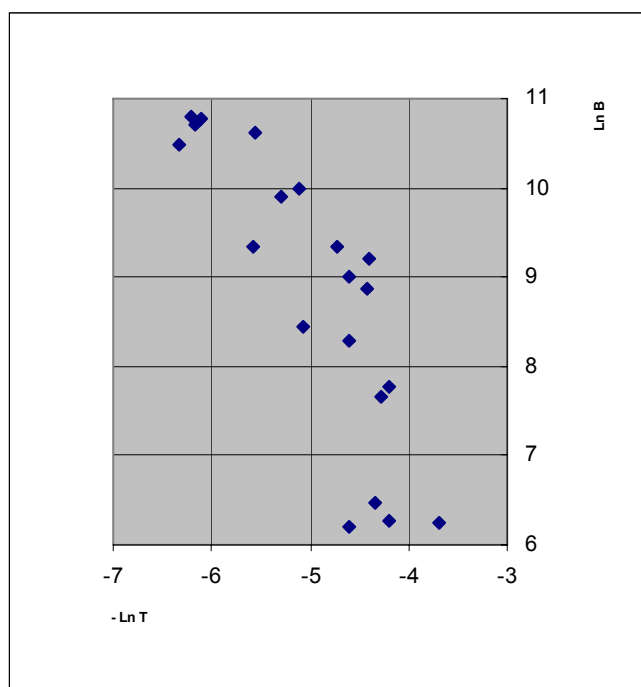
Рис. 2. Зависимость параметра В от водопроводимости по данным откачек разведочных скважин с диаметром бурения 12 1/4"-15" и скважностью фильтра 8-10%
