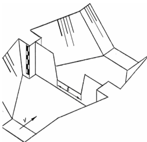
Водослив Чиполетти
