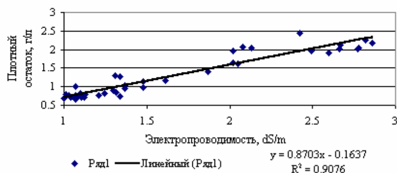
Рис. 6. Зависимость между электропроводимостью воды и плотным остатком, n=42 , r=0.953 (ЭП 1.0-2.86 dS/m, плотный остаток 0.672-2.44 г/л)
