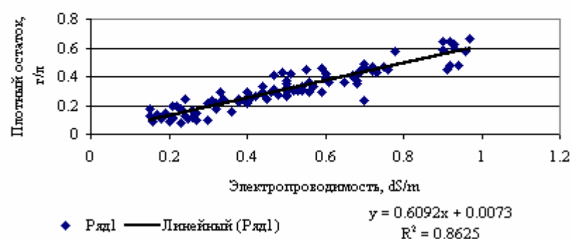
Рис. 5. Зависимость между электропроводимостью воды и плотным остатком, n=109 , r=0.929 (ЭП 0.15-0.97 dS/m и плотный остаток 0.074-0.66 г/л)
