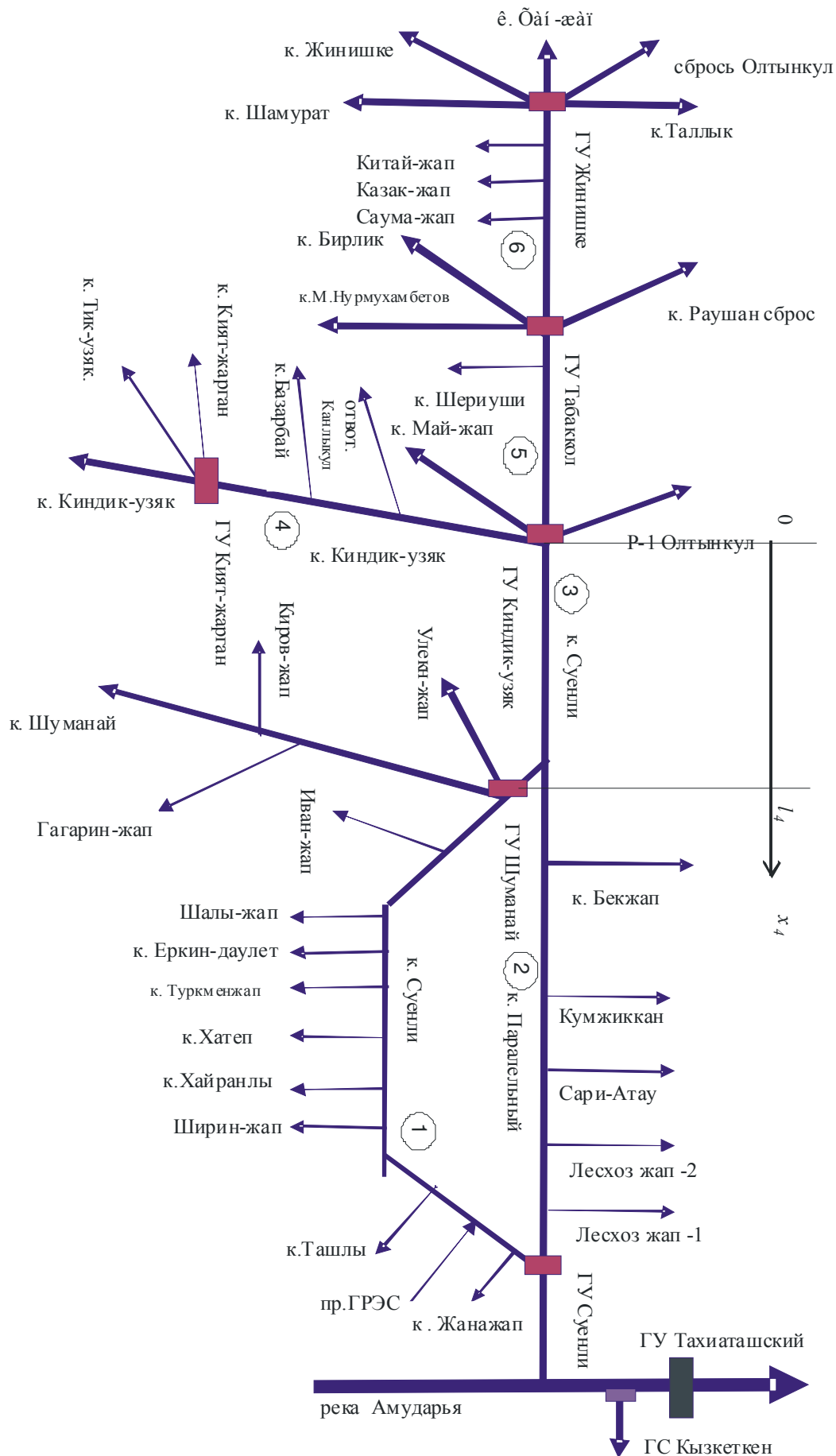
Рис. 1 Линейная схема магистральной части ирригационной системы Суенли
