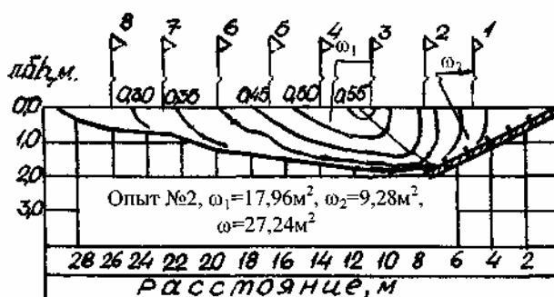
Рис.2. Распределение продольных скоростей потока в изотах (левая ветка Георгиевского магистрального канала, ПК91+50, ПК114)
