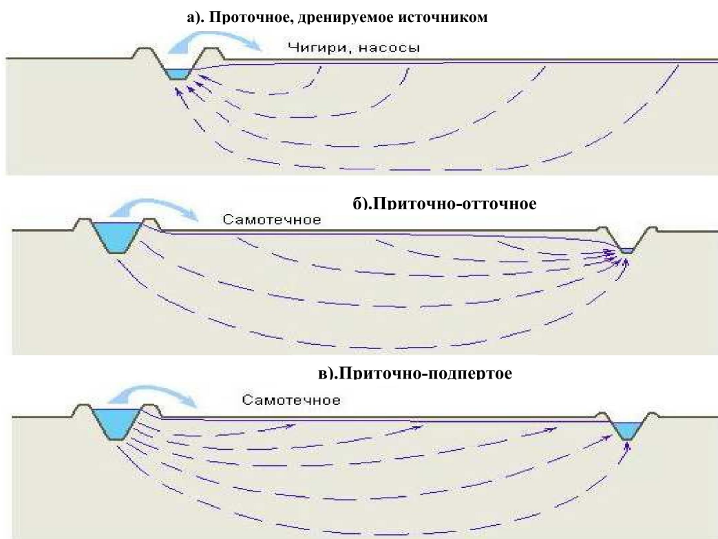
Рис. 1 Пути движения грунтовых вод в различных условиях подвода оросительной воды и отвода грунтовой ( а – случай заглубленных каналов и механического подъёма воды, б – при самотёчной водоподаче и работающей коллекторно-дренажной сети, в – при самотёчной водоподаче и затруднённом оттоке дренажно-сбросных стоков).
