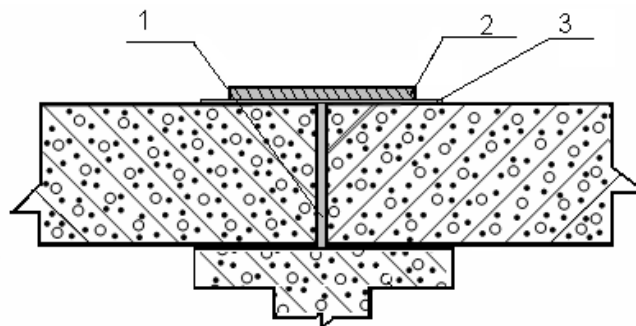
Рис. 1. Варианты уплотнения стыков-лотков
