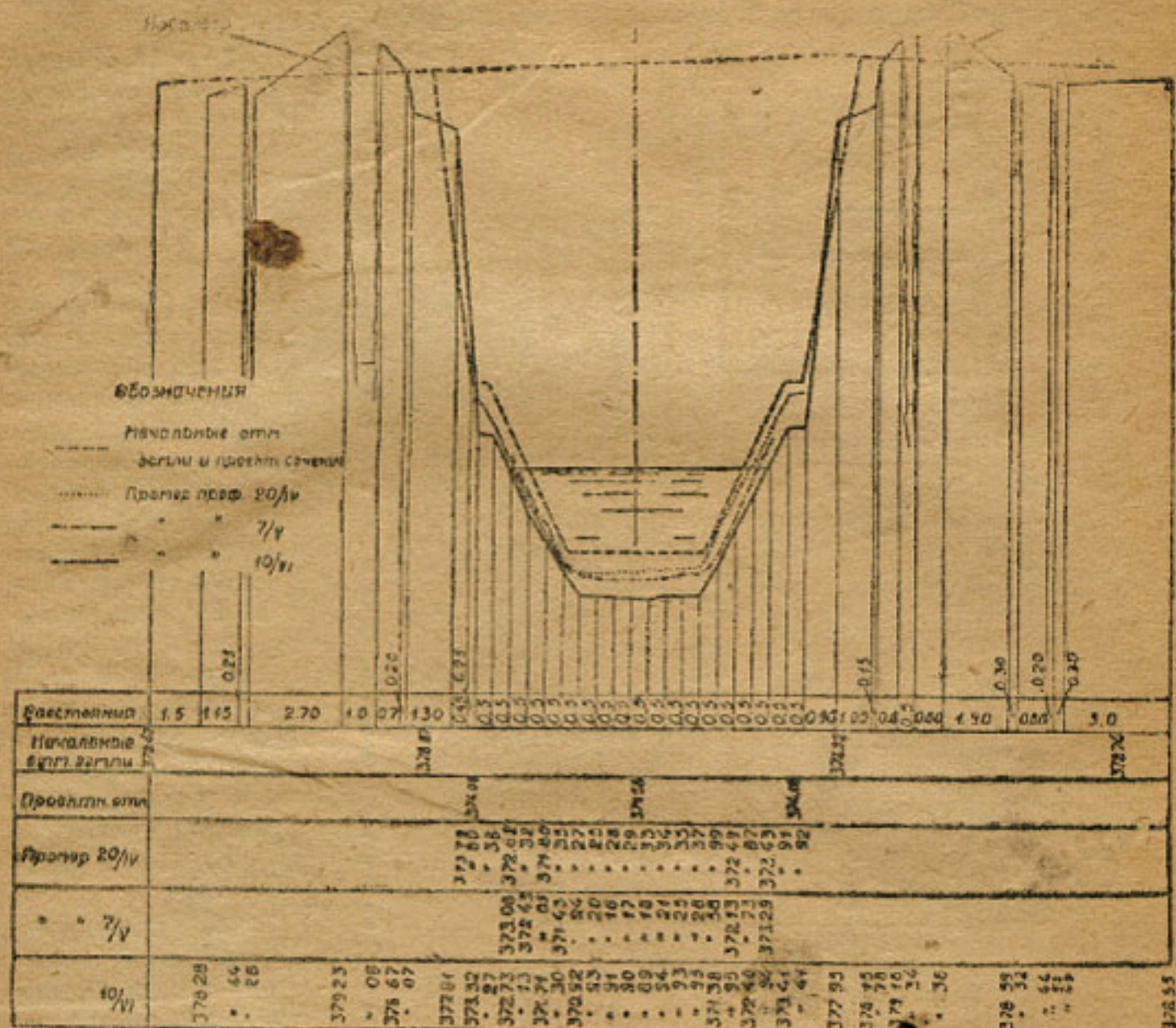
Рис. 18. Средний профиль участка Старого Джун.
