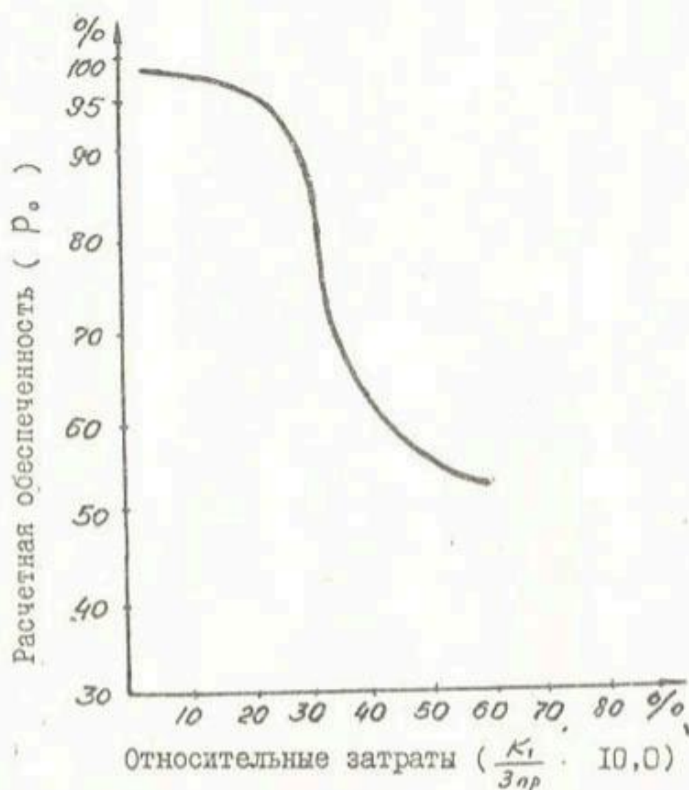
Рис. 2. Влияние размера изменяемой части затрат на выбор \beta :
