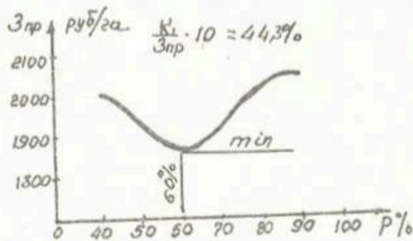
Рис. I. Зависимость расчетной величины P_c \% от соотношения \frac{K_1}{Зпр} .
