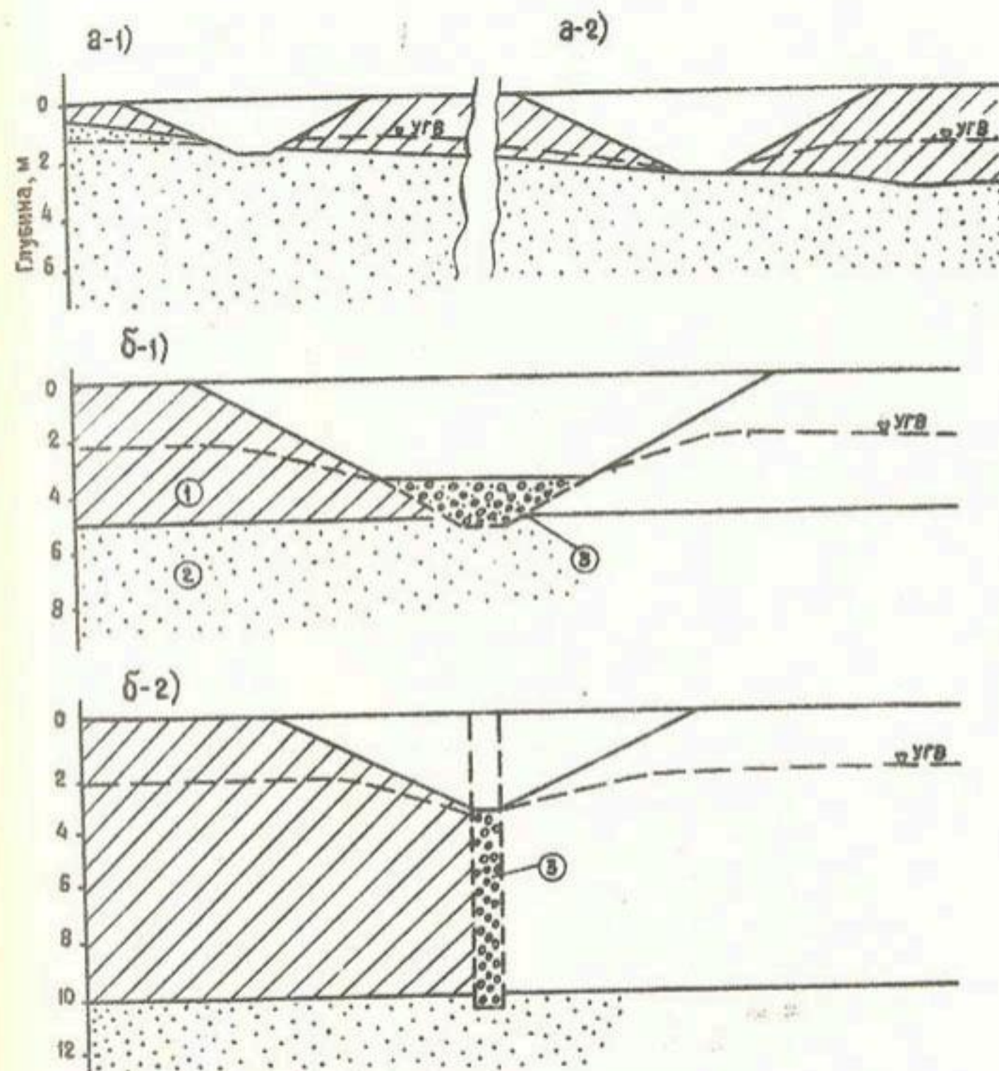
Рис.2. Схемы предлагаемых типов дренажа: а-1) - I тип, дрены глубиной 2 м, критическая глубина УГВ 1,5м; а-2) - I тип, дрены глубиной 2 м, критическая глубина УГВ 2...2,5м; б-1) - II тип, дрены с разгрузочными "окнами" в виде щелей; б-2) - II тип, дрены с разгрузочными "окнами" в виде круглых отверстий; (1) - глинистые грунты, (2) - пески, (3) - галечно-гравийные и щебенчатые грунты
