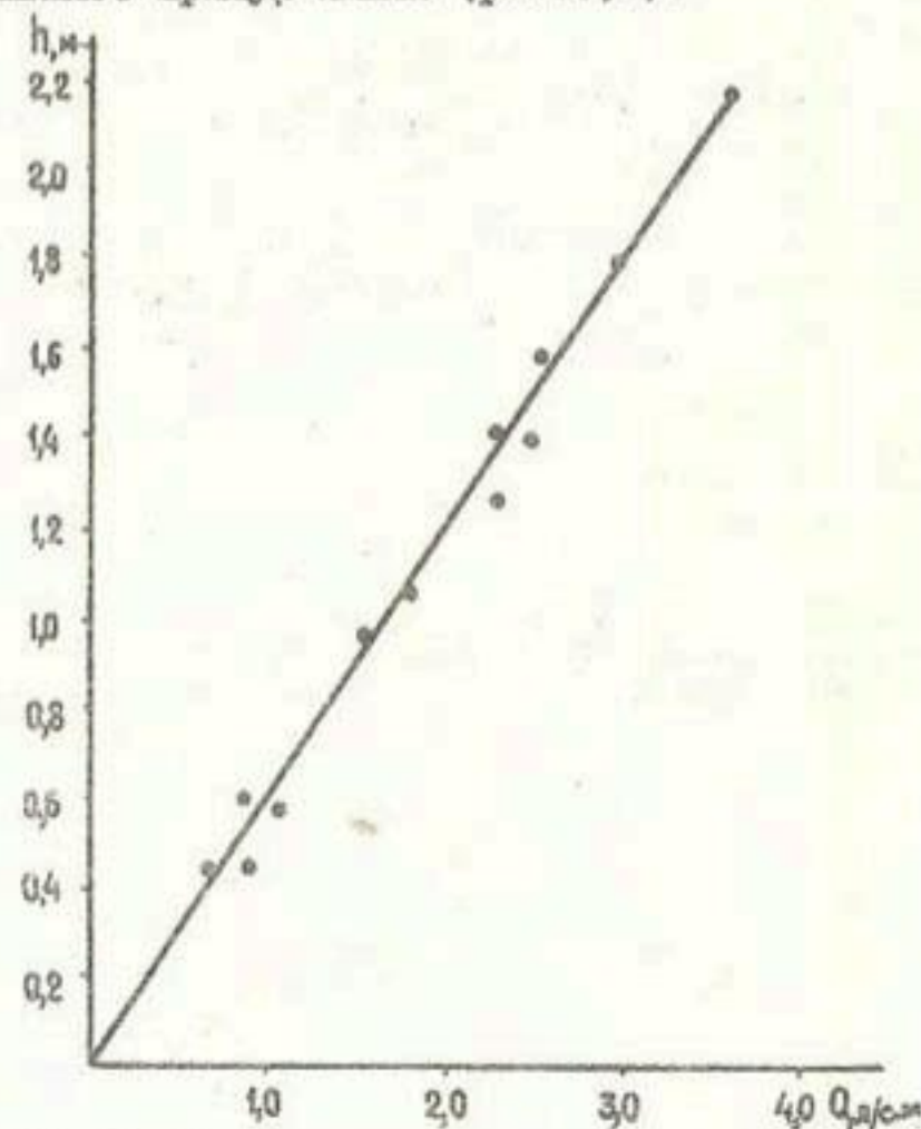
Рис.6. График зависимости расхода скважины-усилителя Q_y-I от действующего напора (По А.В.Толстуну)
