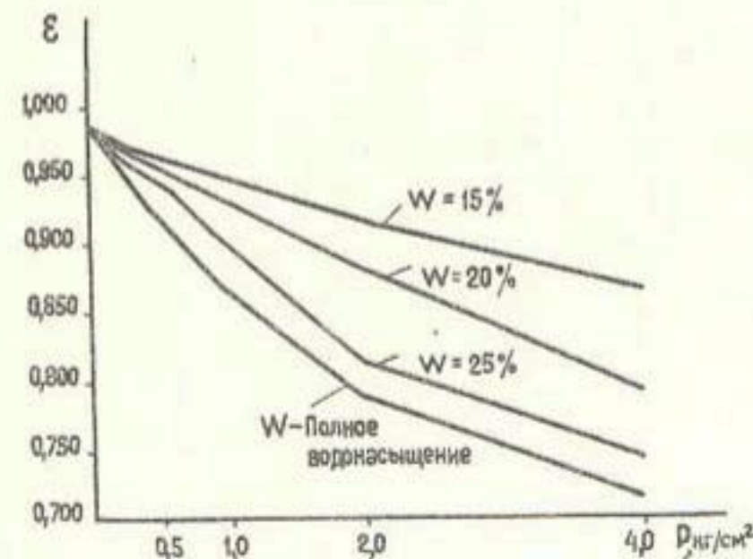
Рис.3. Кривые компрессионных испытаний грунтов при заданной влажности
