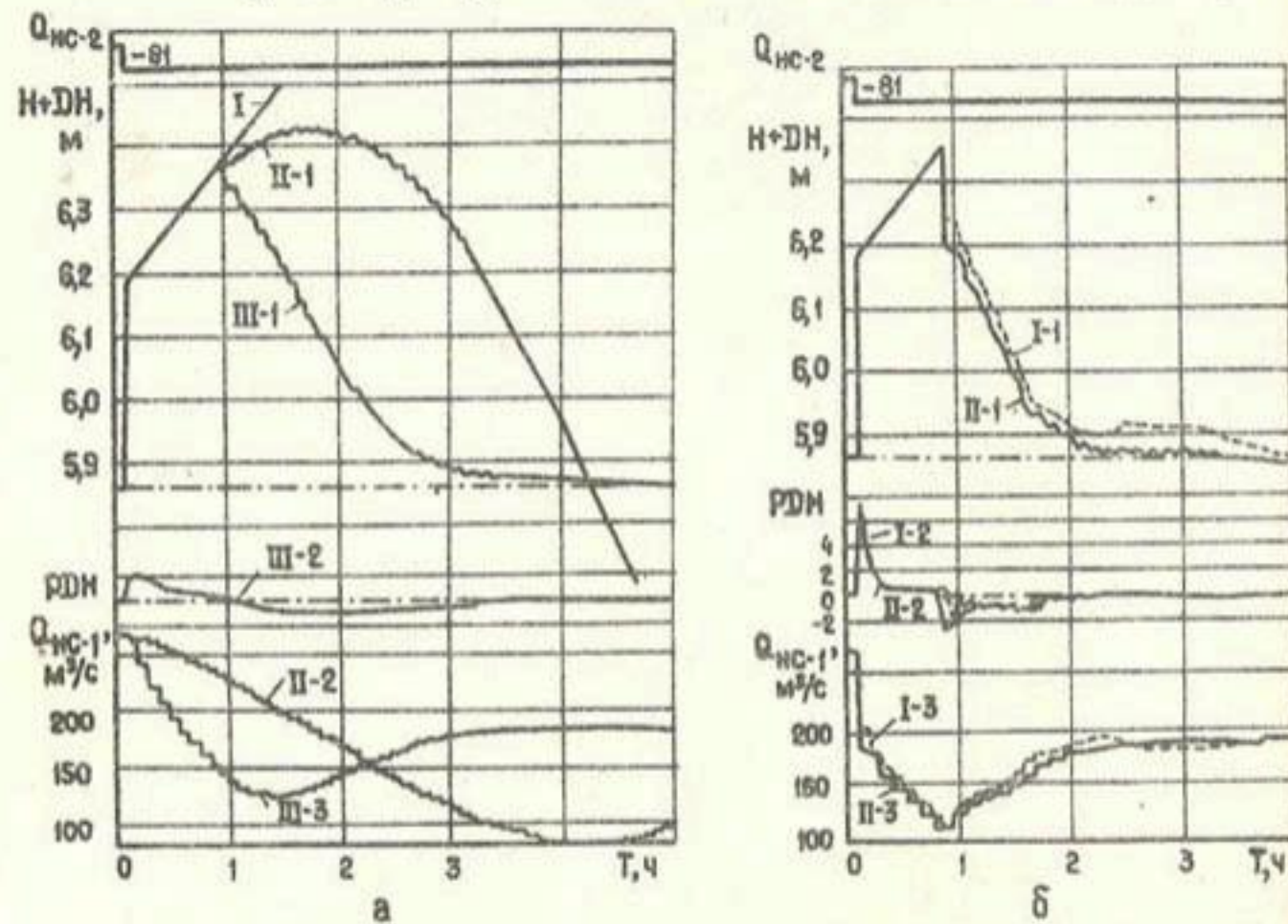
Рис.3. Графики переходного процесса автономной системы регулирования водоподдачи по нижнему бьефу с датчиком уровня в конце участка для НКМ (длина участка 20 км, расход 270 м³/с, возмущение \Delta Q_K = -8 \text{ м}^3/\text{с} = -30\% ): а) в локальном оптимуме: I – без регулирования; II – с регулятором "Янгир-2" ("Парус", ЛТК-133) при K_p=15 \text{ с/м} , T_p=300 \text{ с} ( J_2=48,2 \cdot 10^6 \text{ м} \cdot \text{с}^2 ), III – с регулятором "Янгир-5" при K_p=15 \text{ с/м} , T_p=300 \text{ с} , K_d=10 , T_d=180 \text{ с} ( J_2=12,78 \cdot 10^6 \text{ м} \cdot \text{с}^2 ); б) в локальных оптимумах с регулятором "Янгир-5": I – при K_p=15 \text{ с/м} , T_p=300 \text{ с} , K_d=90 , T_d=90 \text{ с} ( J_2=8,5 \cdot 10^6 \text{ м} \cdot \text{с}^2 ); II – при K_p=20 \text{ с/м} , T_p=450 \text{ с} , K_d=90 , T_d=90 \text{ с} ( J_2=6,6 \cdot 10^6 \text{ м} \cdot \text{с}^2 )
