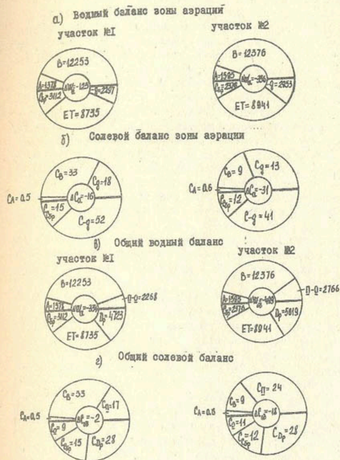
Рис.2. Диаграммы статей общего и частичного водно-солевого баланса, м 3 /га (среднее за 1978-1983 гг.): В — водоподача; А — осадки; (-q) — нисходящий ток поливных вод через зону аэрации орошаемого поля; Д р — дренажный сток; ET — эвапотранспирация; П-Q — разность подземного притока и оттока; ΔW — изменение запасов влаги в расчетном слое; C а , C б , C ±q , C д , C е , C др , C сгр — поступление или вынос солей соответствующими элементами водного баланса; C а , C сб — суммарное изменение запасов солей в зоне аэрации и на территории.
