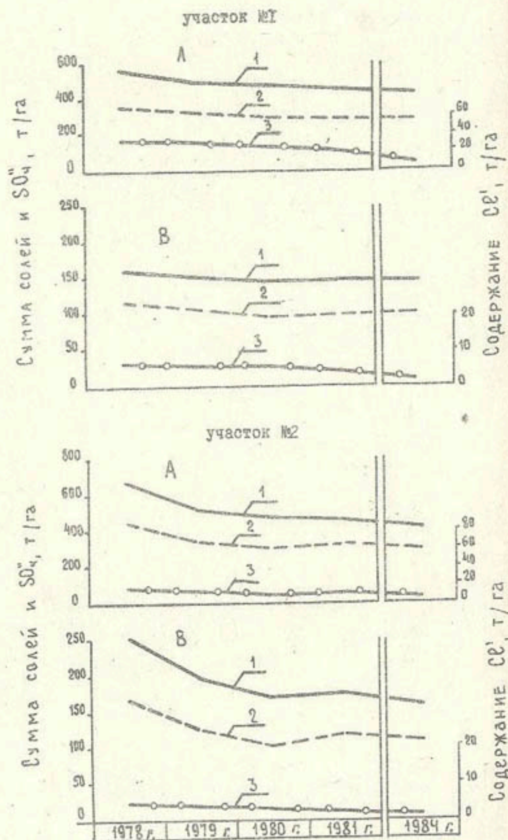
Рис.5. Интенсивность опреснения почвогрунтов на ОПУ, т/га А - в 3-метровом слое; В - в 1-метровом слое; 1 - сумма солей; 2 - сульфат-ион; 3 - ион хлора.
