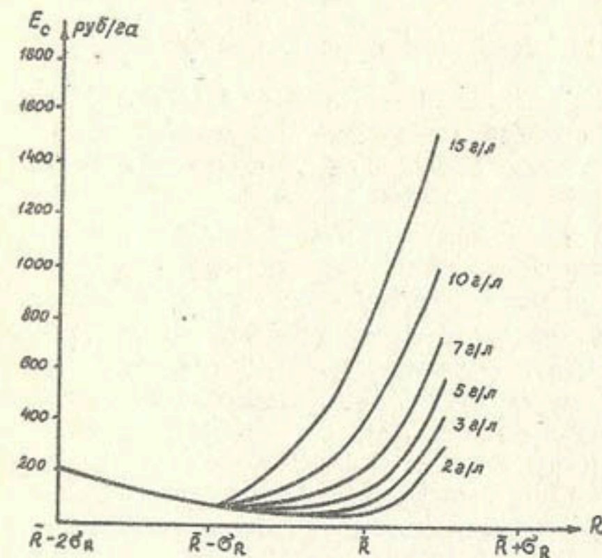
Рис.2. Зависимость экономической эффективности строительства вертикального дренажа от принятого запаса прочности междренного расстояния при различной минерализации грунтовых вод (изменчивость исходных параметров C_v = 20\% ).
