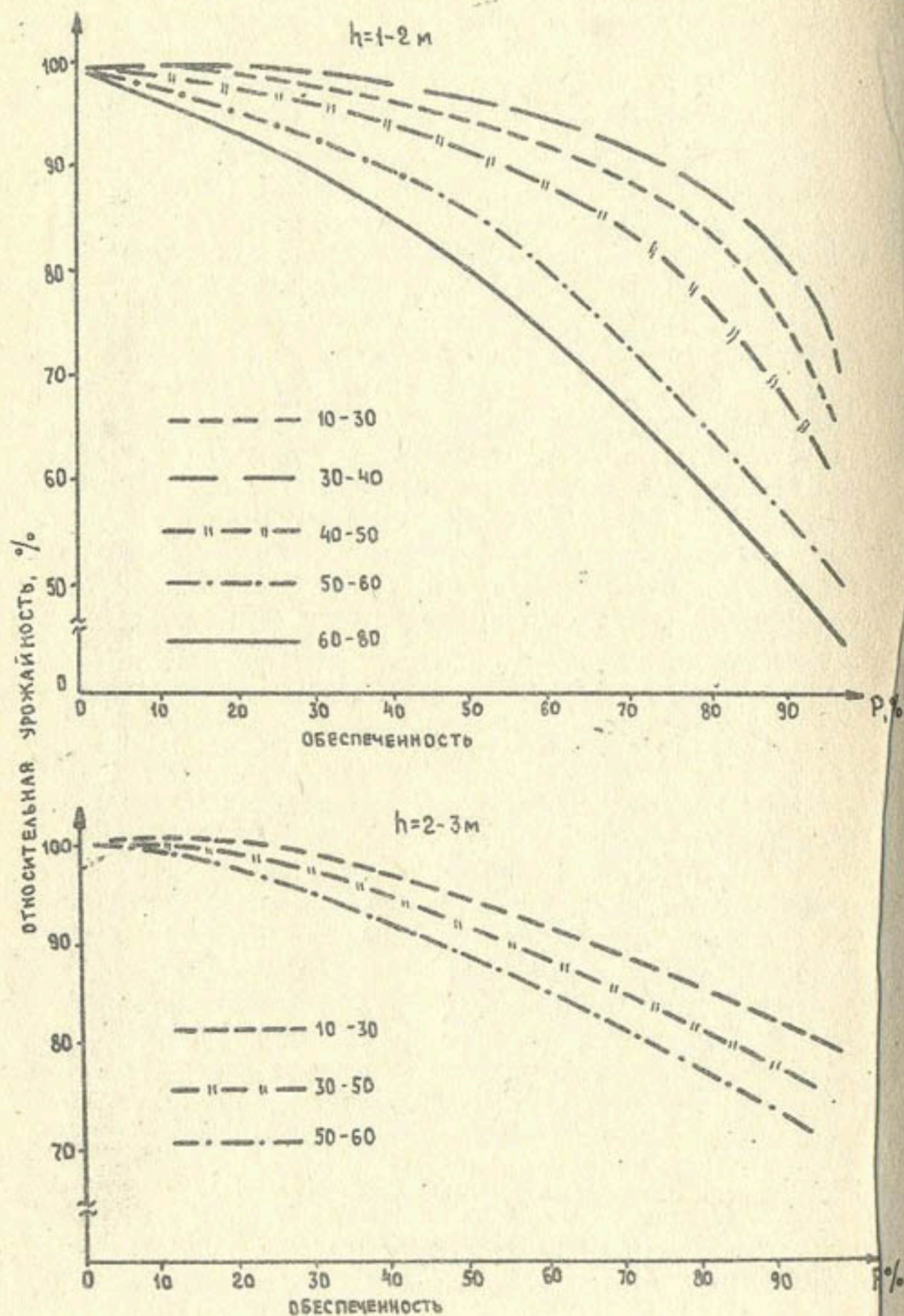
Рис. 5. Кривые обеспеченности относительной урожайности хлопчатника при разной доле участия грунтовых вод в водопотреблении.
