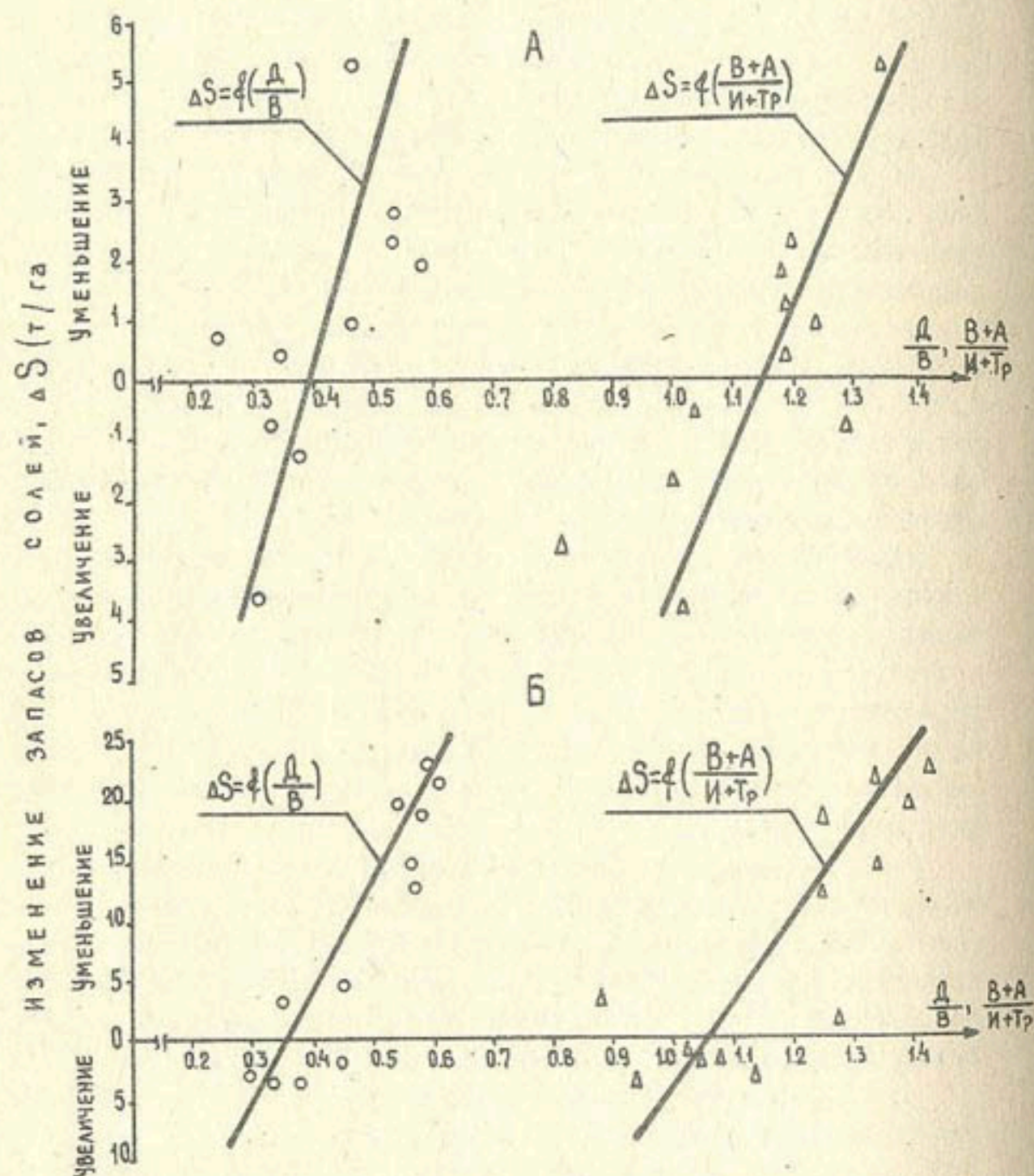
Рис. 3. Изменение запасов солей в расчетном балансовом слое от величины отношения дренажного стока к водоподаче ( A/B ) и водоподачи и атмосферных осадков к суммарному испарению ( \frac{B+A}{И+Тр} ) на опытных участках: А - на первом; Б - на втором (контрольном).
