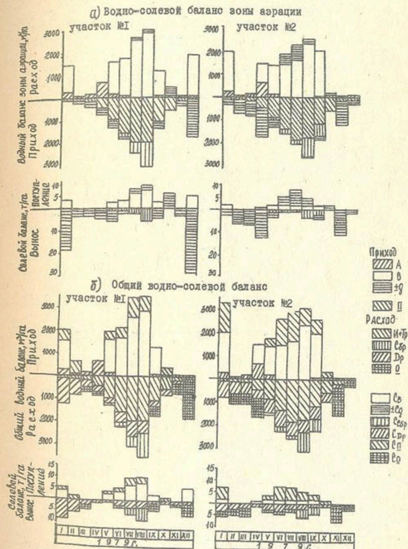
Рис. 4. Характерное внутригодовое распределение статей общих и частных водно-солевых балансов на ОПУ в Центральной Ферганае: А - атмосферные осадки; В - водоподача; ±q - водообмен между зоной аэрации и грунтовыми водами; П - приток подземных вод; Q - отток подземных вод; Спр - сброс с полей; Др - дренажный сток; (И+Тр) - суммарное испарение; Сл+Сд, Сср, Сл, Сдр, Со - поступления и вынос солей соответствующими элементами водных балансов.
