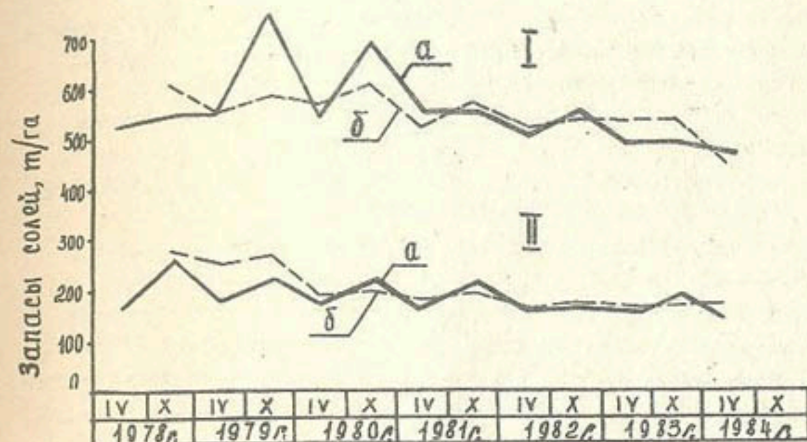
Рис. 7. Солевой режим почвогрунтов во внутригодовом разрезе: I — изменение запасов солей в 3-метровом слое; II — то же, в метровом слое; а — на участке № I (солевая точка № 2); б — на участке № 2 (солевая точка № 200)
