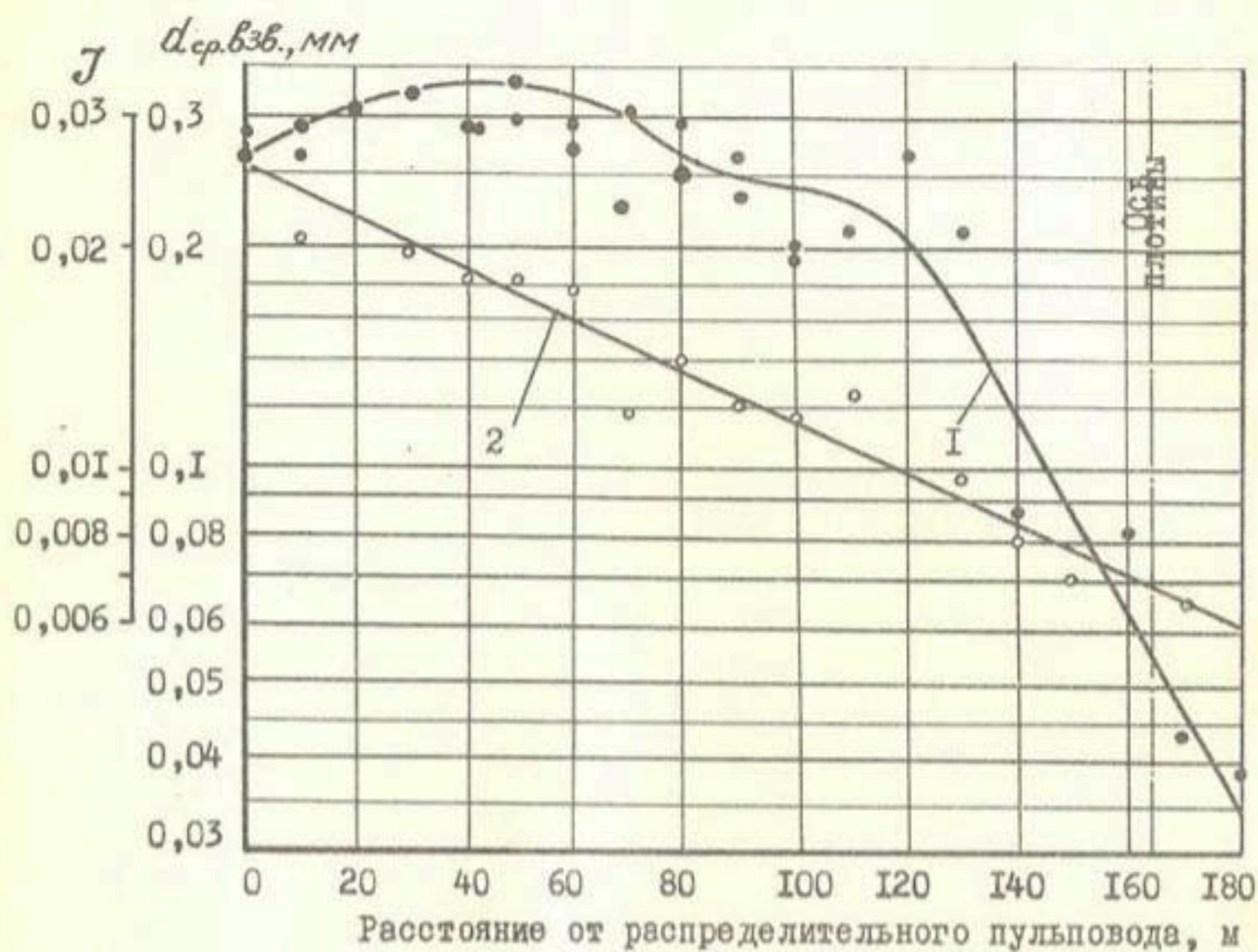
Рис. I Изменение средних уклонов поверхности карты и средневзвешенного диаметра частиц при рассредоточенном намыве из суглинка среднего, з/с 350- ЛК; I-уклон, 2-средневзвешенный диаметр частиц намываемого грунта
