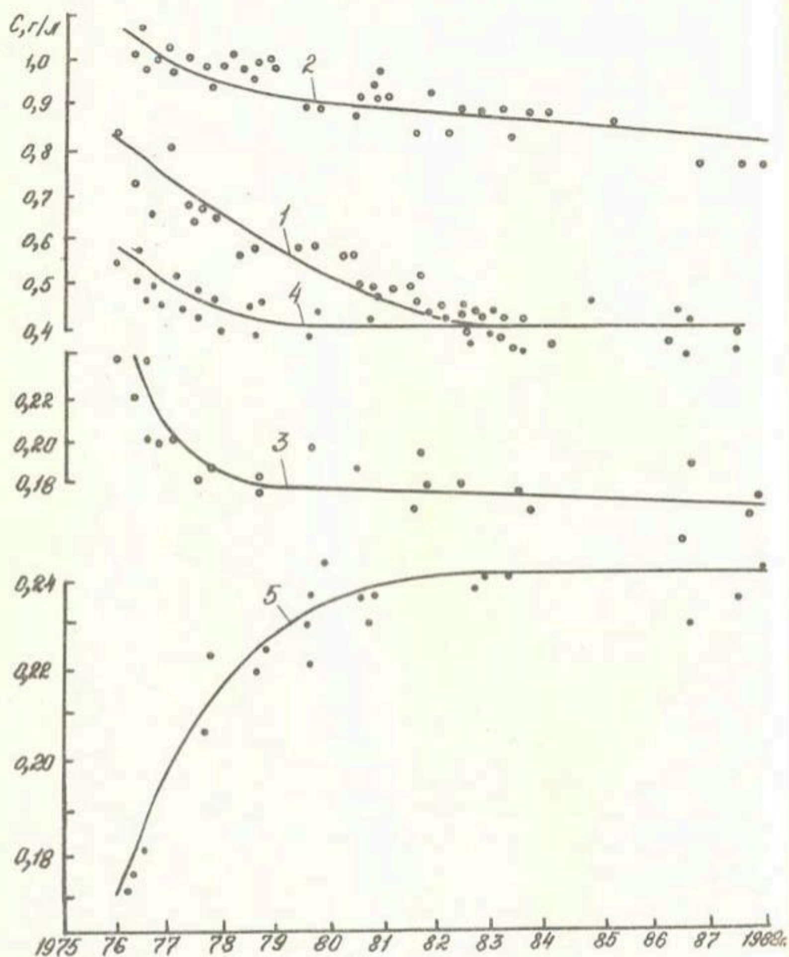
Рис. 1. Динамика содержания ионов \text{Cl}^- , \text{SO}_4^{2-} , \text{Ca}^{2+} , \text{Na}^+ , \text{HCO}_3^- в коллекторно-дренажных водах Главного Левобережного коллектора по данным режимных наблюдений, проводимых на Чарджоуской опытно-мелиоративной станции с 1976 по 1988 годы. 1- \text{Cl}^- . 2- \text{SO}_4^{2-} . 3- \text{Ca}^{2+} . 4- \text{Na}^+ . 5- \text{HCO}_3^- .
