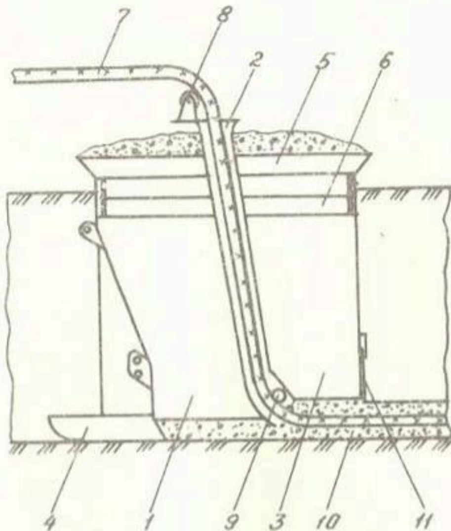
Рис.1. Конструктивная схема бункера-трубоукладчика для укладки длинномерных пластмассовых труб с круговой обсыпкой сыпучим фильтрующим материалом.
