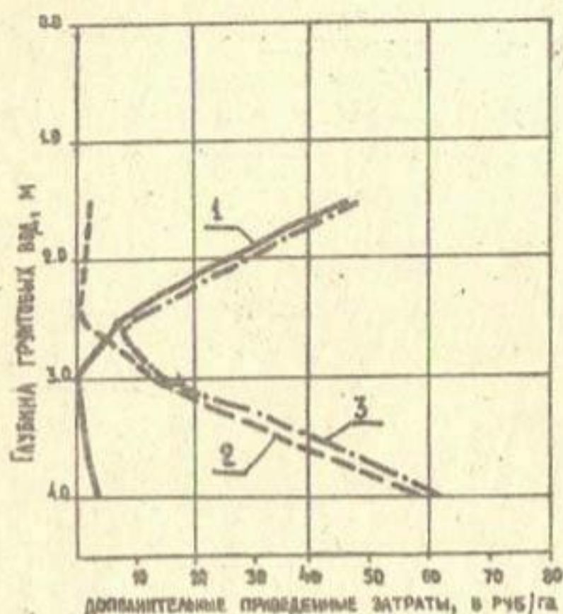
Рис.3. Зависимость приведенных затрат по дренажу и с/экономленной воде от глубины грунтовых вод: 1-приведенные затраты с/экономленной воды; 2-то же, по дренажу; 3-суммарные приведенные затраты по дренажу и с/экономленной воде.
