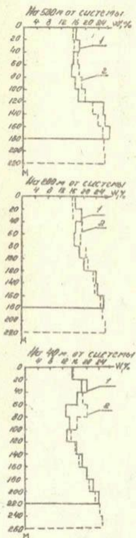
Рис. 3. Типовые эпюры влажности почвогрунтов на различном расстоянии от системы комбинированного дренажа на весенний (1) и осенний (2) периоды.
