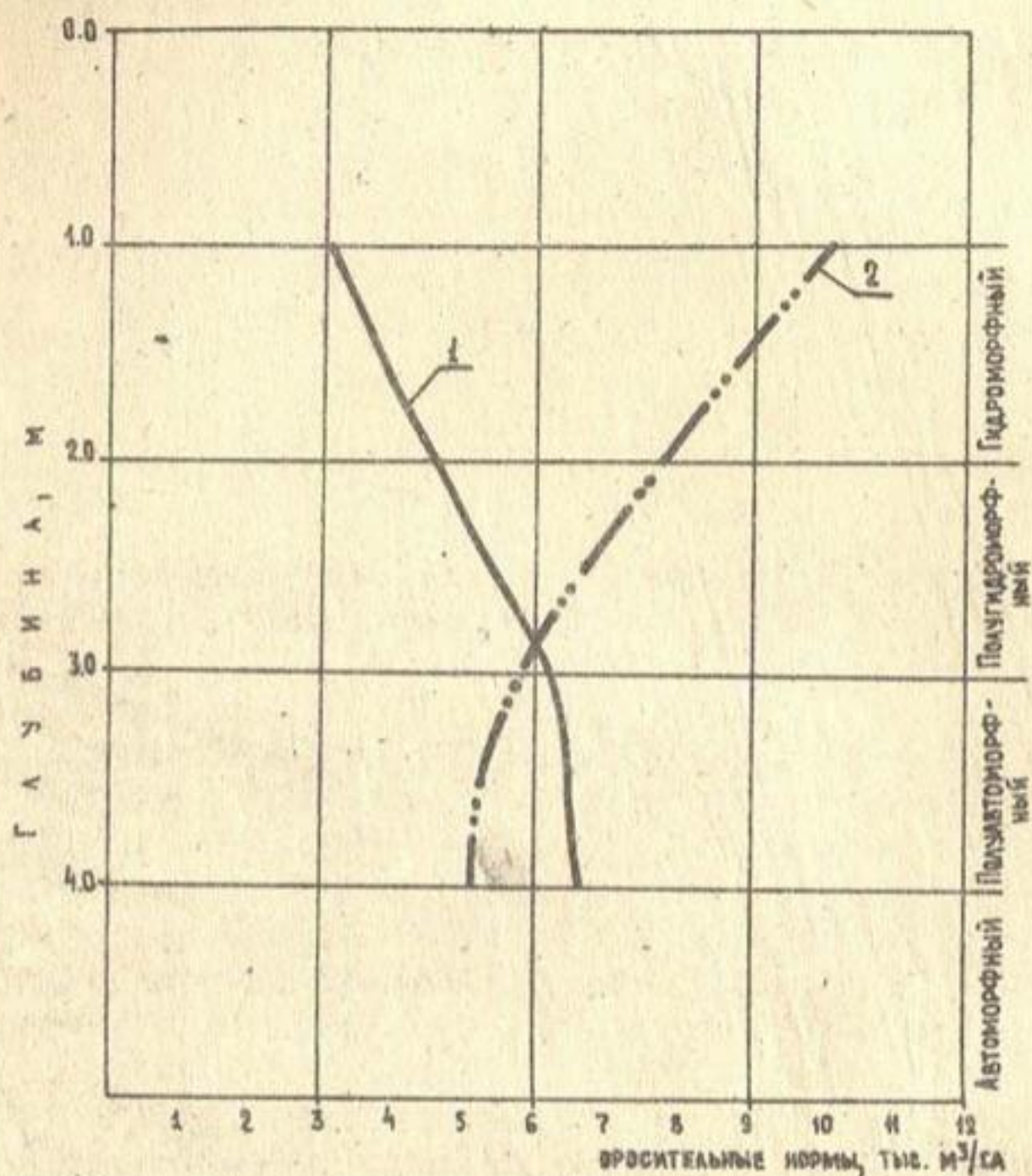
Рис. 1. Зависимость оросительной нормы от глубины залегания грунтовых вод и минерализация поливной воды: 1—оросительная норма с учетом питания из грунтовых вод за вегетационный период (полив пресной водой; по данным СоюзНИХИ); 2—водоподача за год с учетом поддержания солевого режима (полив пресной водой; величины расчетные).
