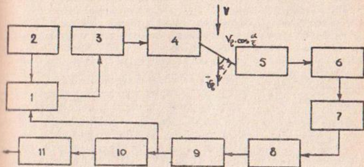
Рис.1. Структурная схема одного канала датчика: 1 — усилитель-манипулятор; 2 — генератор частоты; 3, 6 — согласующие каскады; 4 — вибратор-передатчик; 5 — вибратор-приемник; 7 — усилитель-ограничитель; 8, 9 — детектор и усилитель частоты; 10 — формирователь пилообразного напряжения; 11 — умножитель "x8".
