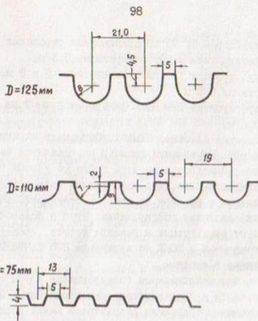
Рис. I. Профили гофров исследуемых труб диаметром 125; 110 и 75 мм
