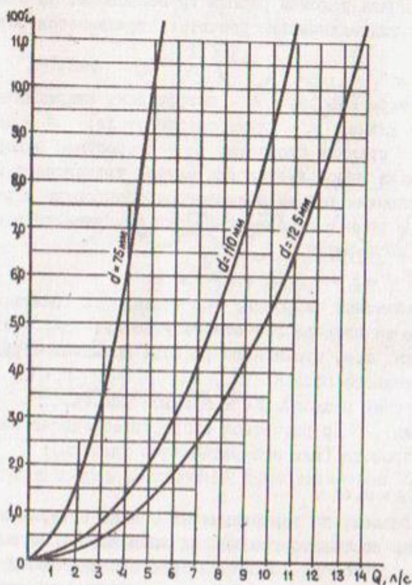
Рис.2. Зависимость Q = f(100h) для гофрированных пластмассовых труб диаметром 75; 110 и 125 мм
