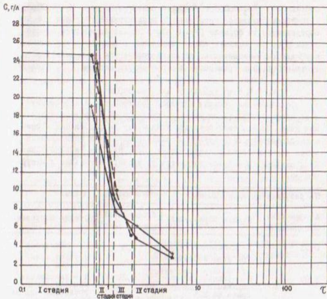
Рис.4. Сопоставление экспериментальных и натуральных данных об изменении минерализации в зависимости от коэффициента сменности поровых растворов: •—•—• скв. №15-1; ▲—▲—▲ опыт №3; + — + — + опыт №1
