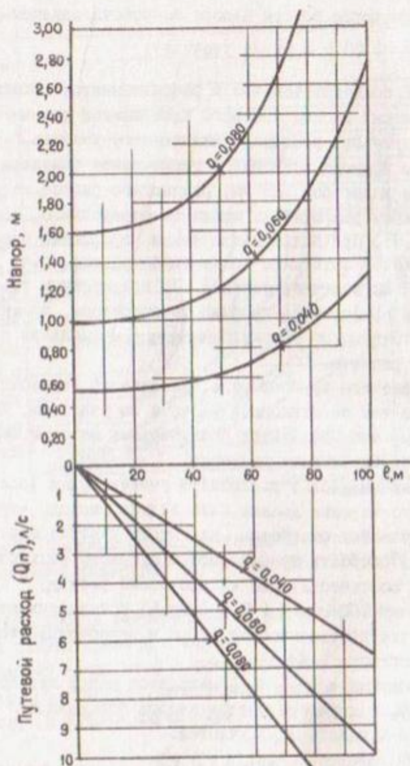
Рис. 7. Пример расчета трубопровода 125 мм, раздающего расход по длине из отверстий 5 мм
