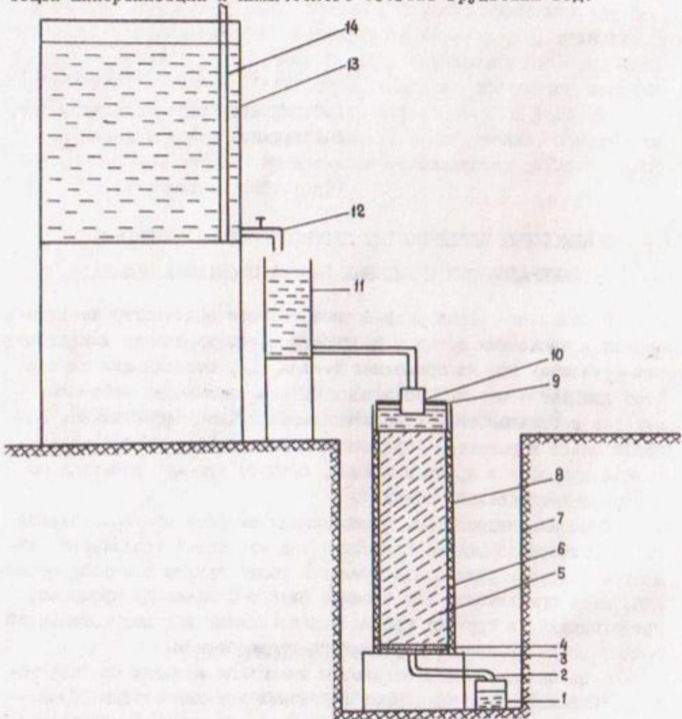
Рис. I. Инфильтрационная колонна: I - поддон; 2 - сливной шланг; 3 - песчаная обсыпка; 4 - галунная сетка; 5 - монолит; 6 - изоляция; 7 - траншея; 8 - корпус колонны; 9 - кольцо; 10 - поплавок; II - емкость для поддержания постоянного напора; 12 - кран; 13 - емкость для воды; 14 - рейка
