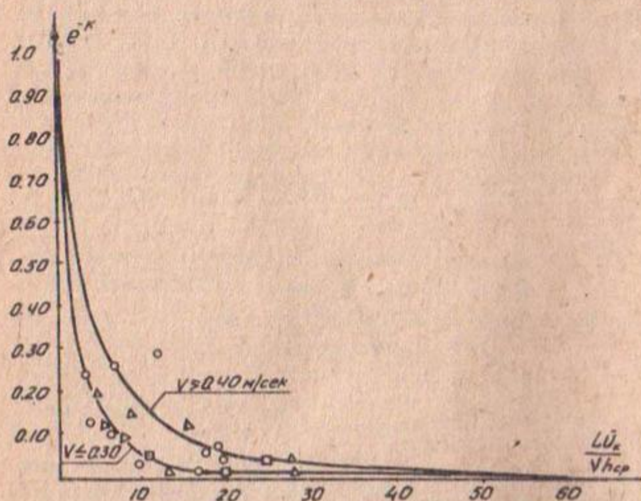
Рис.1. График зависимости e^k = f\left(\frac{L\bar{U}_x}{V_{нсп}}\right) (для фракции наносов 32-2мм/сек):
