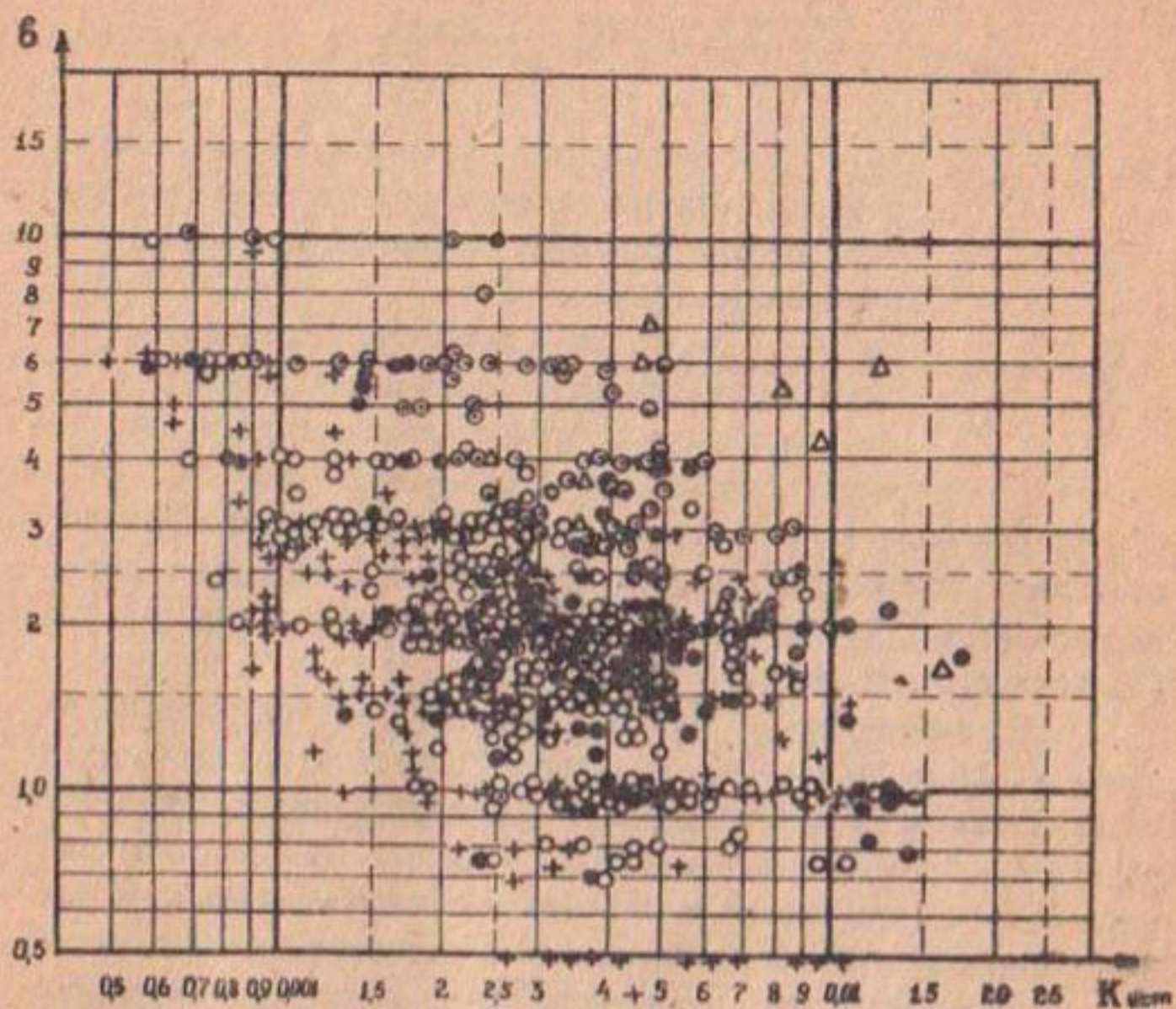
Рис. 2. Найденные из опытов x=f(t) параметры K_{вс} , \eta и \alpha к формуле впитывания
