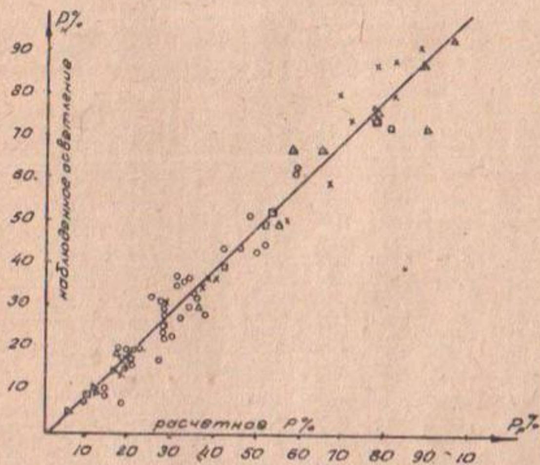
Рис.3. График сравнения освещения потока в отстойниках: о -отстойники Q < 10 м/сек; \Delta -отстойник Пахтаарна; □ -спрямление канала им.Ленина; * -отстойник Каракумского канала (по данным ВНИИГМ).
