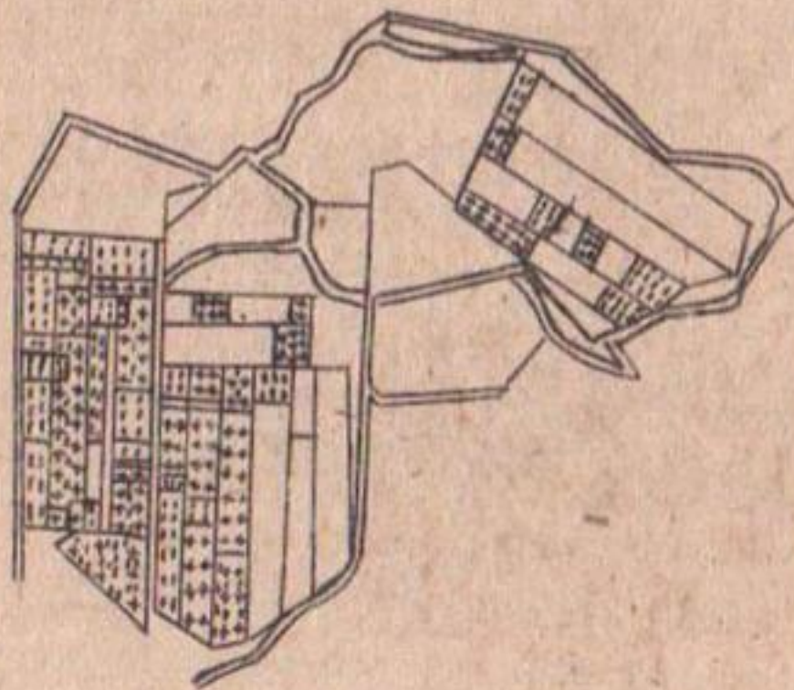
Рис. 1. Агрохимическая картограмма полей НИСТО по содержанию нитратного азота и гумуса в 1966 г. до дифференцированного распределения удобрений.
