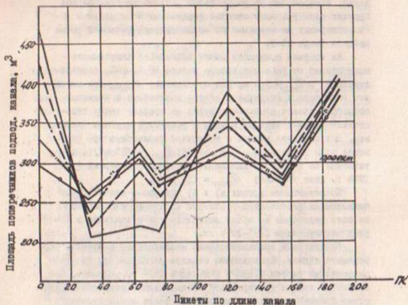
Рис. 2. Фактические площади поперечников подводящего канала НС-I ЮМК в фиксированных створах; динамика изменения поперечников в процессе эксплуатации в 1974 г.: март — — — — — ; апрель - - - - - ; май - — . — . — . ; июнь - — — — — ; июль - — — — — .
