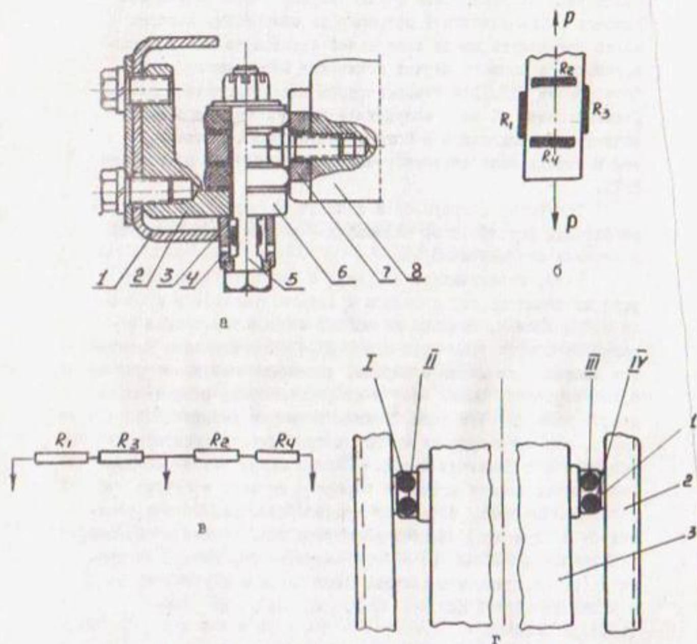
Тензоузел передней опоры двигателя: а) конструкция; б) схема наклеивания проволочных тензодатчиков; в) схема включения тензодатчиков в полумост; г) схема установки тензоузлов; I, II, III, IV - тензоузлы; 1 - кронштейн опоры; 2 - лонжерон; 3 - двигатель.
