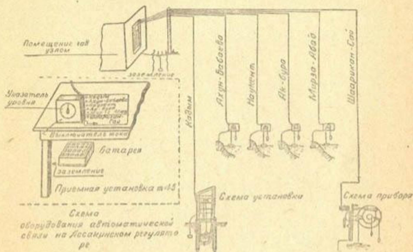
Рис. 13. Схема оборудования автоматической связи на Ассакинском регуляторе.
