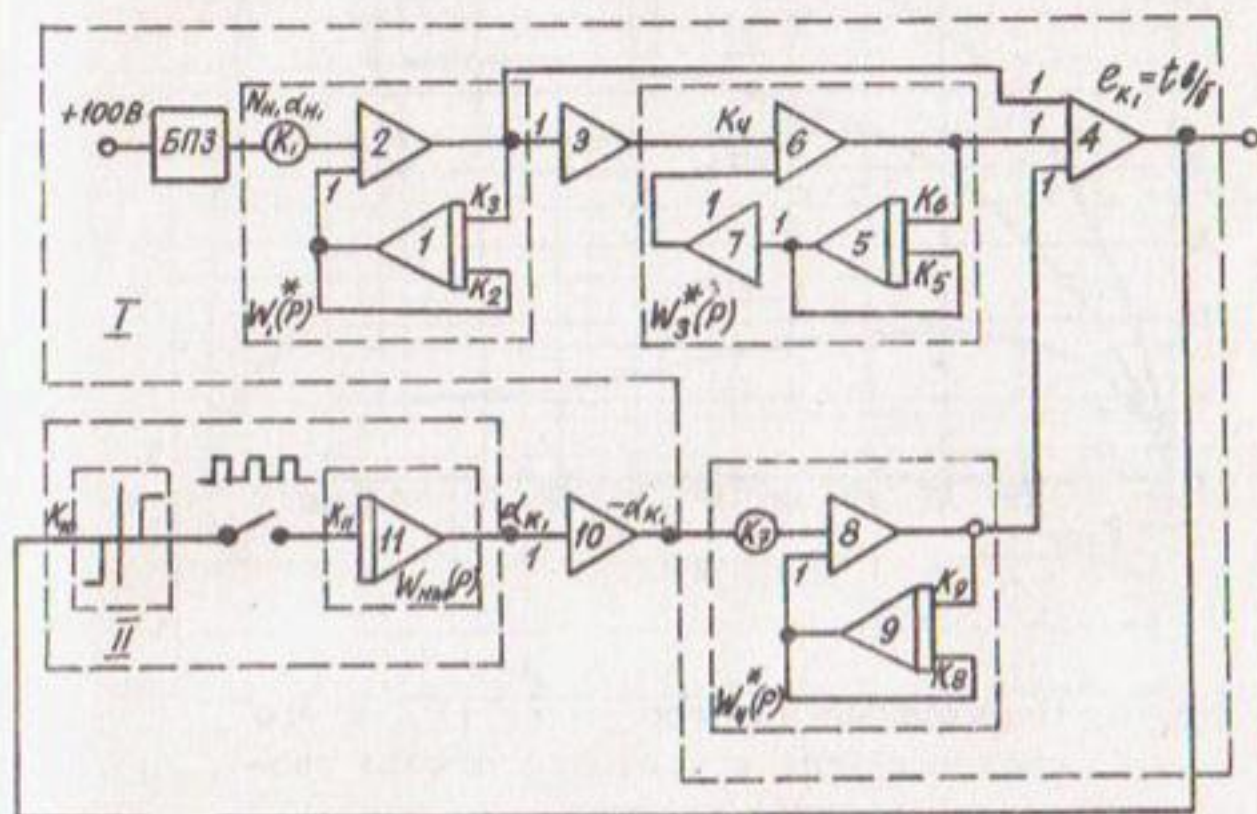
Рис. 3. Структурная схема модели САУ расчетного участка: 1 — модель объекта; П — модель авторегулятора.
