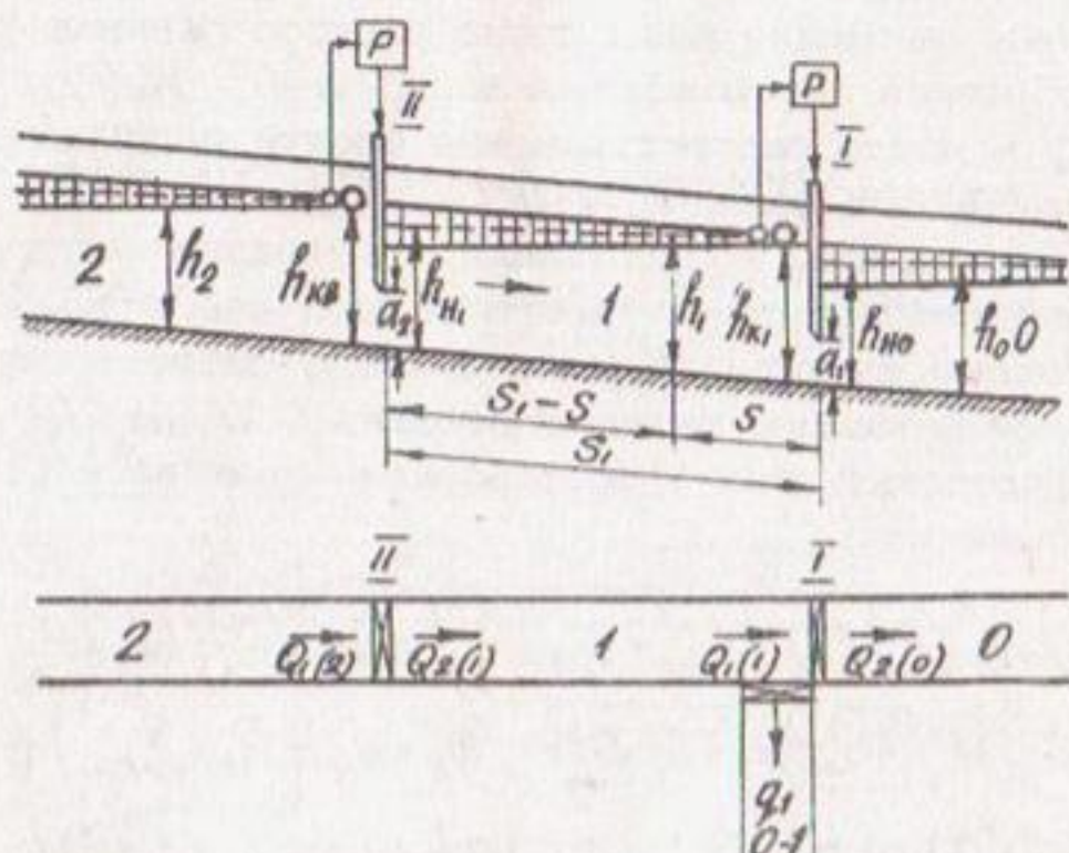
Рис. 1. Схема звена каскада при регулировании по верхнему бьефу.
