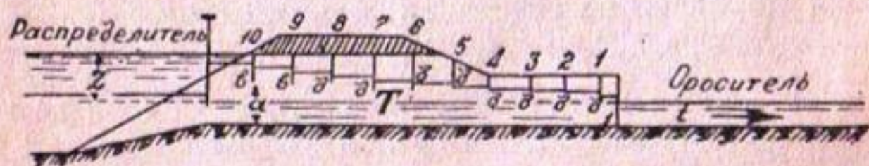
Рис. 40. Диафрагмовый автомат Журина.
