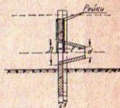
Рис. 52. Типовой чертеж колхозного водомера-насадка.
