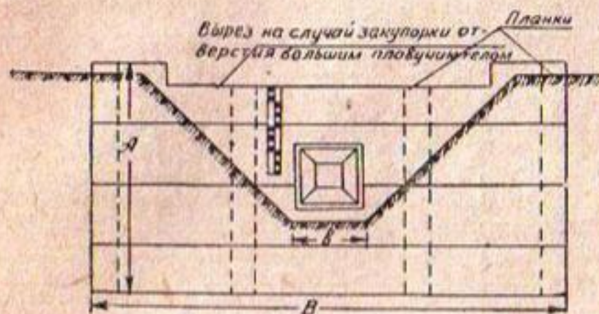
Рис. 52. Типовой чертеж колхозного водомера-насадка.
