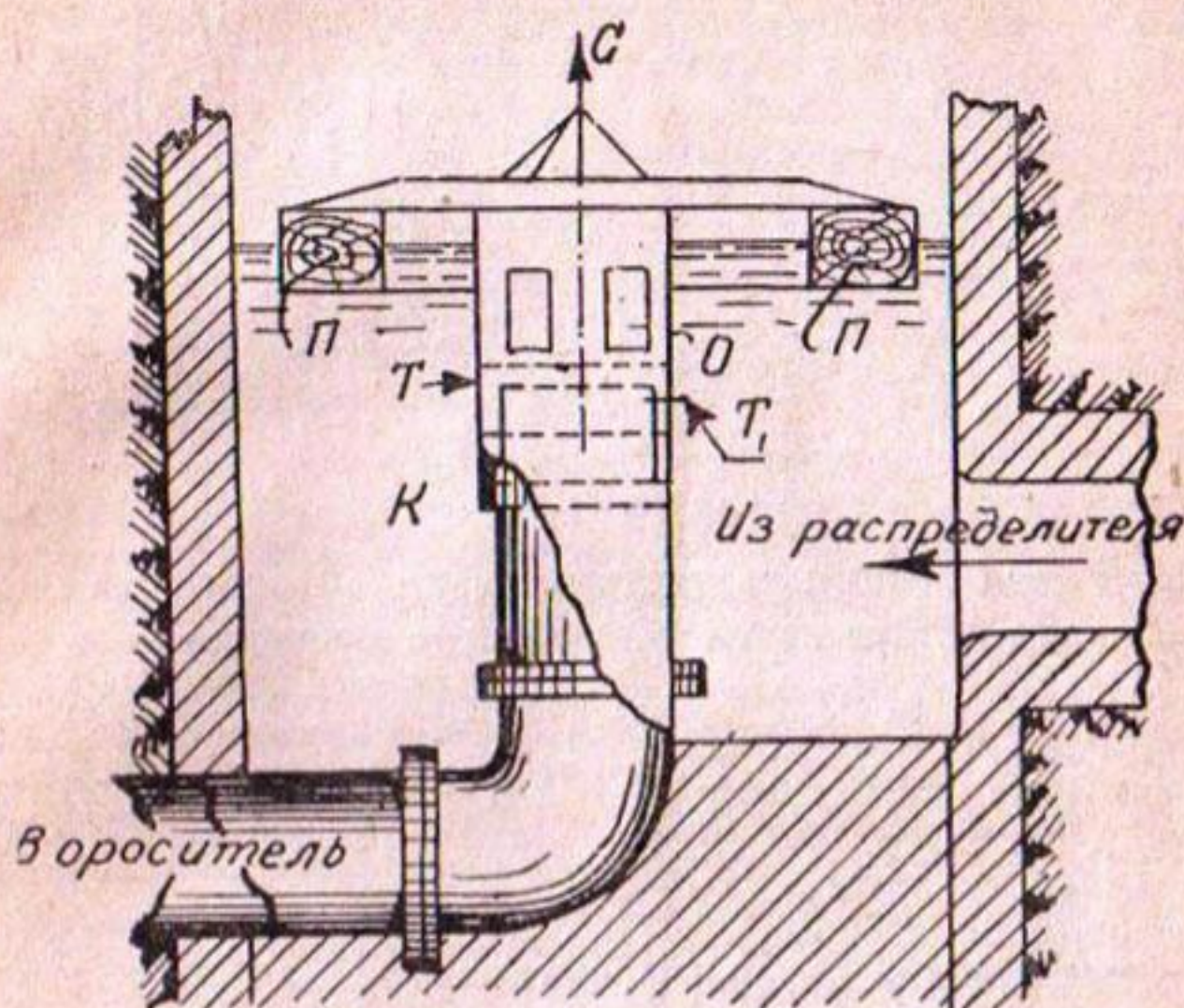
Рис. 33. Автомат Линдлея.
