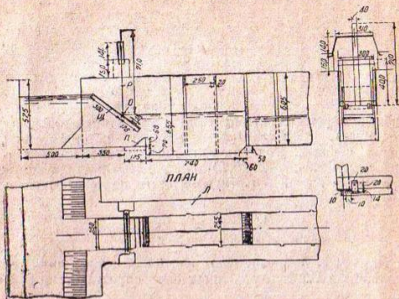
Рис. 61. Исполнительный чертеж модели водомера-автомата.
