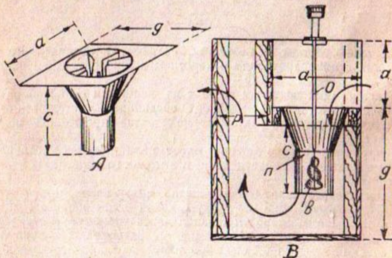
Рис. 8. Водомер Рилайнса. Установка в деревянном ящике.
