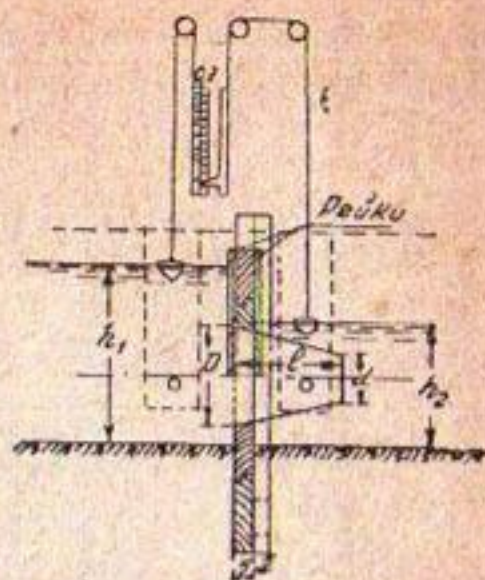
Рис. 51. Типовой чертеж колхозного водомера-насадка со схемой указателя.
