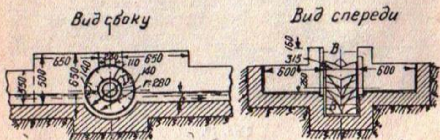
Рис. 21. Водомер Барановского.
