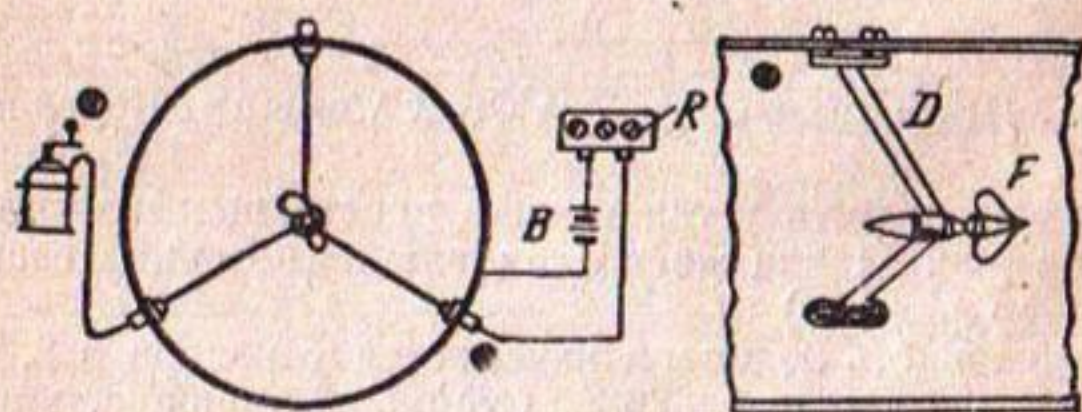
Рис. 13. Установка непрерывно действующей вертушки Отта в круглой трубе.
