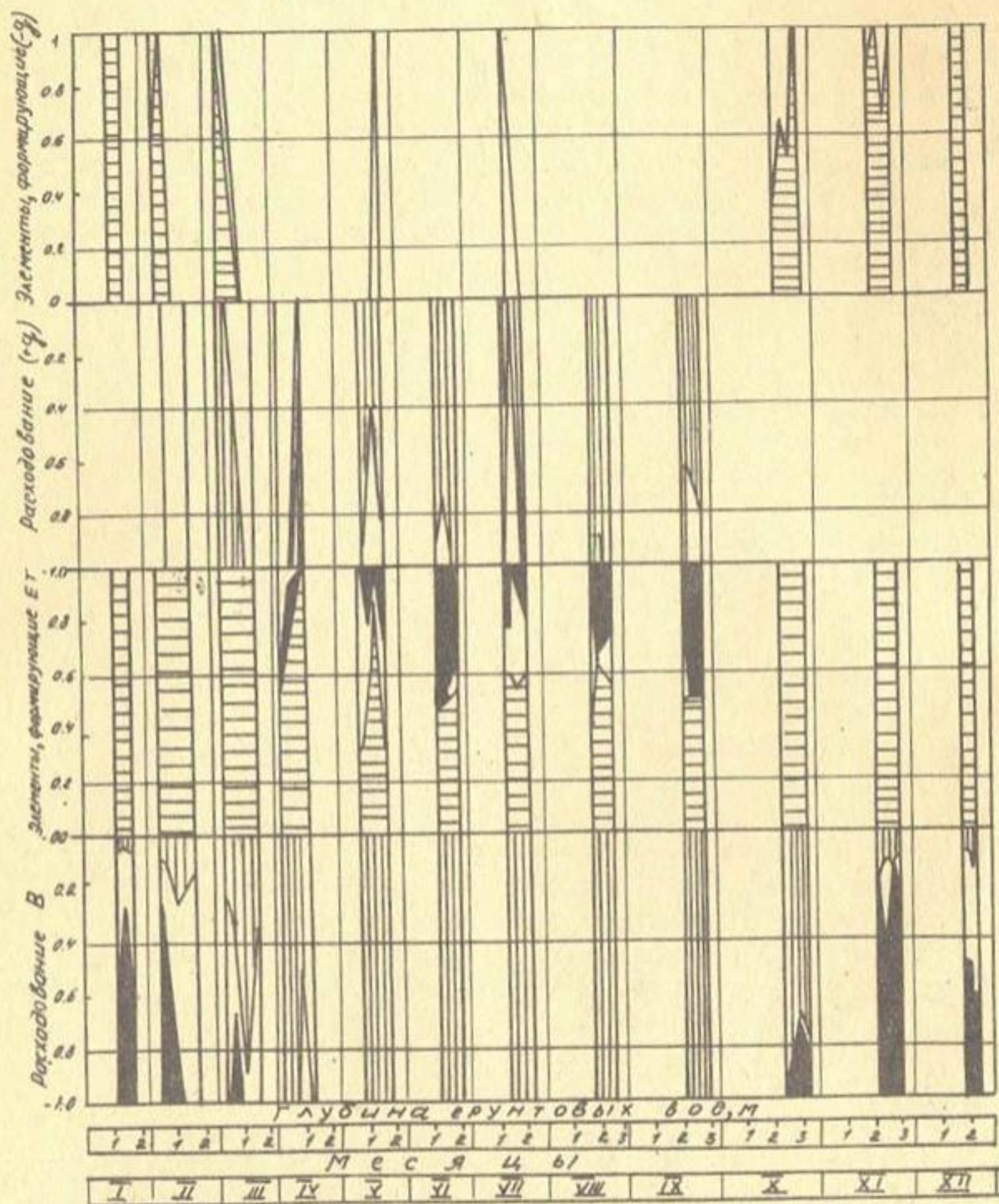
Рис. 3. Количественный характер формирования и расхода основных составляющих водного баланса зоны эврации при гидрометеорологическом режиме (ОПС в с-зе Поктаарал в бездренажных условиях)
