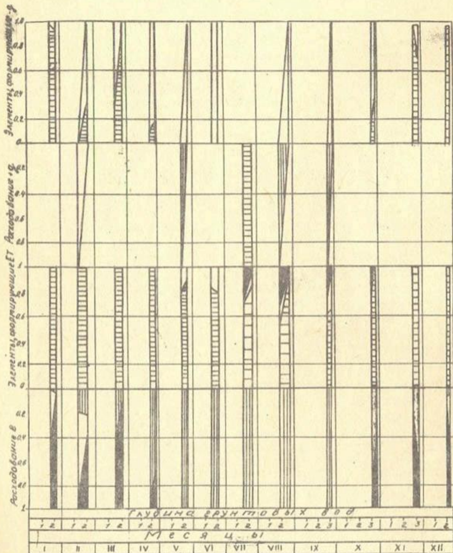
Рис. 4 Количественный характер формирования и расхода основных составляющих водного баланса зоны эвации при полувлажном мелкоморфном режиме (опс в с-зе Пахтаарал после ввода в эксплуатацию вертикального дренажа).
