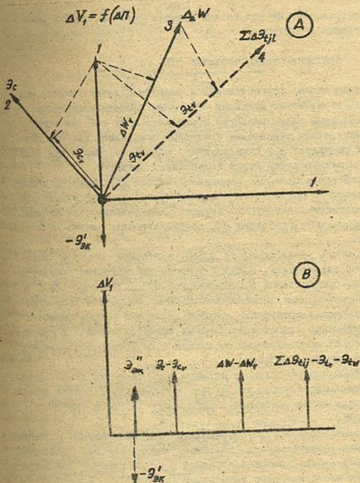
Рис. 18. ПРИМЕНЕНИЕ ВЕКТОРНОГО МЕТОДА ОЦЕНКИ ЭФФЕКТИВНОСТИ ПО Р.И. ШИЛПЕРУ А - оцениваемый вариант; В - сумма альтернативных вариантов
