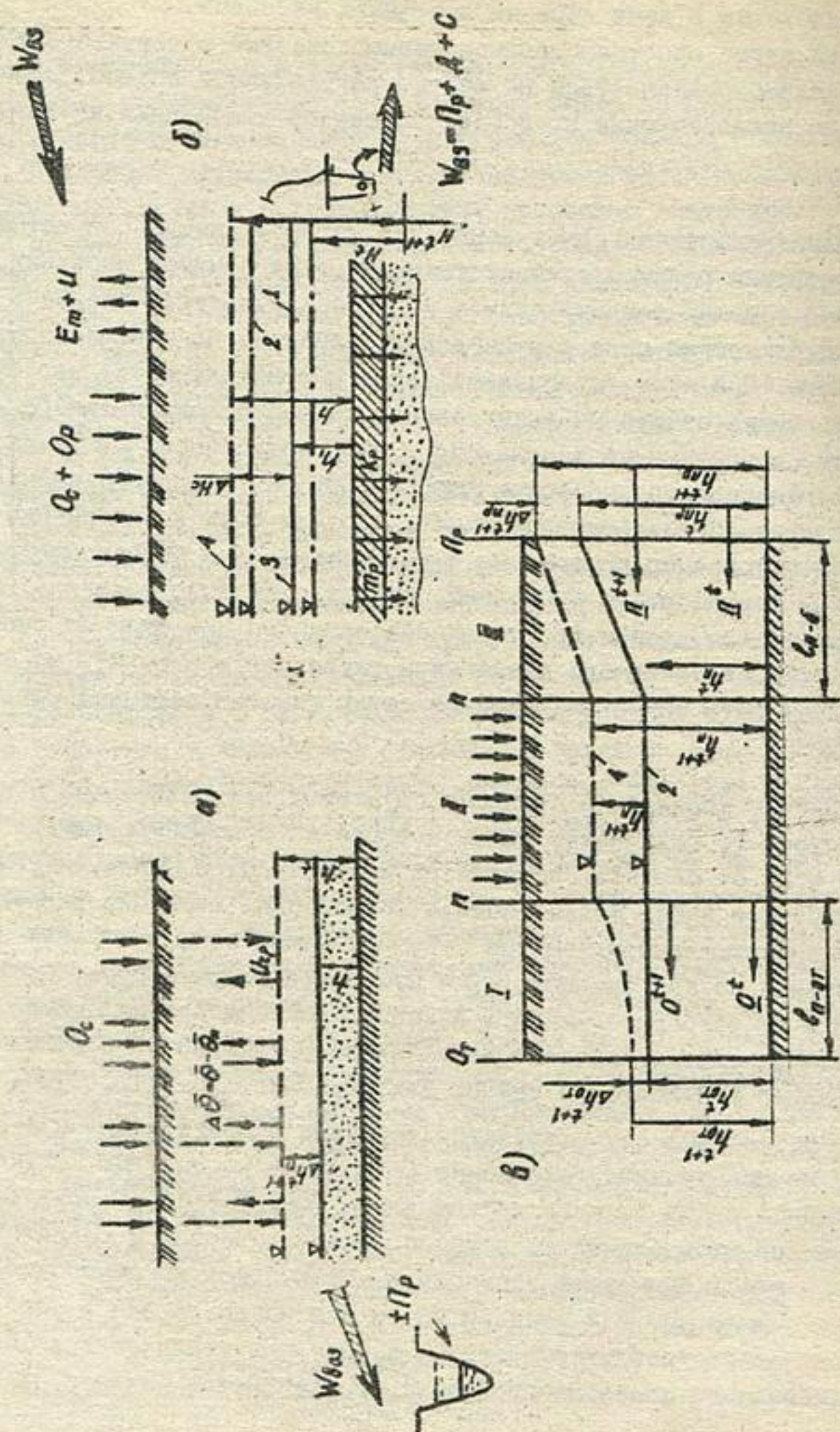
Рис. 9. Схемы взаимодействия вод: а) до орошения; б) при орошении; I - УТВ до орошения; 2 - УТВ при орошении; 3 - линия пьезометрического напора до орошения; 4 - то же при орошении
