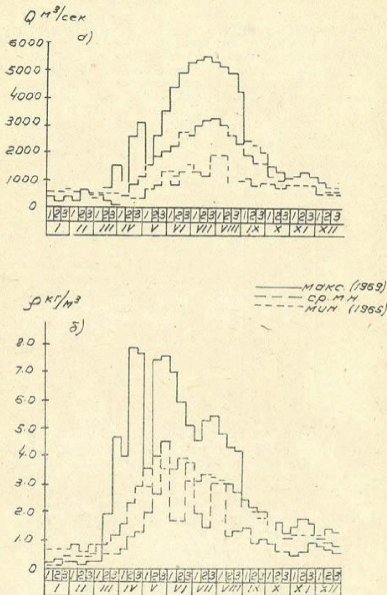
Рис. 5. Гидрографы средних декадных расходов (а) и мутности воды (б) по створу Чатлы.
