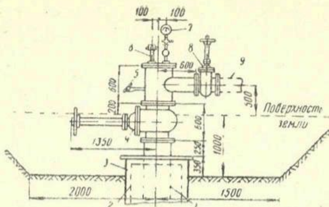
Рис. 9. Схема оборудования устья скважины с самоизливом из них:
