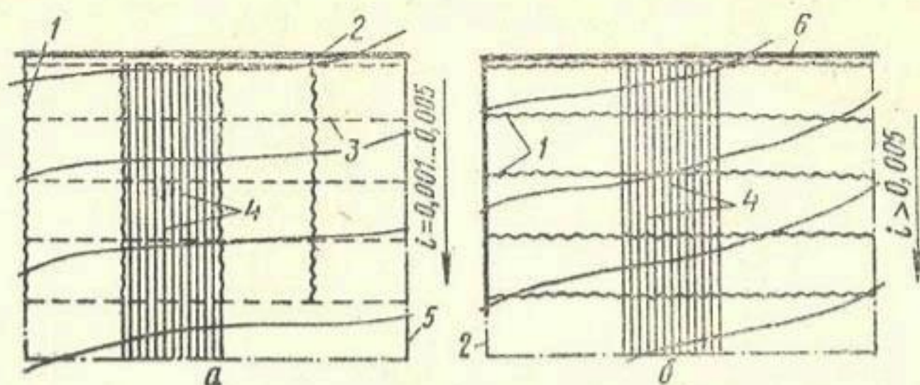
Рис. 2. Схемы расположения временной оросительной сети: а, б — продольная и поперечная схемы; 1 — временный ороситель; 2 — участковый распределитель; 3 — выводные борозды; 4 — поливные полосы или борозды; 5 — граница поливного участка; 6 — распределитель.
