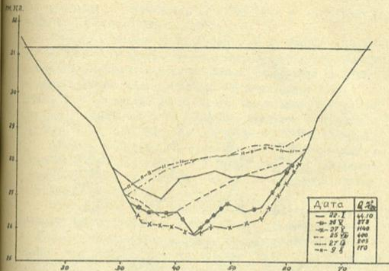
Рис.1. Совмещенные поперечные профили р.Чирчик (г/п Ходжикент, 1969г.)
