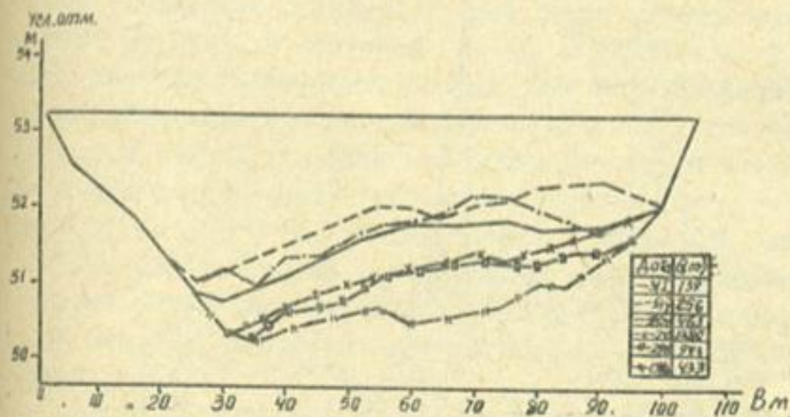
Рис.2. Совмещенные поперечные профили р.Нарин (г/п Учкуртан, 1941г.)
