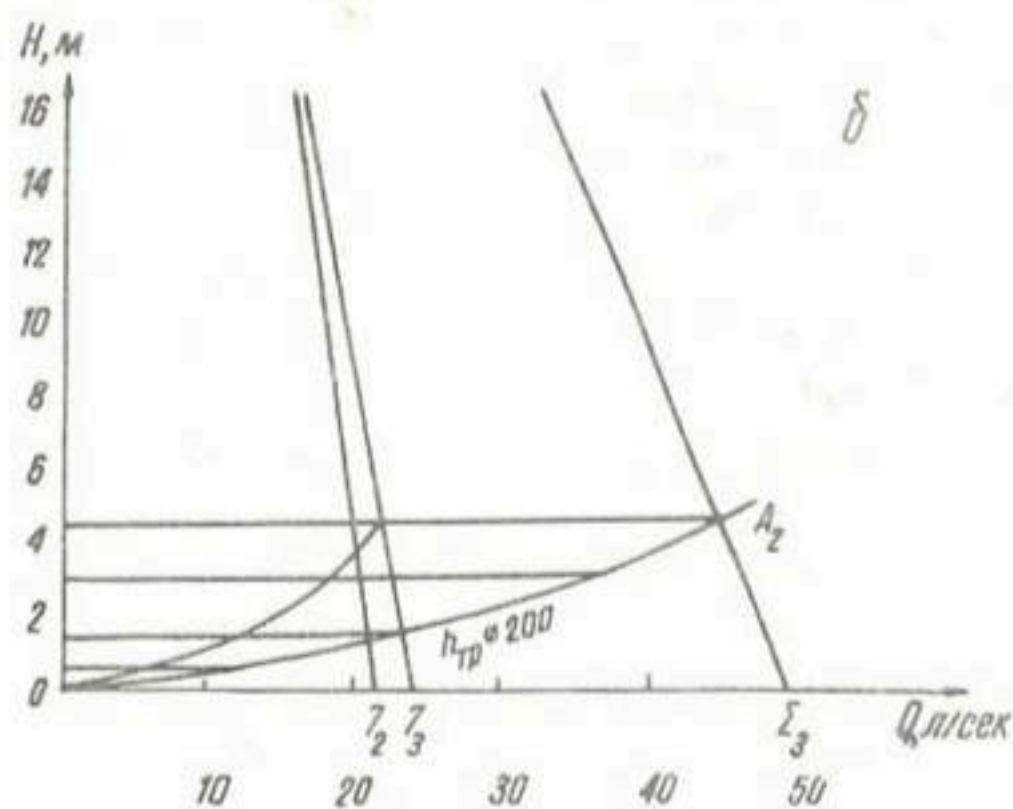
Рис. 3. Совместная работа группы скважин на общую магистраль (а) и распределение потерь напора (б).
