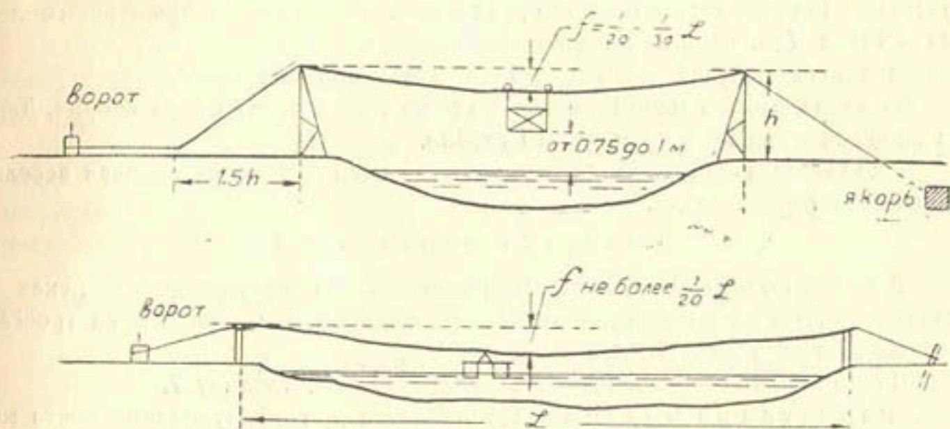
Рис. 6. Схема люлечной установки и паромного створа
