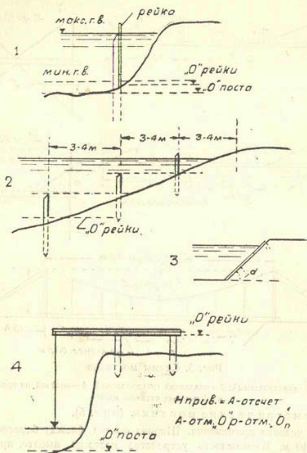
Рис. 4. Водомерные рейки
