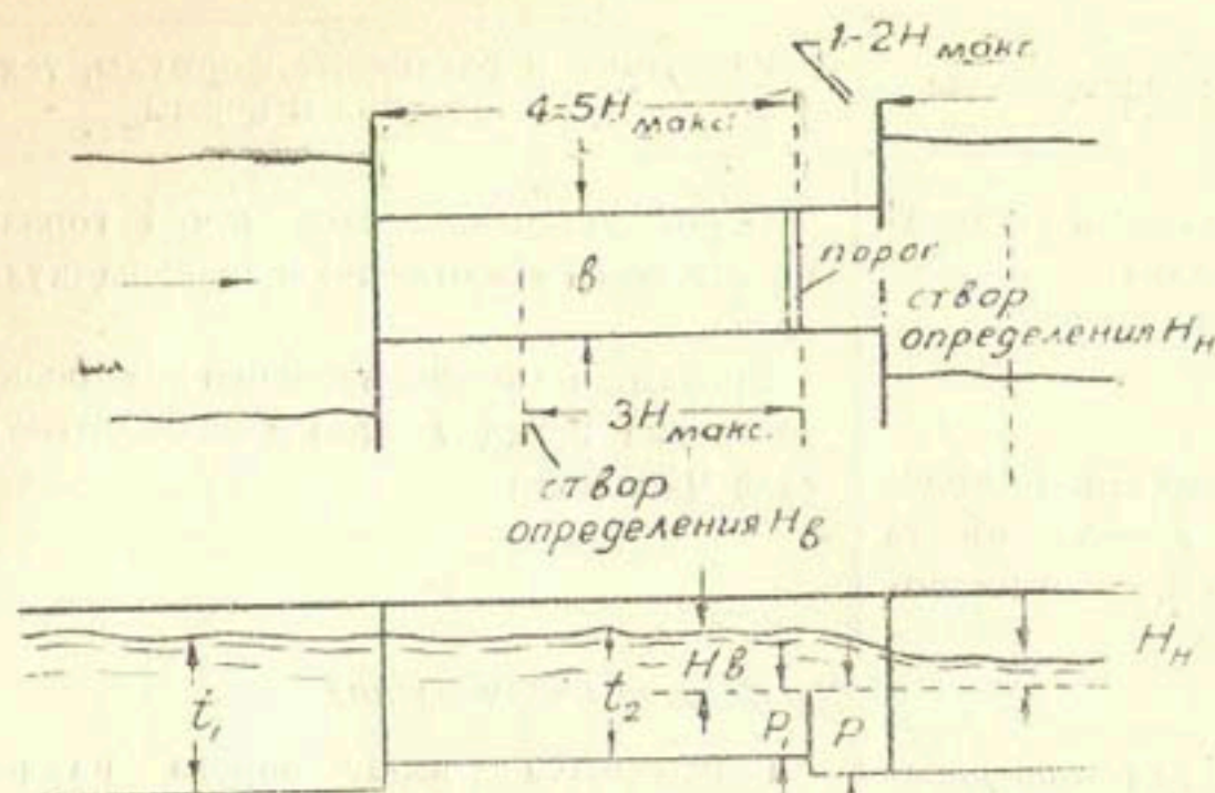
Рис. 10. Водослив Базена
