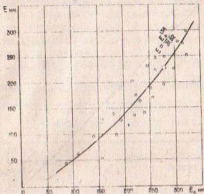
Рис.2. Связь суммарного испарения хлопковым полем с испаряемостью (III гидромультильный район):
