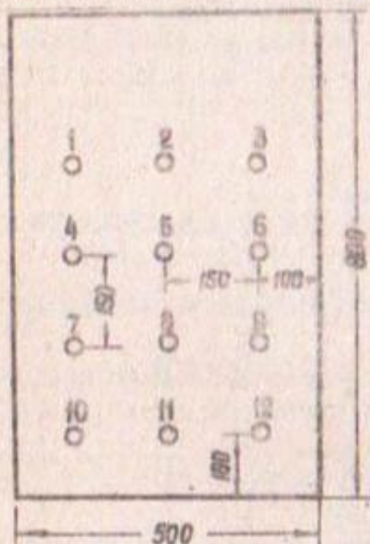
Рис.3. Боковая стенка лотка с указанием расположением пьезометров (размеры в мм).
