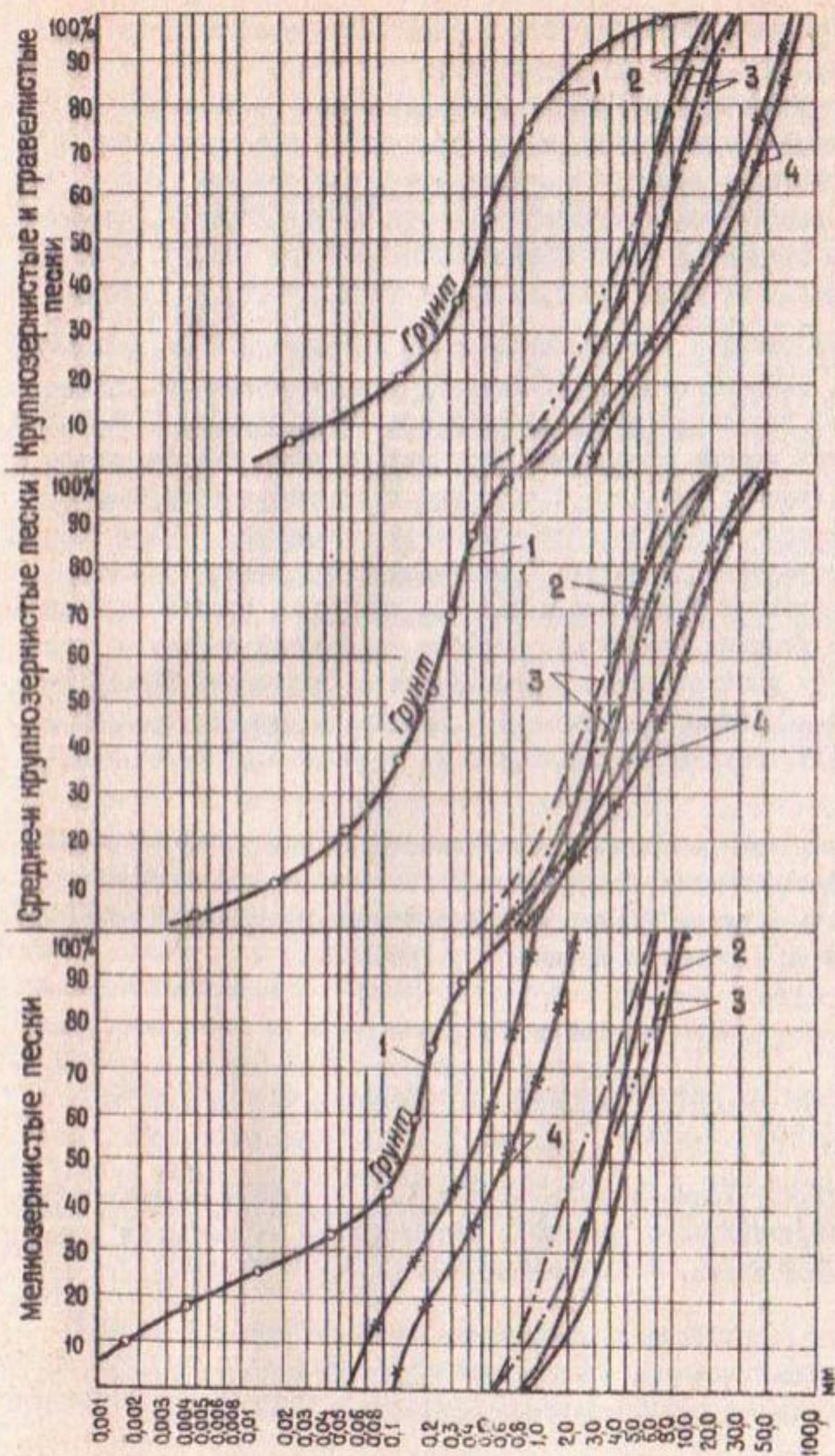
Рис. 2. Варианты фракционного состава сильных обсыпов для скважин вертикального дренажа ( \lambda — о — о фракционный состав грунтов; расчетная область обсыпок: 2 — — — по рекомендациям Снеда; 3 — — — по рекомендациям Санитарии; 4 — — — по рекомендациям Виггема).
