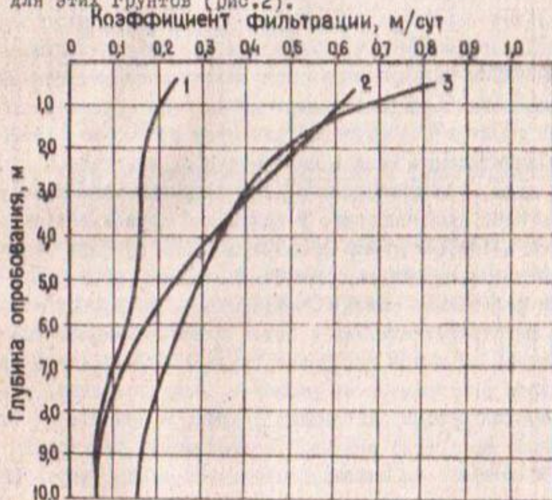
Рис. 2. Зависимость коэффициента фильтрации от глубины опробования грунтов для крупных логов (1), склонов крупных логов (2) и водоразделов (3).
