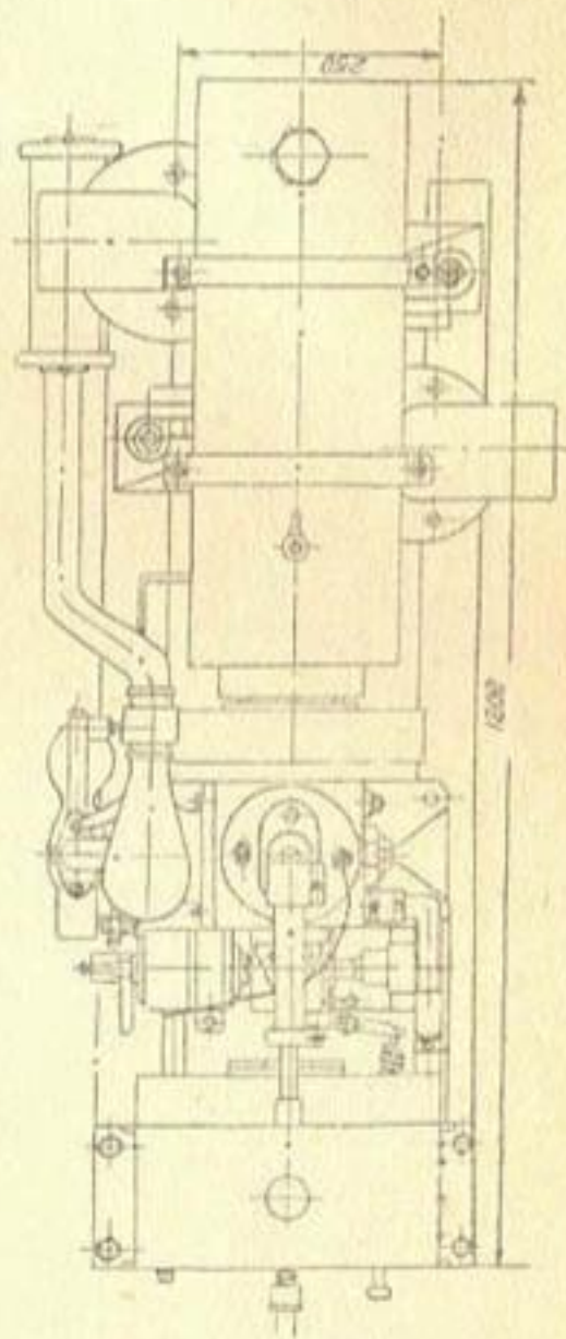
Рис. 44. Передвижной всасывающий эрлифт сист. Алексеева.
