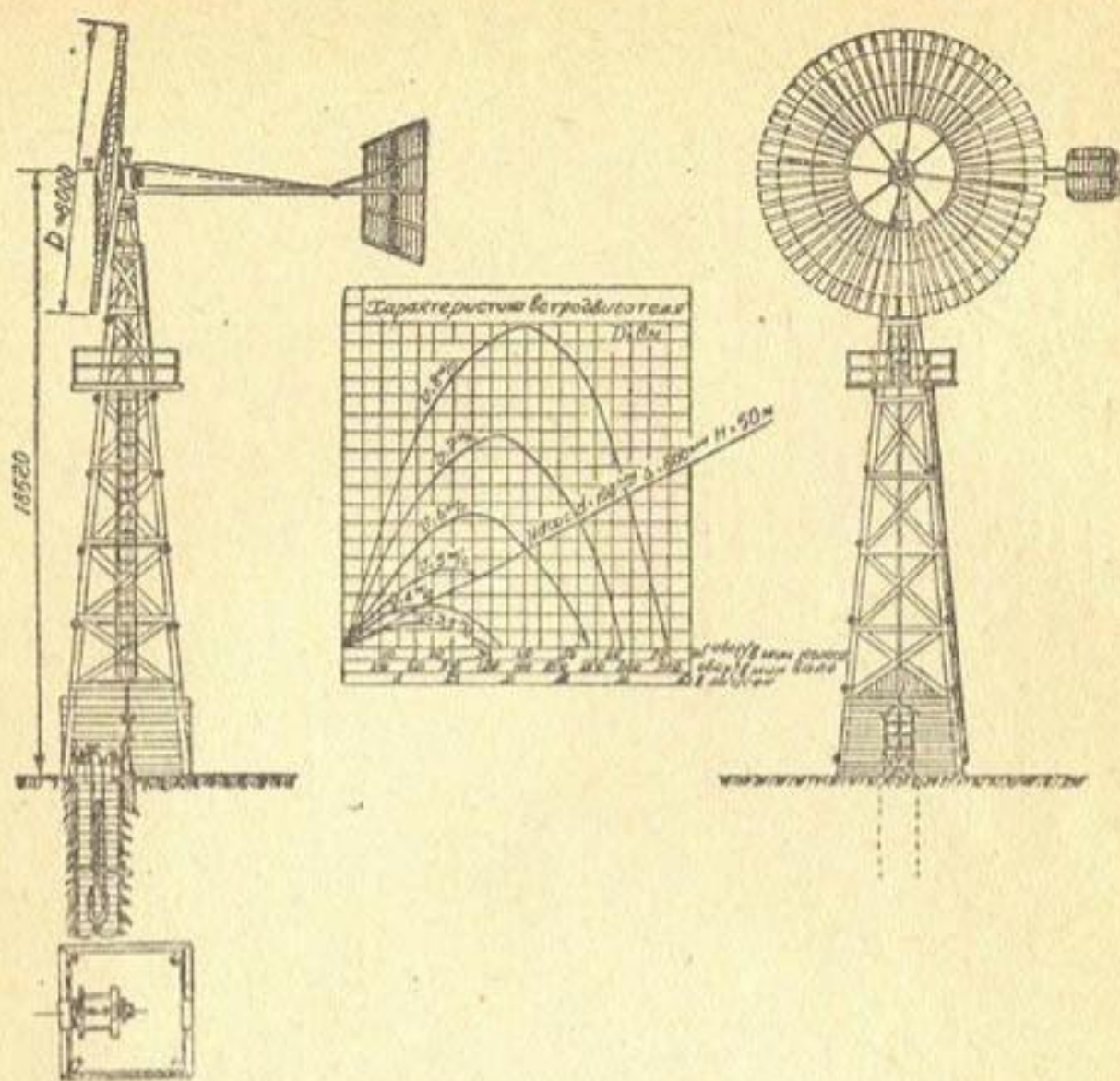
Рис. 8. Ветровая водоподъемная установка со сдвоенным поршневым насосом.
