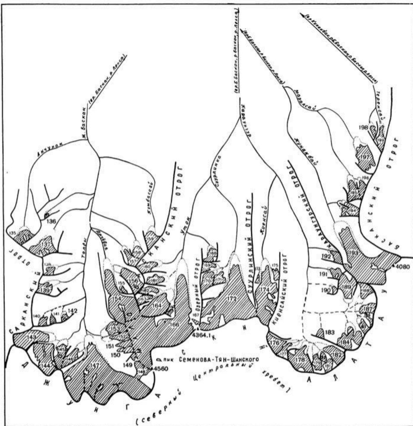
Рис. 21. Схема расположения ледников в бассейне р. Баскан. Усл. обозначения см. на рис. 17.
