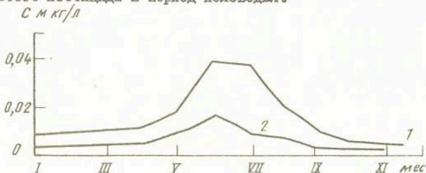
Динамика концентраций \alpha -ГХЦГ в воде рек Кызылча (1) и Бошкызылсай (2)
