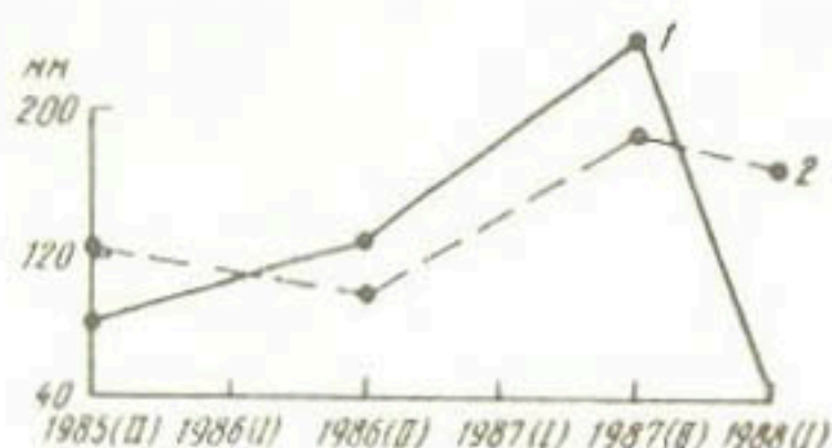
Рис. 1. Выпадение осадков в 1985-1988 гг. в Алтыарыкском районе Ферганской области (1) и Термезском районе Сурхандарьинской области (2). Римские цифры - полугодия
