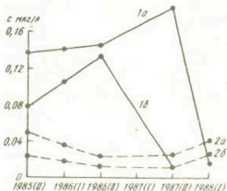
Рис. 2. Содержание \alpha - (а) и \gamma - ГХП (б) в Северобагдадском коллекторе п. Алтыарык (1) и р. Амударье г. Термез (2): I - весна, 2 - осень
