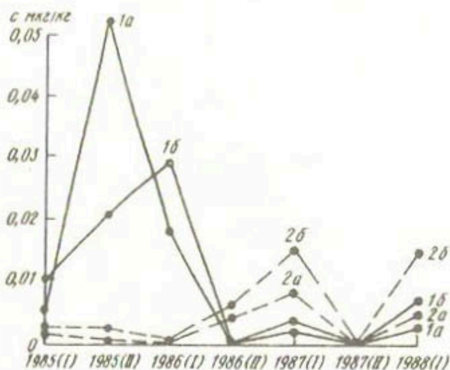
Рис. 3. Содержание \alpha - (а) и \gamma - ГХП (б) в почве Алтыарыкского (1) и Термезского (2) районов: I - весна, II - осень
