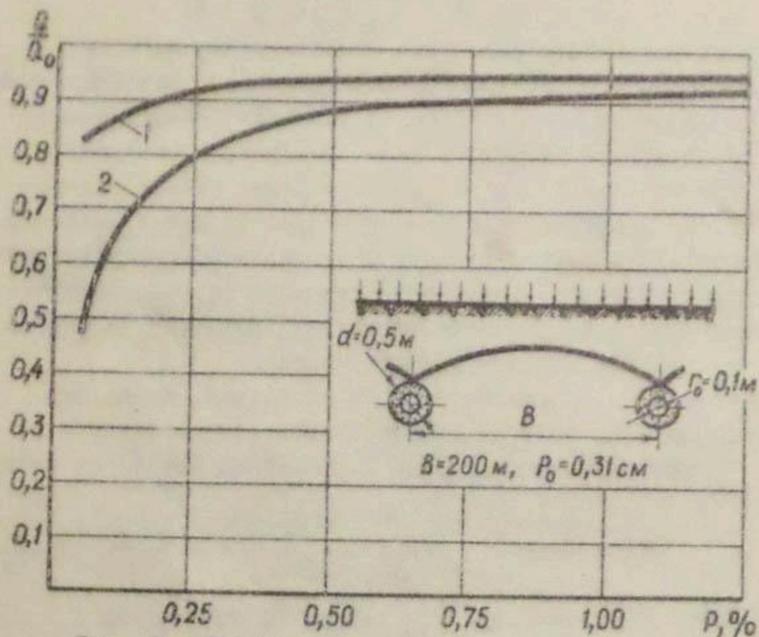
Рис. 3. Графики относительного расхода: 1- с учетом фильтрационных деформаций, 2- без учета фильтрационных деформаций.
