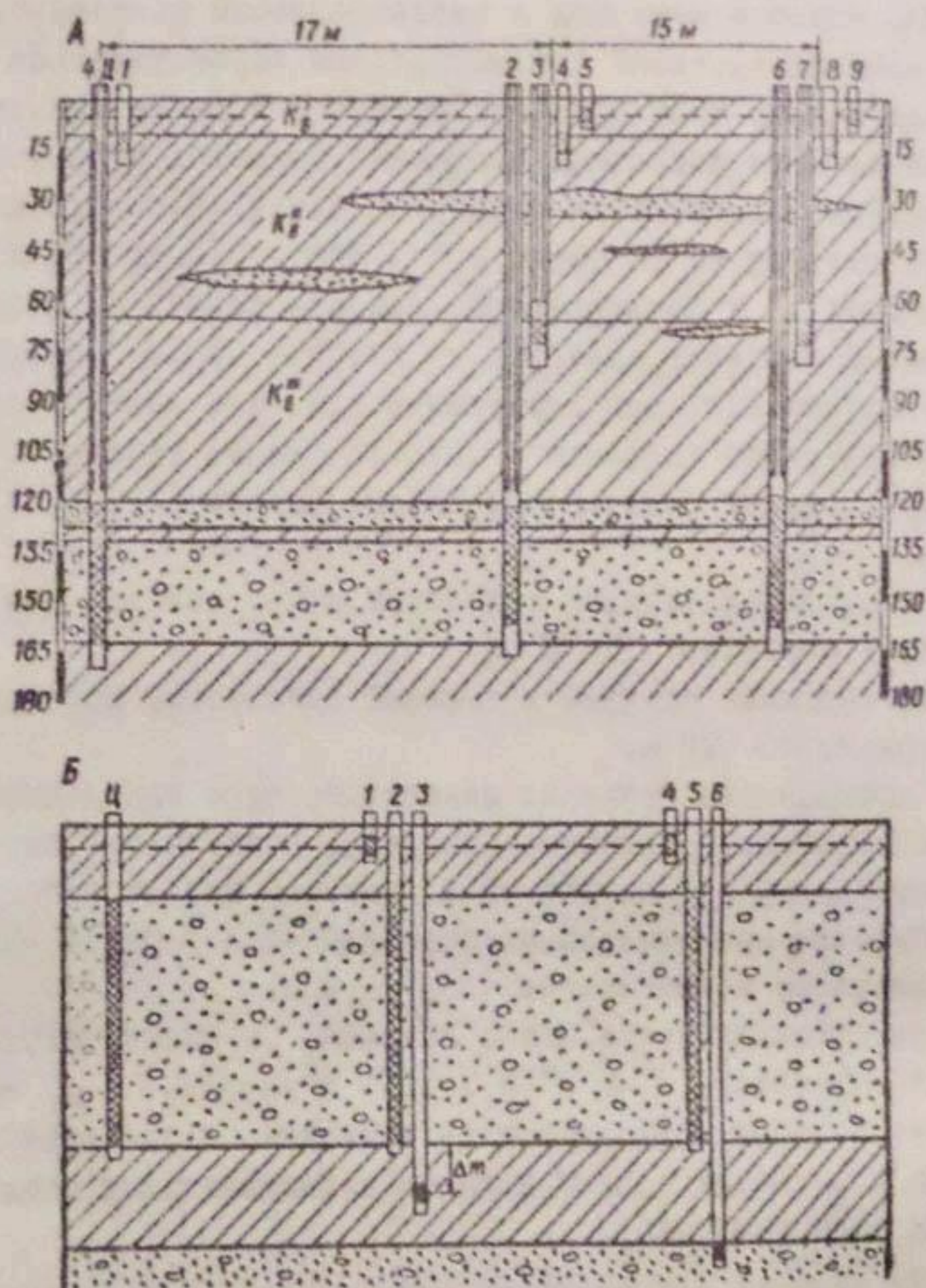
Рис. 4. А- схема опытного куста № 4 в Кокаральской степи, Б- принципиаль- ная схема опытного куста в двухплас- товой системе с маломощным покровным слоем.
