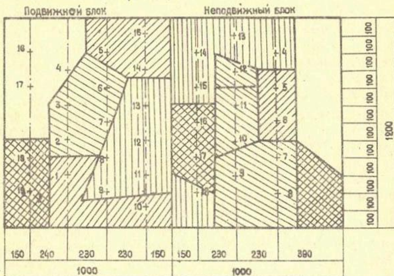
Рис. 5. Схема разрушения контакта "металл шпонки-бетон" при поэтапном перемещении подвижного блока (для фрагмента А):
