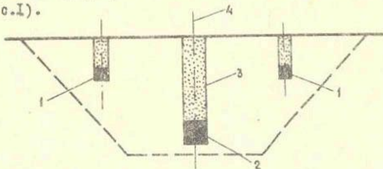
Рис.1. Схема расположения траншейных зарядов: 1 - вспомогательные заряды; 2 - основной заряд; 3 - забойка; 4 - ось выемки
