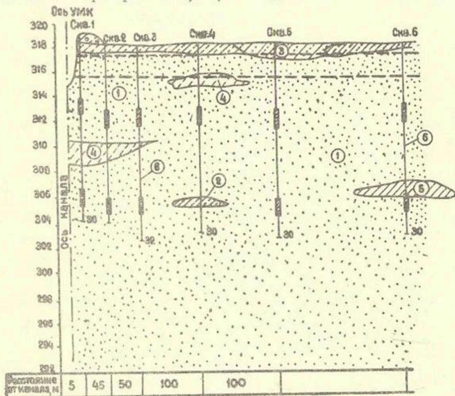
Рис.3. Гидрогеологический профиль режимного отвора I-I в совхозе № 26:
