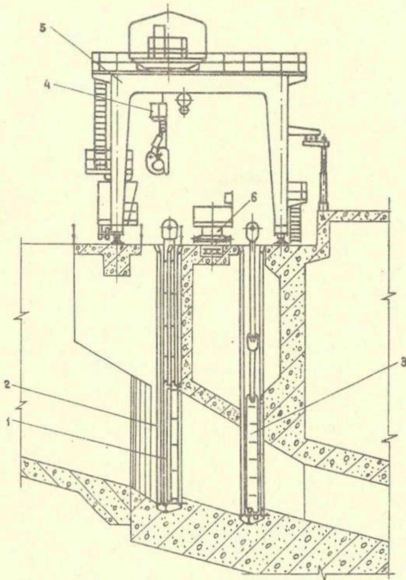
Рис. I. Компоновка механического оборудования нижнего бьефа насосной станции
