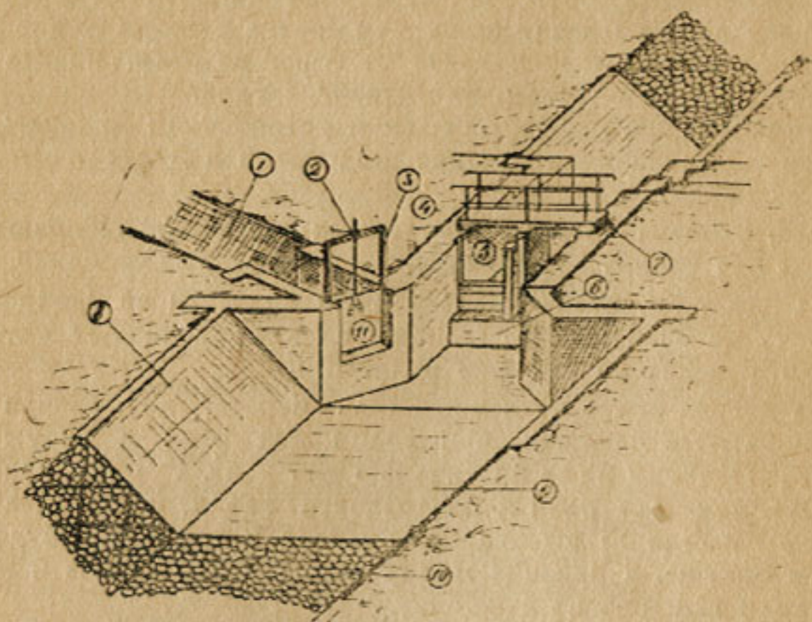
Рис. 2: 1) Водовыпуск, 2) подъем, 3) рама щита, 4) паз, 5) шандоры, 6) порог, 7) служебный мост, 8) бетонный откос, 9) бетонное дно, 10) крепление канала, 11) щит.
