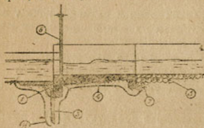
Рис. 1-а: 1) глинобетон, 2) линия фильтрации, 3) шпунт, 4) флютбет, 5) отмокки, 6) щит, 7) обратный фильтр (гравий, крупный песок)
