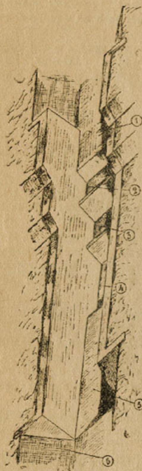
Рис. 3: 1) вход, 2) колодец 1-й ступ., 3) колодец 2-й ступ., 4) успокоит. колодец, 5) выход, 6) откос
