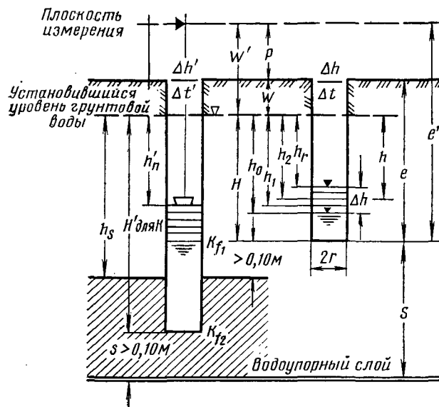
Рис. 3.12. Схема измерения водопоницаемости в буровой скважине [3.3].
