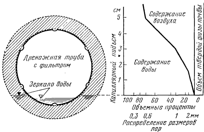
Рис. 5.12. Содержание воды и воздуха в дренажном фильтре из коксового волокна при частичном заполнении водой дренажной трубы [5.7].
