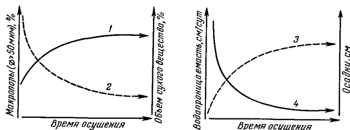
Рис. 7.9. Влияние осушения торфяного болота на структуру, осадку и водопроницаемость торфа [7.3]:
