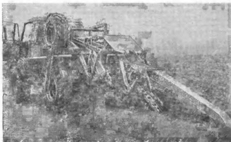
Рис. 9.8. Фрезерный траншеекопатель на тягаче «Униномг».
