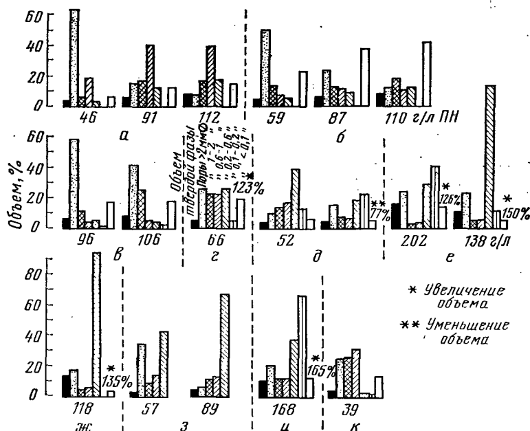
Рис. 8.13. Распределение объема пор в некоторых дренажных фильтрующих материалах [5.6]: а — кокосовое волокно; б — ржаная солома; в — древесная шерсть; г — волокнистый торф (филтан без картона); д — акриловискозная смесь (дуо); е — полиэфирное волокно (фибертекс, тревираспунбоид); ж — полипропилен (влинт); з — стеклянная шерсть (мсфи); и — стеклоткань; к — полнуретановый пенопласт.
