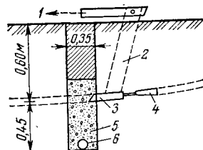
1 — направление тяги; 2 — нож (стальная полоса толщиной 3 см, заостренная спереди); 3 — кротователь сечением 8 см; 4 — уширитель в виде прицепной конусообразной болванки сечением 10 см; 5 — фильтрующий слой над гончарными трубами; 6 — гончарная труба.
