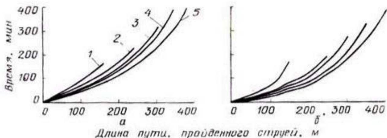
Рис. 30. Зависимость длины пути, пройденного струями разной величины по дну борозды, от времени:
