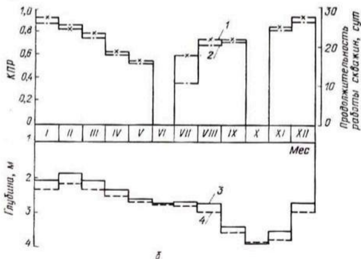
Рис. 13. График режима откачек из скважин вертикального дренажа: а — мелиоративный период; б — эксплуатационный период; 1 — продолжительность работы скважины, 2 — коэффициент полезной работы (КПР), 3 — глубина грунтовых вод, м, 4 — глубина напорных вод, м
