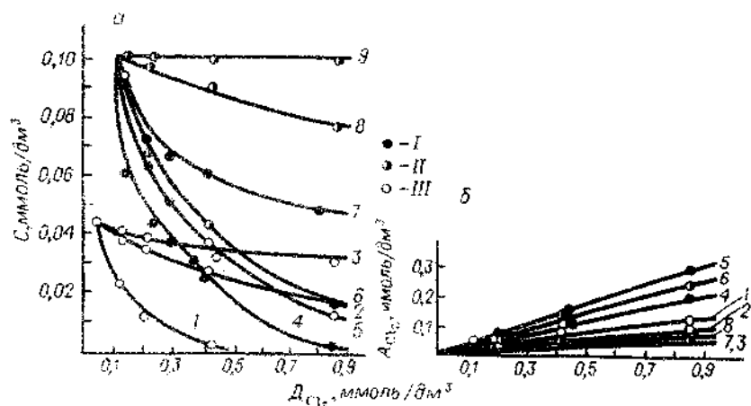
Рис. 25. Разложение феноурана (I), которана (II), диурана (III) (а) и поглощенного ими хлора (б) в зависимости от дозы введенного реагента
