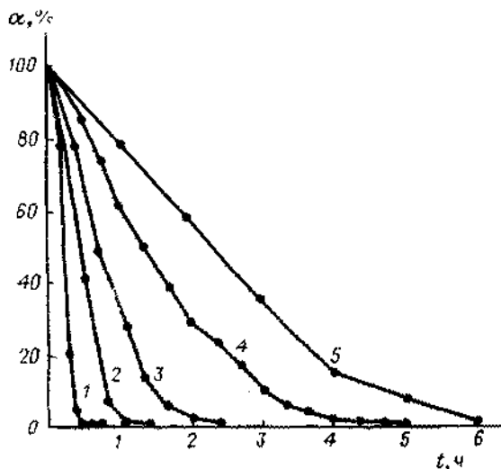
Рис. 38. Степень разложения параквата при озонировании с одновременным УФ-облучением (в присутствии 5 % ацетона)
