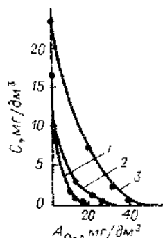
Рис. 29. Изменение концентрации диурана (1), феноурана (2), которана (3) в зависимости от содержания поглощенного озона
