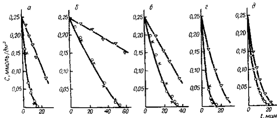
Рис. 18. Влияние pH на скорость разложения нитрофенолов озоном ( DO_3 = 5,8 \text{ мг/дм}^3 , скорость озono-воздушной смеси v_{OBC} = 0,8 \text{ дм}^3/\text{мин} ):
