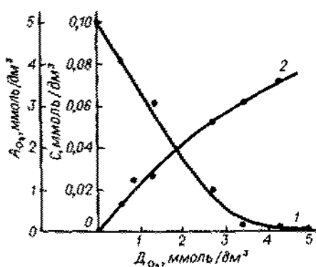
Рис. 15. Зависимость содержания прореагировавшего озона и концентрации цинбеа от дозы введенного озона:
