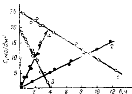
Рис. 32. Кинетика гидролитического разложения бутилового эфира 2,4-Д (1, 3) и накопления 2,4-Д (2, 4) pH: 1, 2 — 1,2; 3, 4 — 9,8
