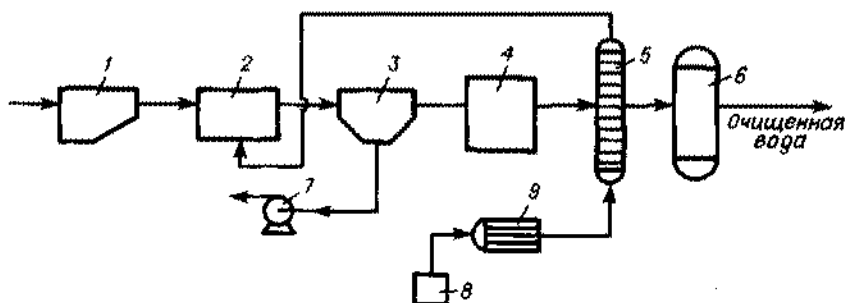
ис. 50. Технологическая схема очистки сточных вод от сложной смеси пестицидов: — накопитель; 2 — усреднитель; 3 — отстойник; 4 — песчаный фильтр; 5 — баротажная колонна; 6 — угольный фильтр; 7 — насосная станция; 8 — блок кондиционирования воздуха; 9 — озонатор
