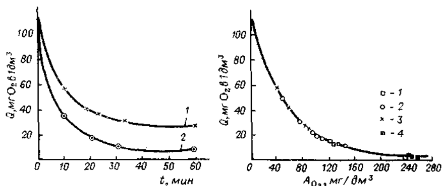
Рис. 46. Зависимость перманганатной окисляемости сточной воды ( Q ) от времени озонирования
