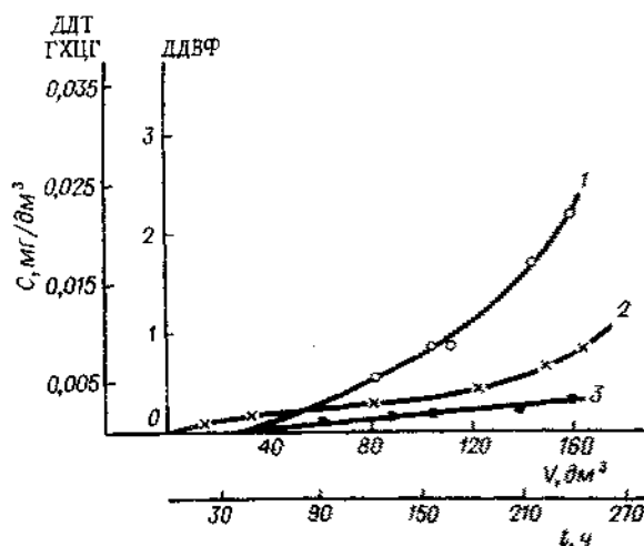
Рис. 31. Выходные кривые динамики адсорбции на угле АГ-3 загрязненных сточных вод производства препарата „Прима-71“: 1 — ГХЦГ; 2 — ДДВФ; 3 — ДДТ
