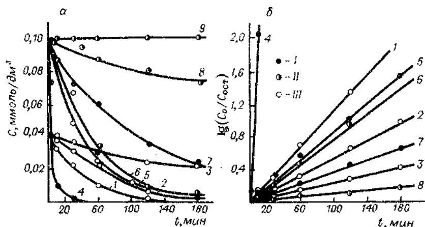
Рис. 27. Кинетические кривые (а) и их полулогарифмические анаморфозы (б) разложения фенурана (I), которана (II) и диурана (III) в условиях 10-кратного молярного избытка хлора рН: 1,4,6 — 4,0; 2,5,8 — 10,5; 3,7,9 — 7,0
