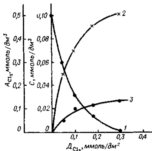
Рис. 8. Зависимость содержания прореагировавшего хлора и концентрации эптама и дипропиламина от дозы введенного хлора: 1 – эптам; 2 – дипропиламин; 3 – хлор
