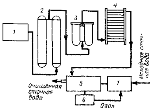
Рис. 48. Принципиальная технологическая схема очистки сточных вод озонотом:
