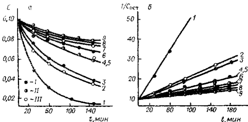
Рис. 26. Кинетические кривые образования N-хлорпроизводных фенола (I), которана (II), диурона (III) и их линейные анаморфозы (б) pH: 1,2,4 — 4,0; 3,5,6 — 9,0; 7,8,9 — 7,0
