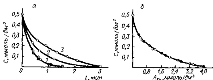
Рис. 13. Зависимость концентрации дипропиламина от времени ( t ) обработки ( a ) и содержания A_{O_3} прореагировавшего озона ( b ) Скорость подачи озono-воздушной смеси, dm^3/min : 1 — 23,4 ( \circ ), 17,6 ( \bullet ), 15,0 ( \circ ); 2 — 11,3; 3 — 6,1
