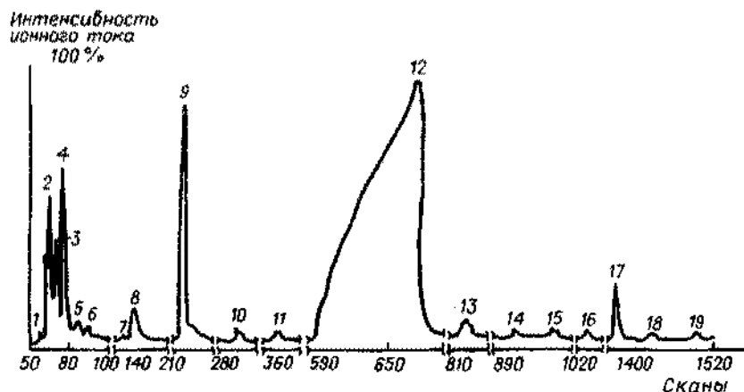
ис. 17. Хроматограмма продуктов разложения 2-метил-4,6-динитрофенола хлором pH_{исх} 6,8 ; pH_{кон} 2,4 ; C_{исх} = 0,1 ммоль/ dm^3 ; соотношение реагентов 1:25; скорость скакирования — 1 масс-спектр/с):
