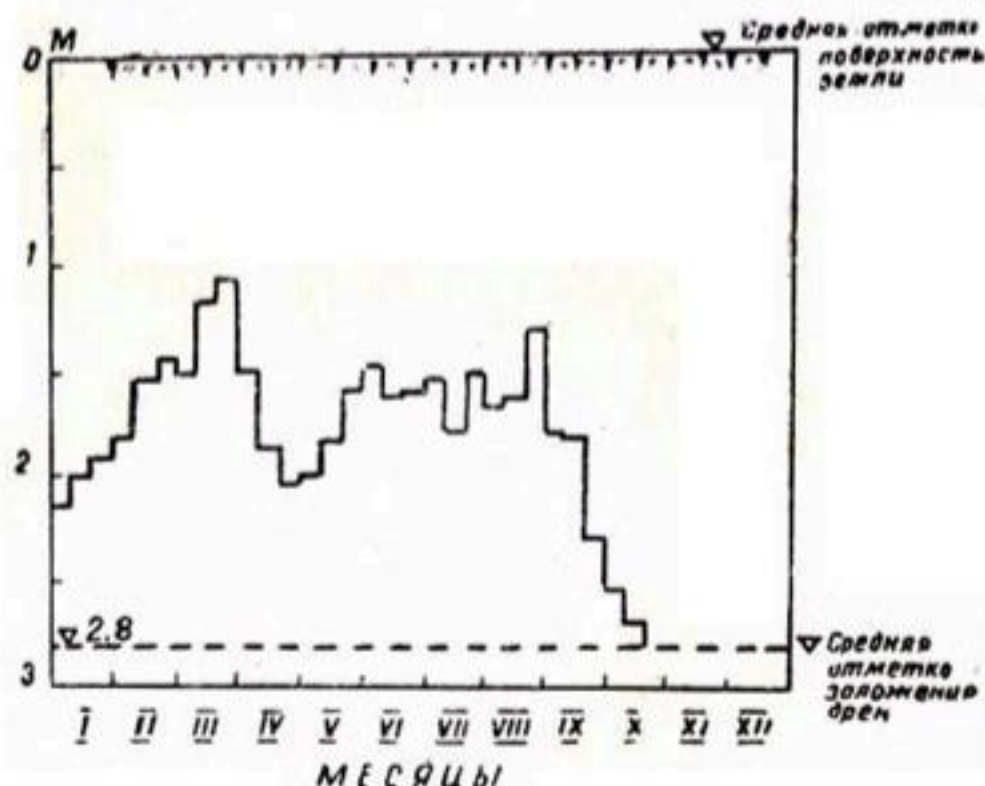
Рис. 5. Динамика среднего уровня грунтовых вод на опытном участке закрытого дренажа в 1964 г.
