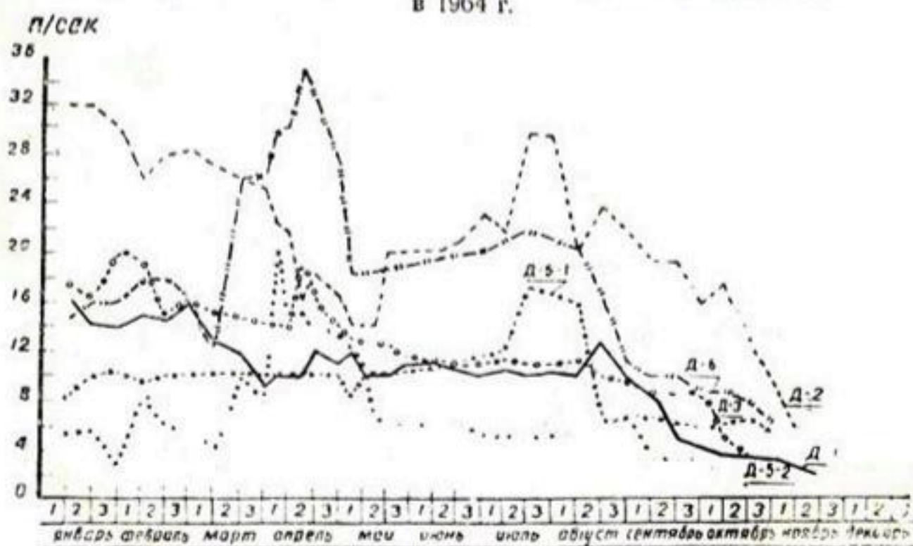
Рис. 3. Колебания расходов воды в устьях закрытых дренах на опытном участке в 1964 г. (по данным одновременных замеров).
