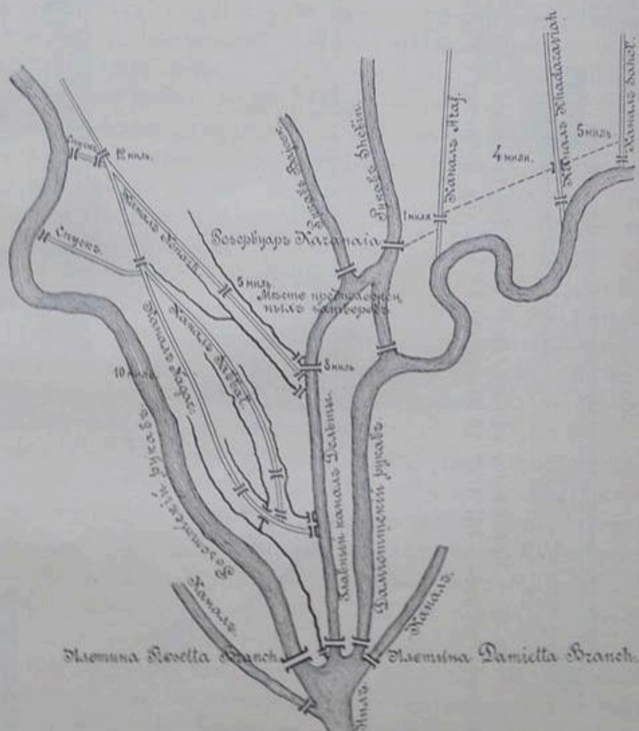
Черт. 31. — Планъ части дельты р. Нила съ указаніемъ расположенія плотинъ и каналовъ.
