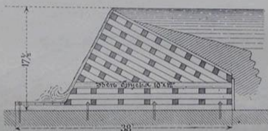
Черт. 21. — Поперечное сѣченіе плотины на р. Беар.
