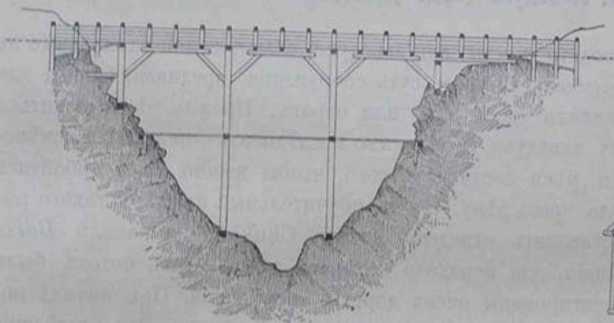
Черт. 79. — Деревянный желобъ на каналѣ Uncomrahgre.
