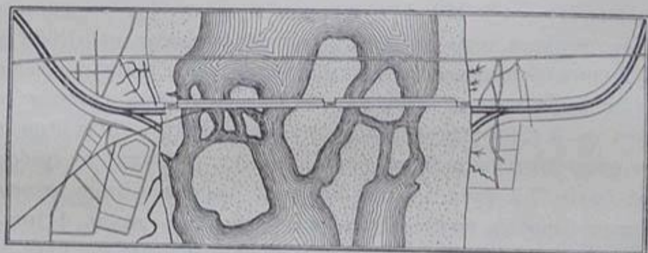
Черт. 36. — Головные сооруженія каналовъ на рѣкѣ Sone.
