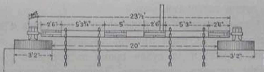
Черт. 59. — Ворота для подниманія затворовъ.
