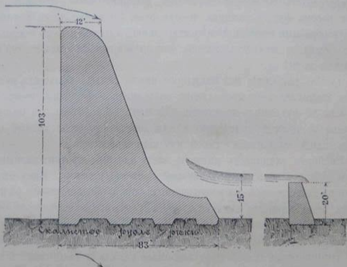
Черт. 45. — Поперечное сѣченіе плотины Turlock.
