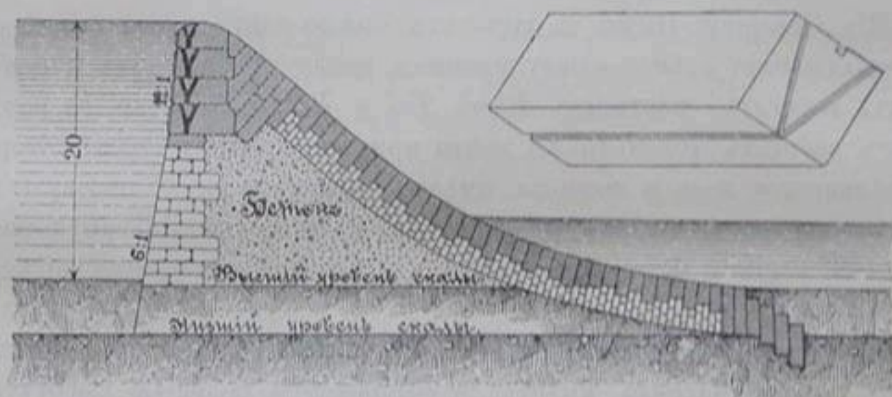
Черт. 46. — Плотина канала Хенаресъ.
