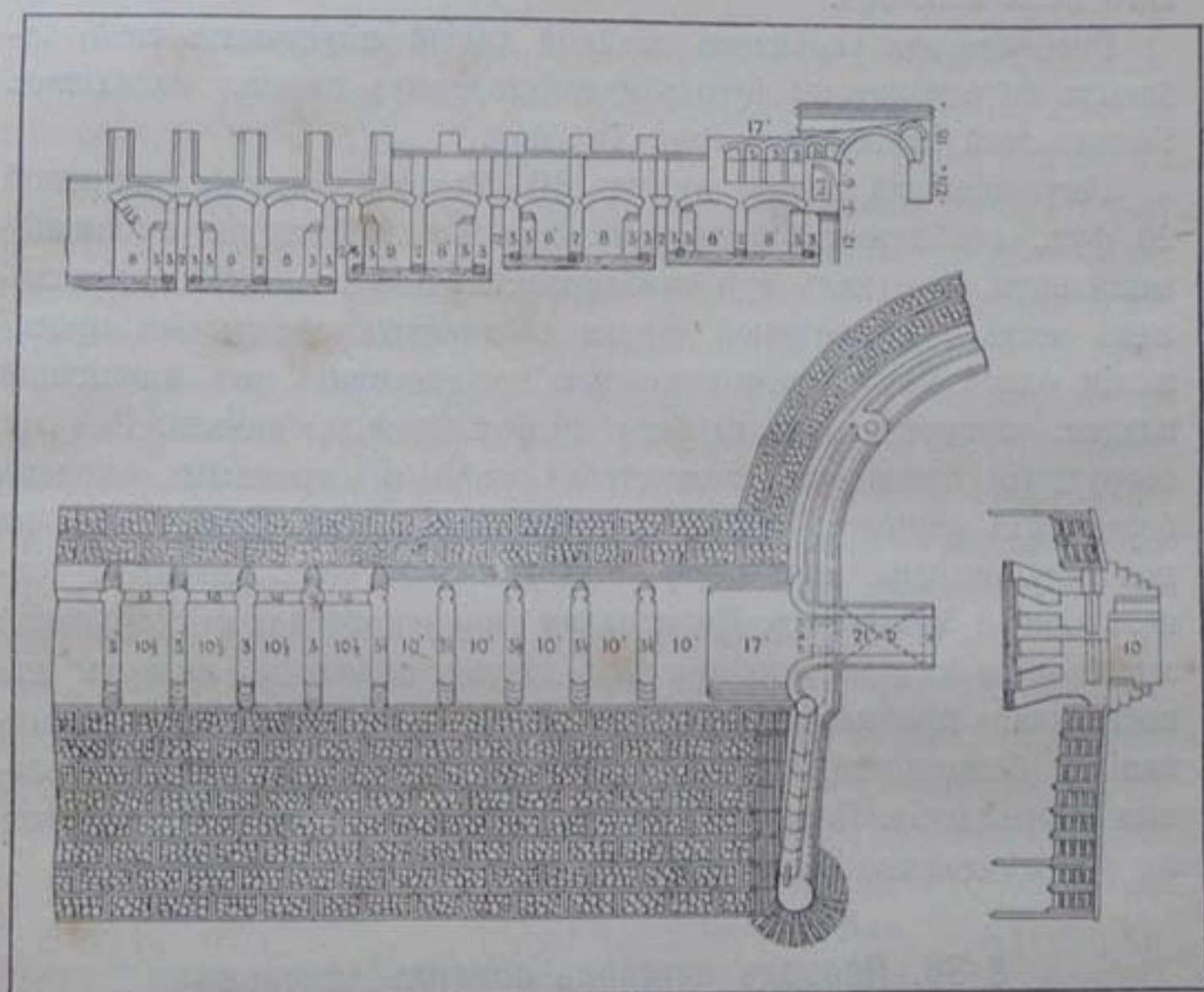
Черт. 94. — Пересѣченіе въ одномъ уровнѣ Гангесскаго канала.
