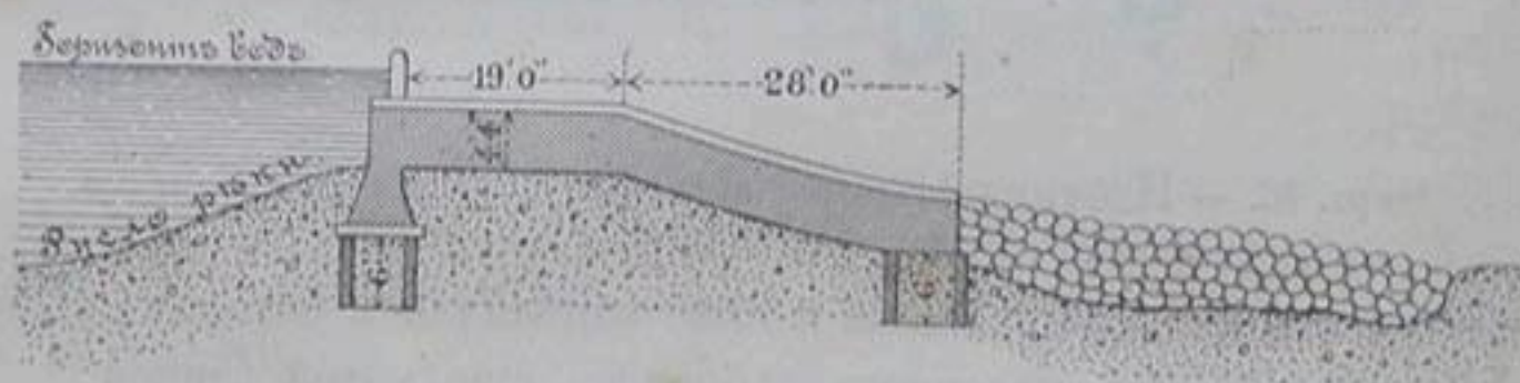
Черт. 44. — Аникуть Годавери.
