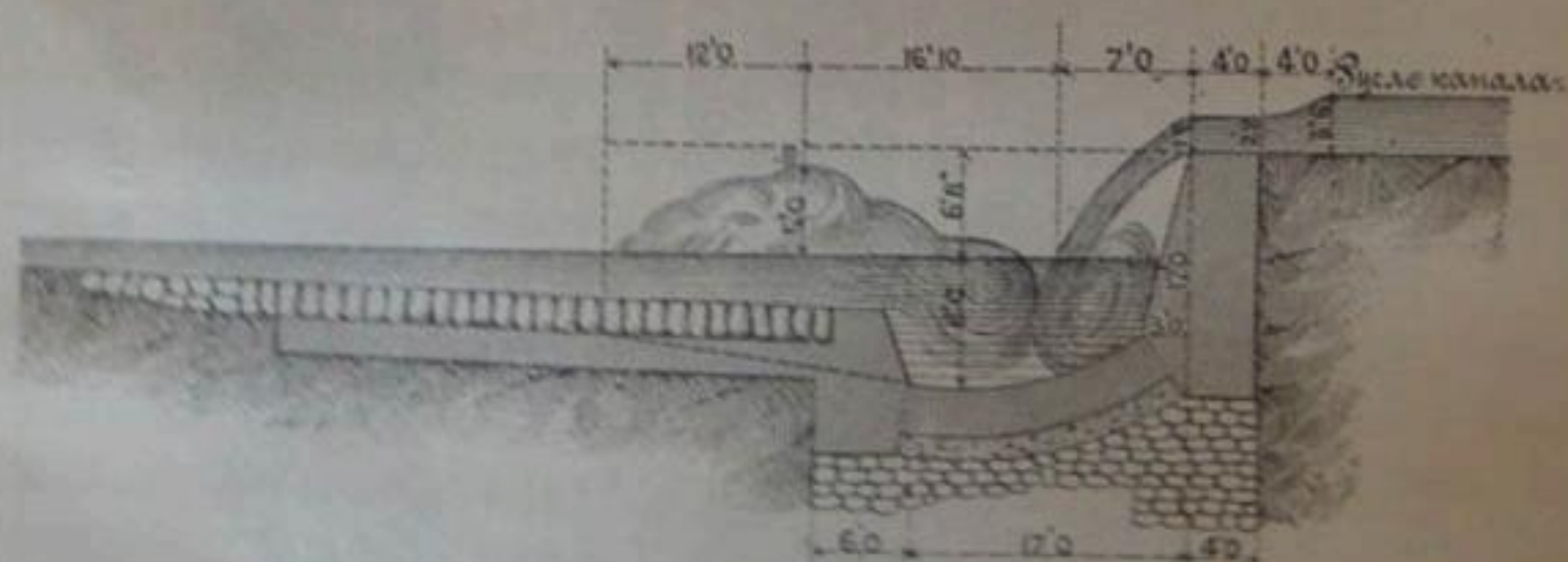
Черт. 114. — Продольное сѣченіе водослива на каналѣ Bagee Doab.
