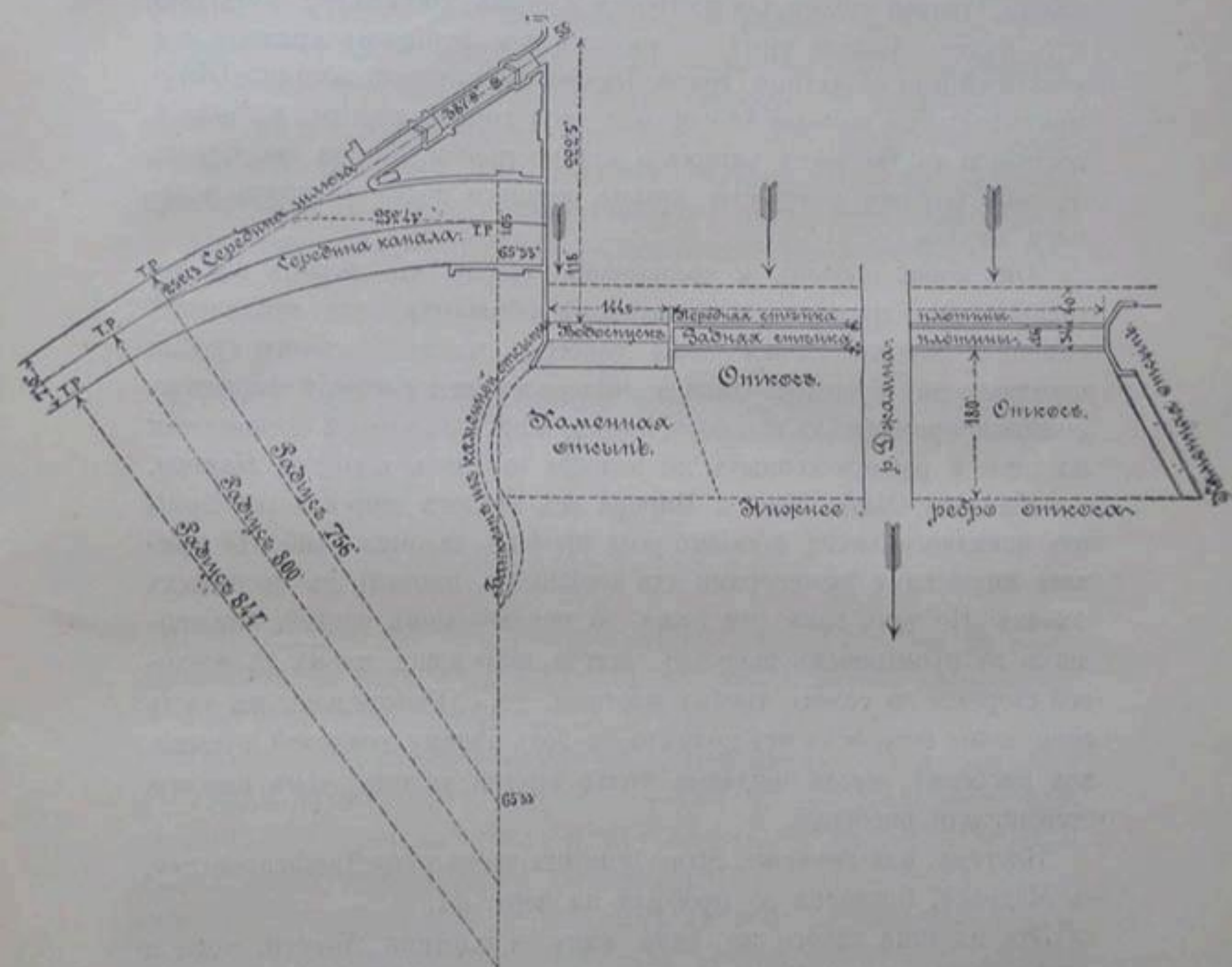
Черт. 40. — Плотина Okhla.
