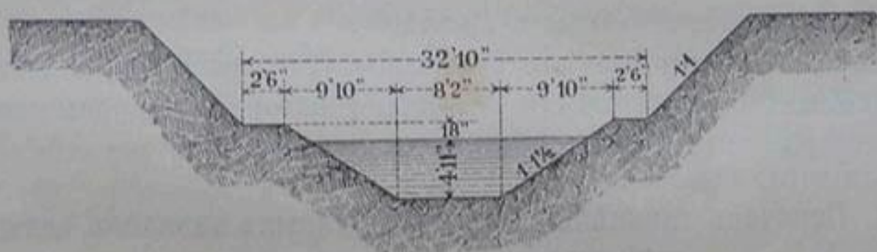
Черт. 9. — Каналь Хенаресь въ Испаніи.
