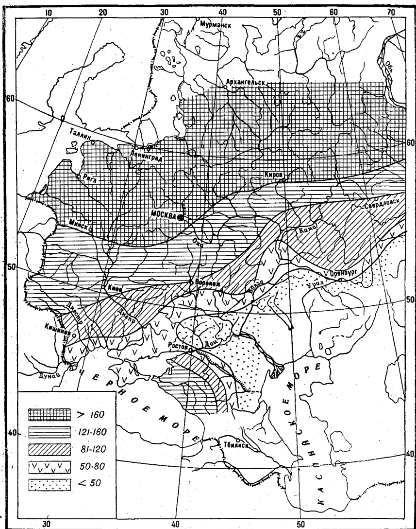
Рис. 52. Ожидаемые запасы продуктивной влаги в метровом слое почвы (в мм) под яровыми культурами в период колошения в 1957 г.
