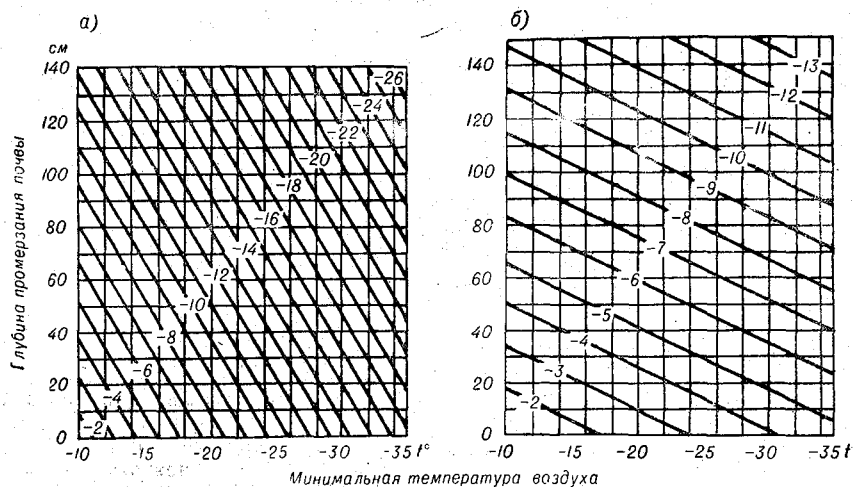
Рис. 11. Зависимость минимальной температуры почвы на глубине залегания узла кущения озимых от минимальной температуры воздуха и глубины промерзания почвы при высоте снежного покрова 5 см (а) и 10 см (б).
