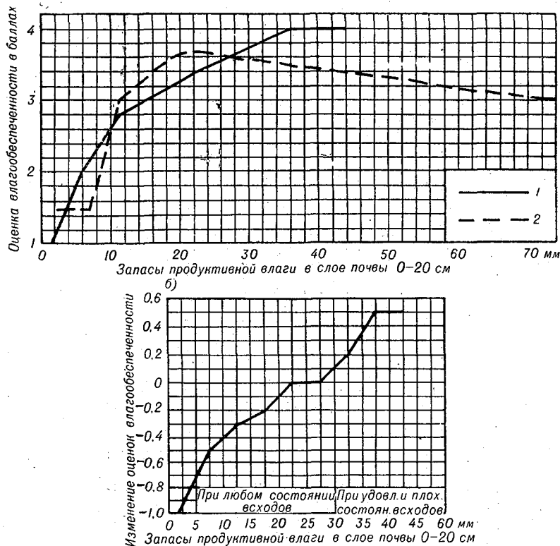
Рис. 49. Оценка влагообеспеченности посевов по запасам продуктивной влаги в почве.
