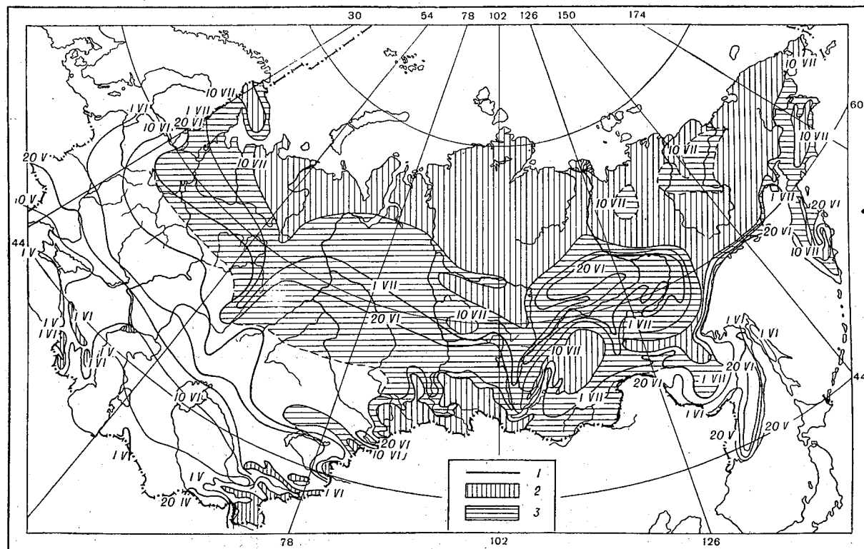
Рис. 32. Самые поздние возможные весенние заморозки в воздухе.
