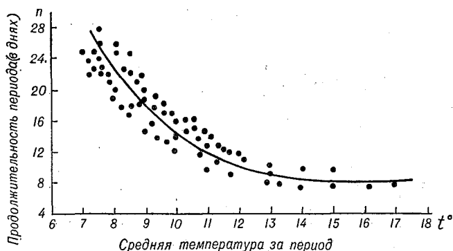
Рис. 3. Зависимость продолжительности периода всходы — кушение озимой ржи от средней температуры за период (при хорошем увлажнении почвы, 30—60 мм в слое 0—20 см).
