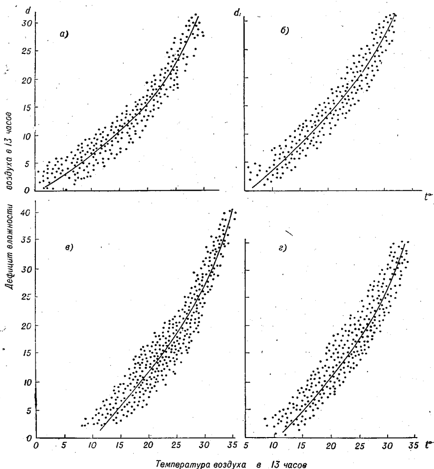
Рис. 55. Связь между дефицитом влажности воздуха и температурой воздуха в 13 часов в дни без дождя (для континентальных станций).
