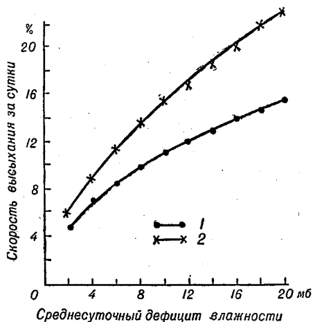
Рис. 73. Зависимость скорости высыхания колосовых хлебов от среднесуточного дефицита влажности. 1 — сухая зона, 2 — влажная зона.
