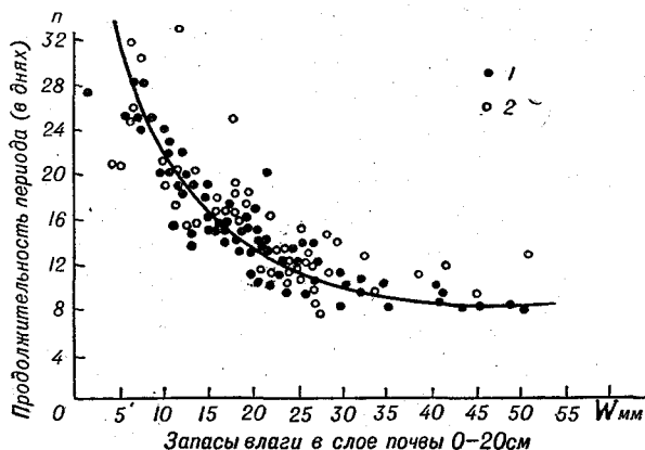
Рис. 4. Зависимость продолжительности периода всходы — кушение озимой ржи и озимой пшеницы от увлажнения почвы (при температуре выше 13^{\circ} ). 1 — озимая рожь, 2 — озимая пшеница.
