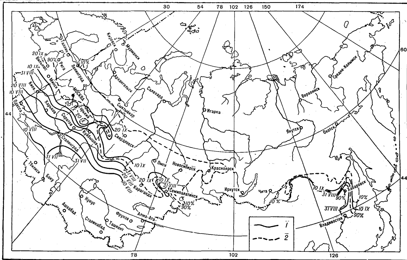
Рис. 36. Средние многолетние сроки созревания кукурузы скороспелых сортов типа Первенец и наступления молочной зрелости початков среднеспелых сортов типа Миннезота 13 (1) и обеспеченность (в %) наступления обеих фаз (2).
