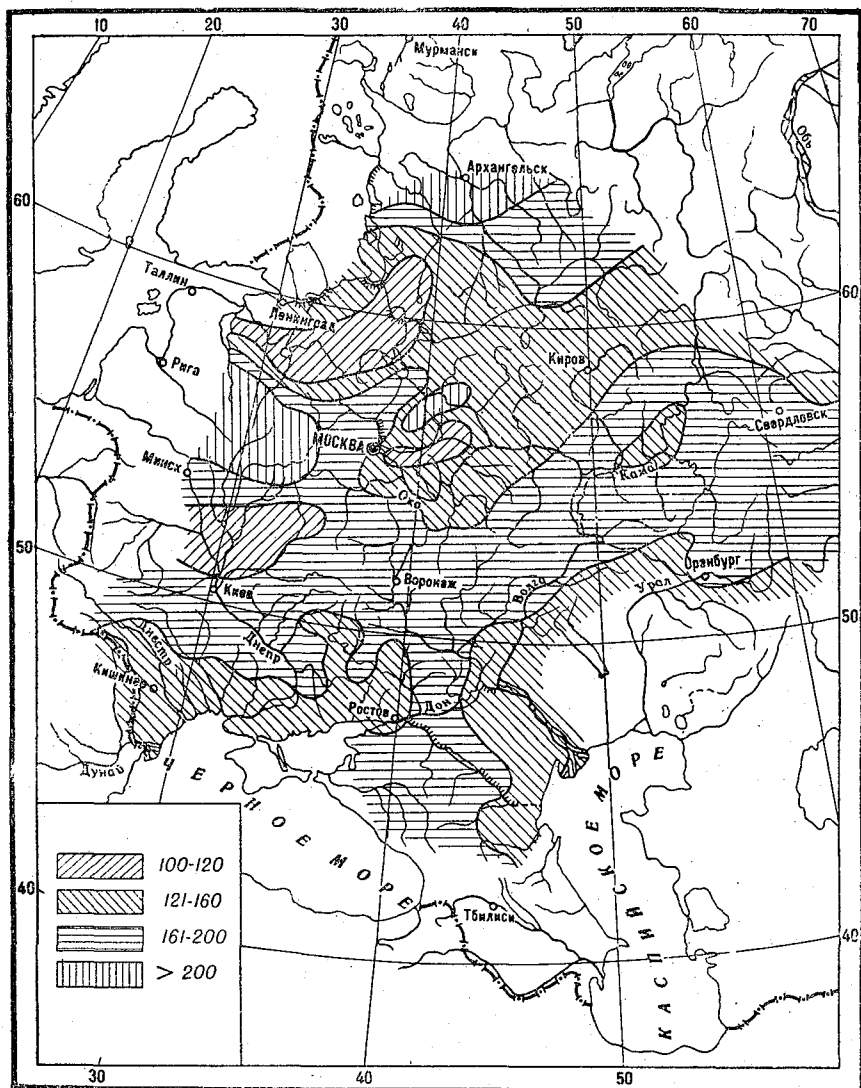
Рис. 18. Наименьшая полевая влагоемкость почв (в мм) на Европейской территории СССР (по А. В. Прохорову).
