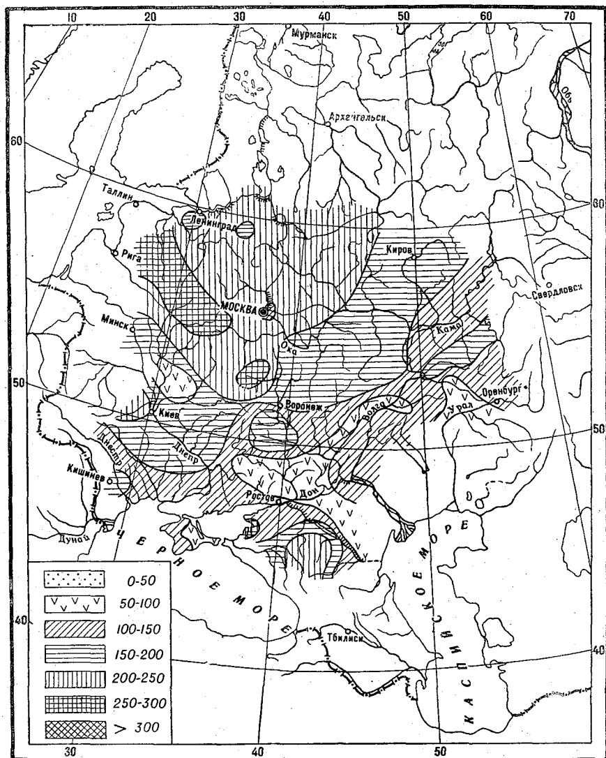
Рис. 20. Средние многолетние запасы продуктивной влаги (в мм) в метровом слое почвы по зяби на Европейской территории СССР в момент перехода средней суточной температуры воздуха через +5^{\circ} весной.
