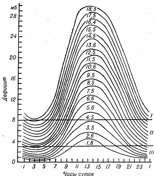
Рис. 74. Суточный ход дефицита влажности воздуха при различных средних его значениях (числа в средней части кривых).
