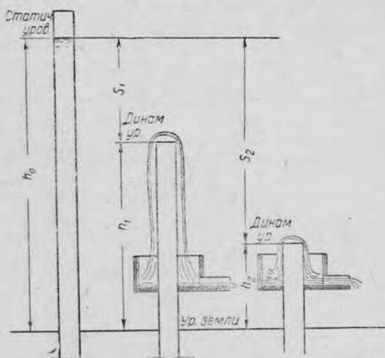
Рис. 3. Измерение дебита самонизливающих скважин.
