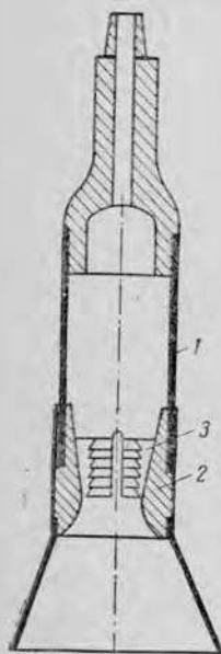
Рис. 86. Шлиц: 1 — корпус шлица; 2 — конус; 3 — прокладки.
