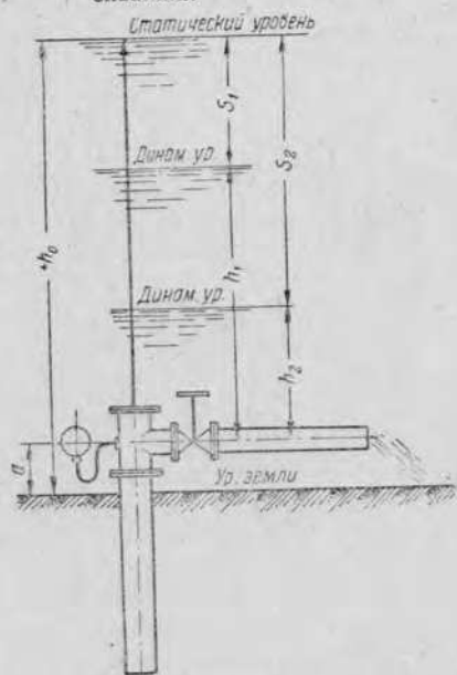
Рис. 4. Измерение дебита самонизливающих скважин при высоком пьезометре.
