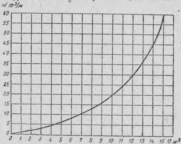
Рис. 48. График для определения объема ресивера.
