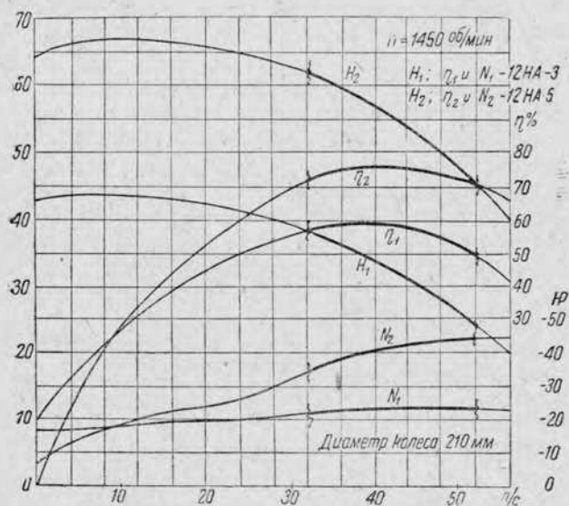
Рис. 35. Характеристика насоса 12-НА.
