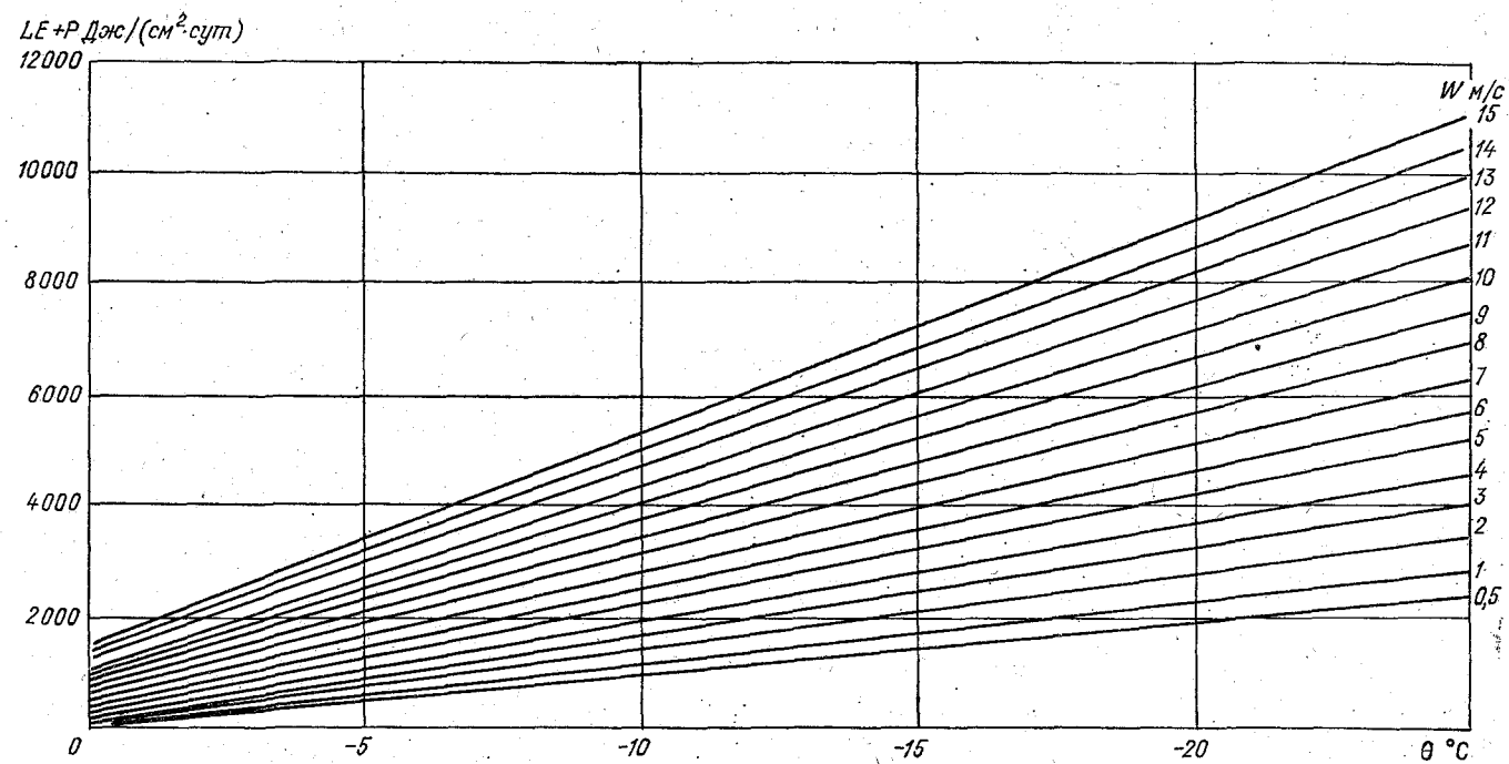
Рис. 1.3. Номограмма для определения суммы тепловых потоков испарения и теплообмена с воздухом ( LE+P ) при температуре поверхности воды \theta ^{\circ}\text{C} .
