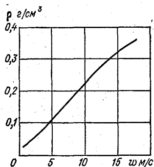
Рис. 4.5. Связь плотности свежавпавшего сухого снега \rho со скоростью ветра w .
