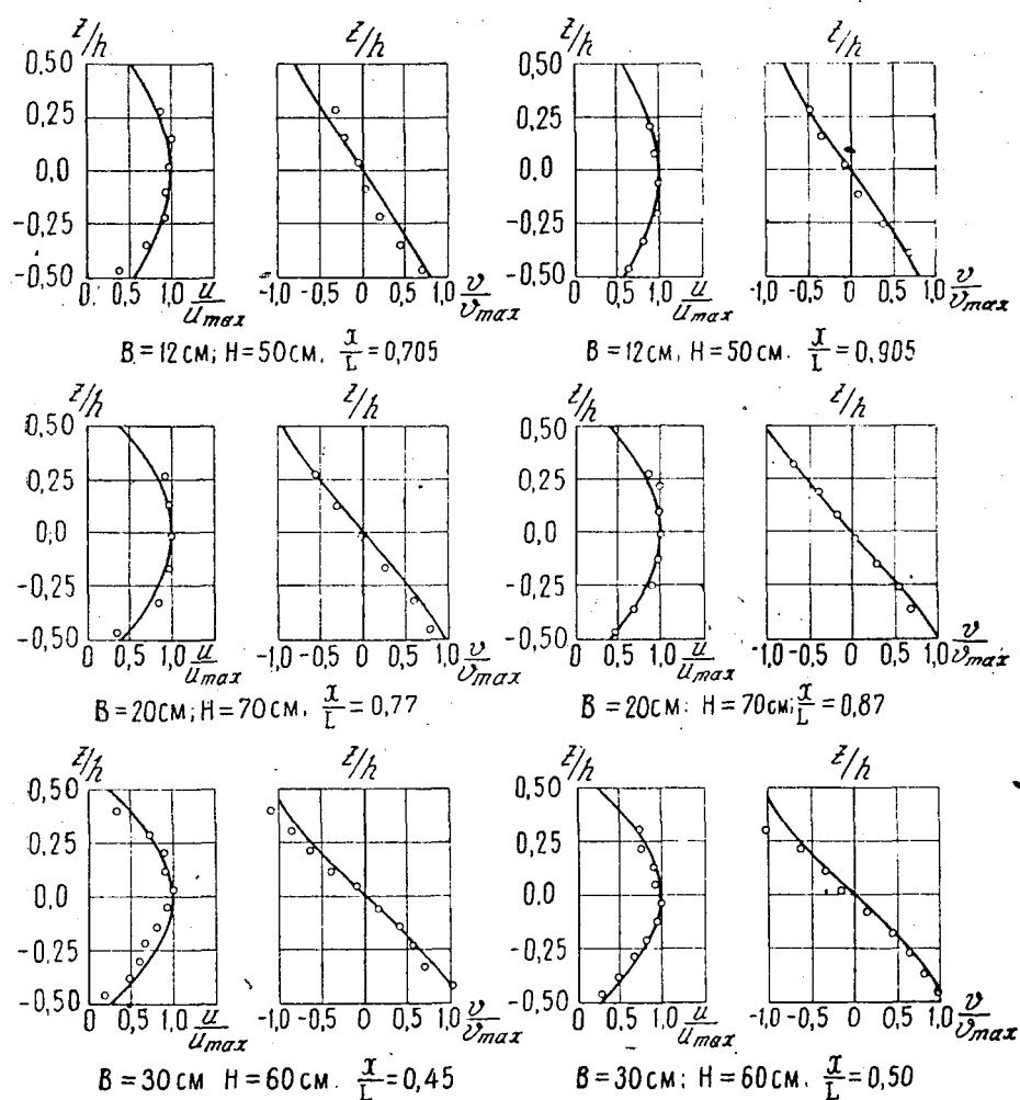
Рис. 3. Расчетные и опытные профили составляющих скорости в поперечных сечениях потока при различных величинах его ширины ( B ) и напорах ( H ).
