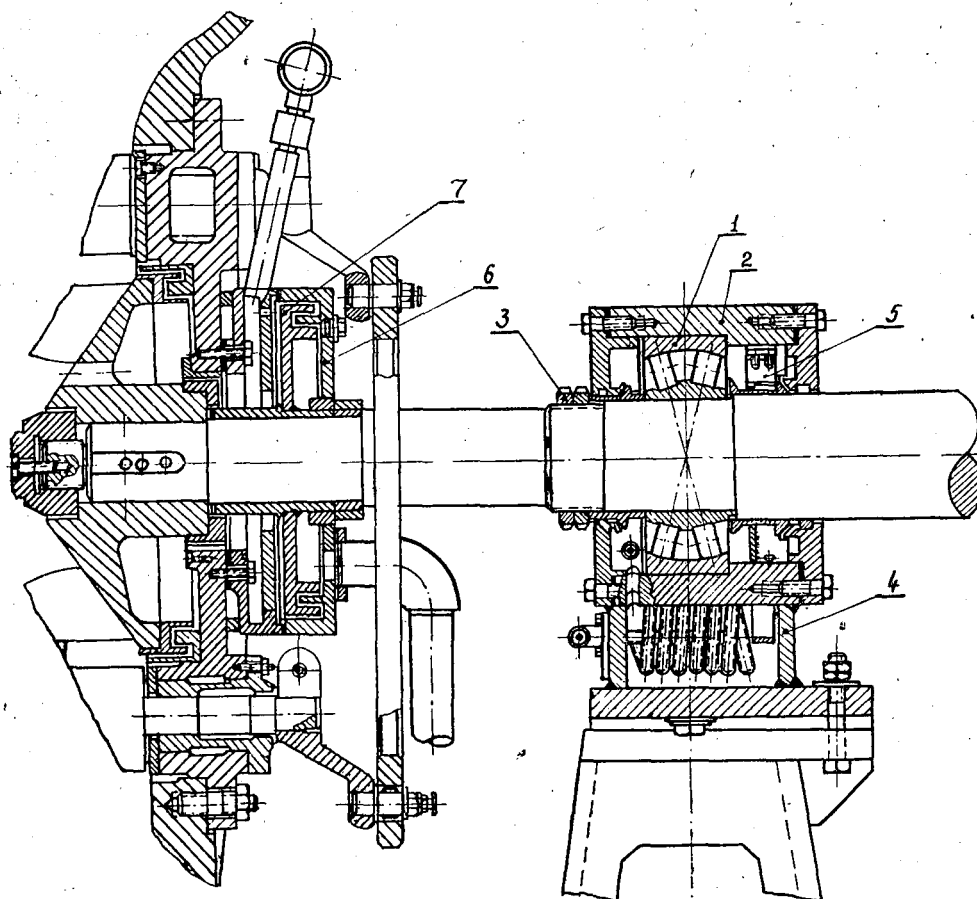
Рис. 2. Радиально-упорный подшипник, выполненный сочетанием двухрядного сферического роликоподшипника с разгрузочным устройством на турбине.
