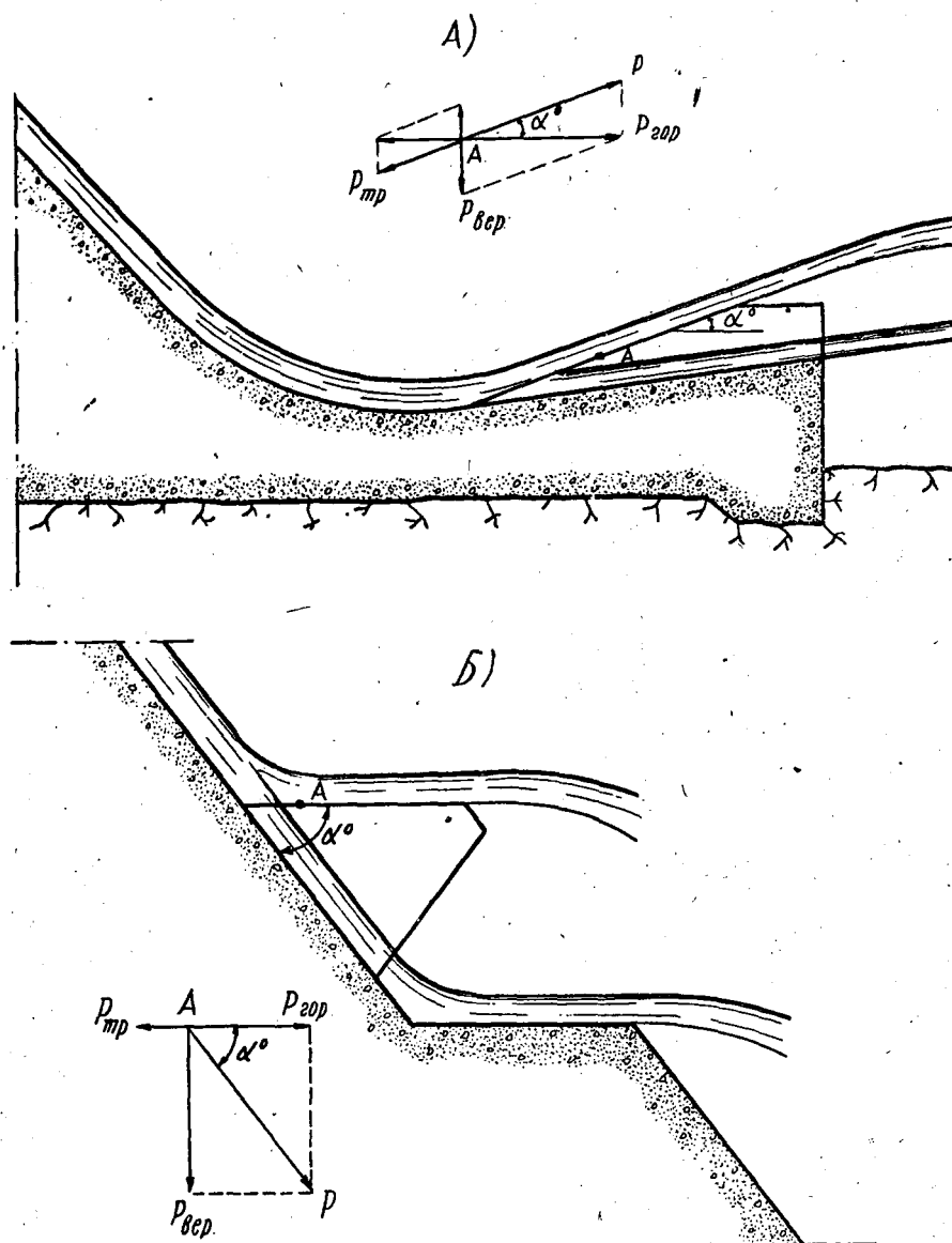
Рис. 1. Схемы сил, действующих на расщепитель.
