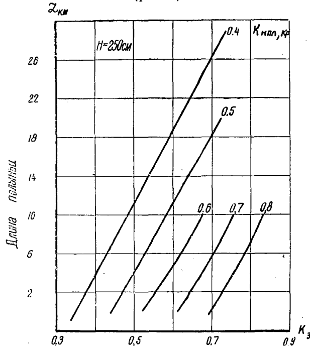
Рис. 2. Зависимость «зимнего» коэффициента ( K_z ) р. Иртыш от длины полыньи ( L ), значения «зимнего» коэффициента на нижней кромке ее ( K_{нпл.кр} ) и уровня значениями K_{пл} оз. Зайсан над нулем графика водомерного поста Топольев Мыс ( H ).
