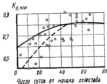
Рис. 3. Зависимость «зимнего» коэффициента, вычисленного по уровню нижней поверхности ледяного покрова ( K_{нпл} ) р. Иртыш у с. Камышенка от числа суток с начала ледостава.
