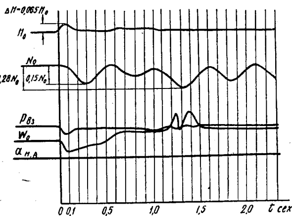
Рис. 2. Осциллограмма сброса мощности гидроагрегата вводом воздуха в отсасывающую трубу.
