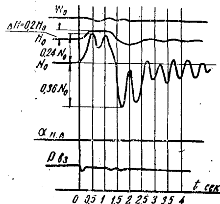
Рис. 3. Осциллограмма сброса мощности гидроагрегата вводом воздуха в область входного патрубка спиральной камеры.
