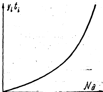
Рис. 2. Принципиальная кривая удельных аварийных ущербов в зависимости от глубины дефицита.
