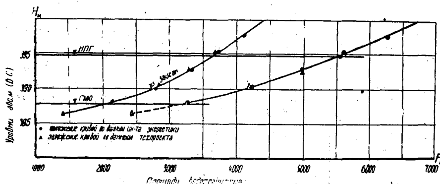
Рис. 7. Зависимость площади озерной части и всего Бухтарминского водохранилища в целом от уровня его наполнения.
