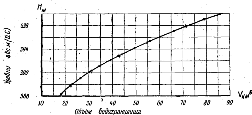
Рис. 8. Зависимость объема Бухтарминского водохранилища от уровня его наполнения по новой крупномасштабной съемке (0) и по данным технического проекта Бухтарминского гидроузла
