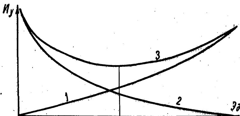
Рис. 5. Распределение дефицита по ЭВХК в целом.
