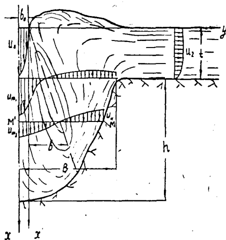
Рис. 1. Схема растекания струи в воронке размыва.
