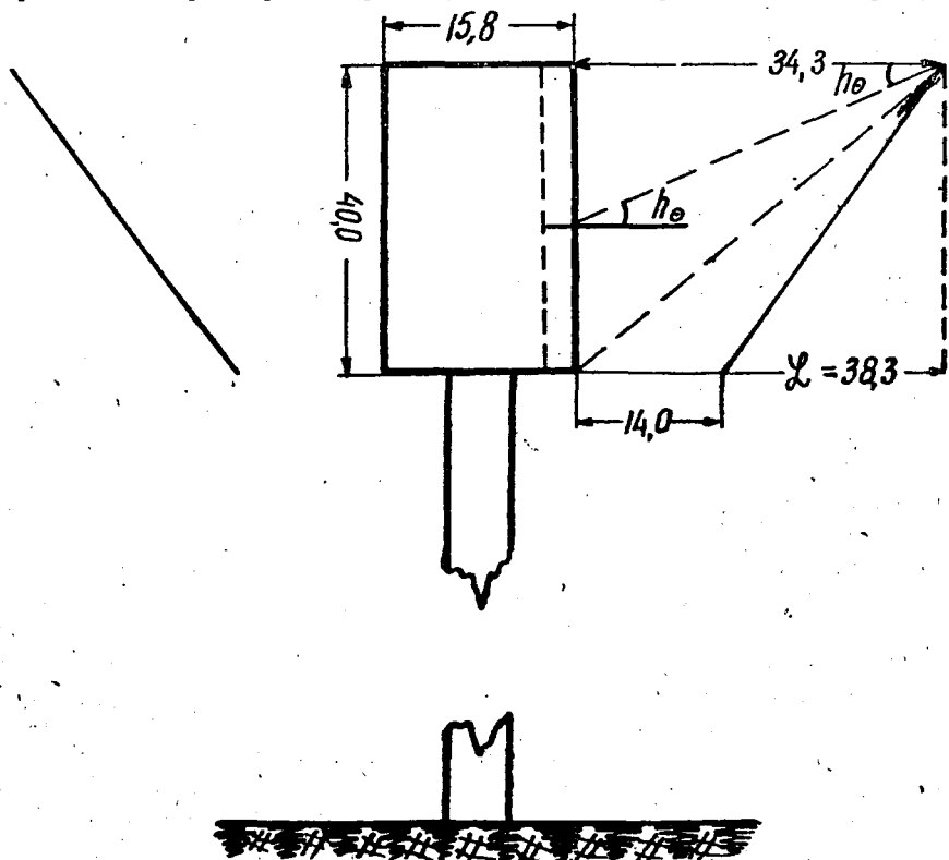
Рис. 2. Схема освещения Солнцем осадкомерного ведра осадкомера Третьякова.
