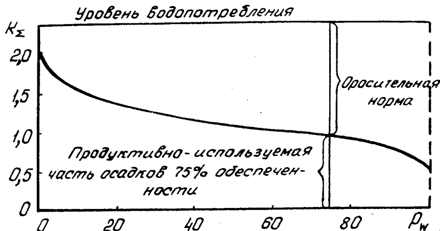
Рис. 4. Схема к расчету оросительной нормы.
