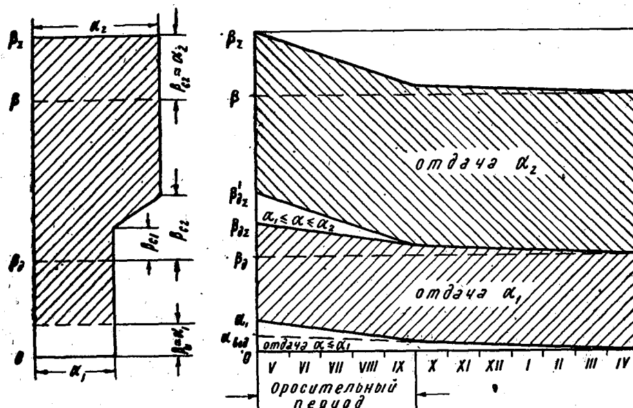
Рис. 6. Диспетчерский график при 2 ступенях отдачи водохранилища (для условий рек казахстанского типа питания).
