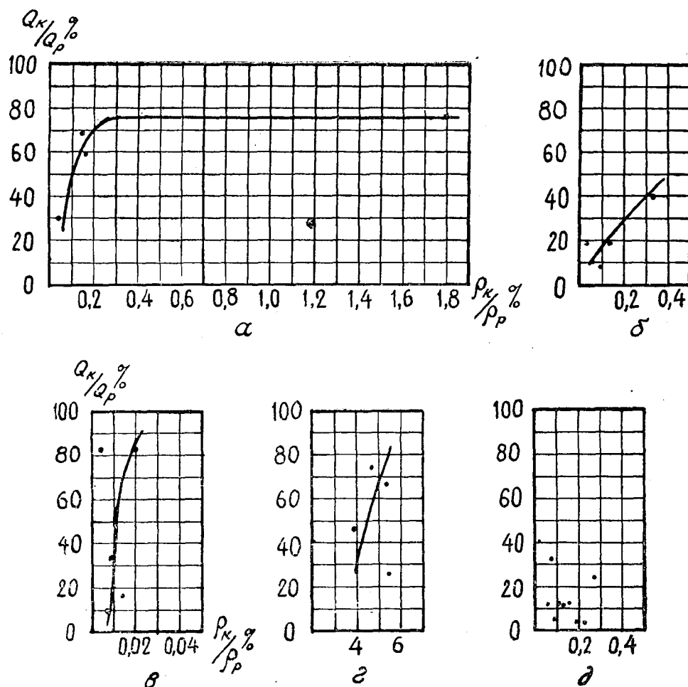
Рис. 1. Графики критерия качества работы модифицированных водозаборов ферганского типа: а — Кампыр-Раватский; б — Кугаратский; в — Иссыкский; г — Сары-Курганский; д — Ангренский.
