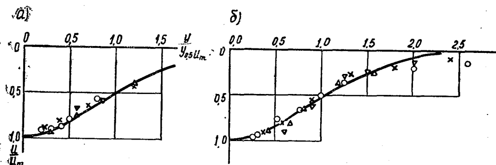
Рис. 5. Безразмерные профили скоростей в поперечных сечениях струи: а — обратное течение; б — прямое течение.
