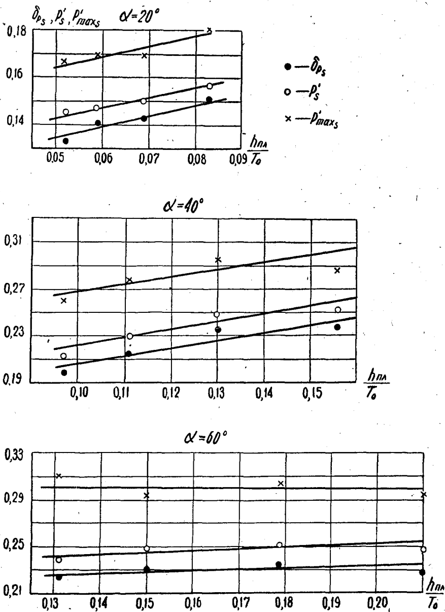
Рис. 2. Графики \delta p_s , p'_s , p'_{\max s} в зависимости от \frac{h_{\text{пол}}}{T_0} при синхронной записи пульсации давления.
