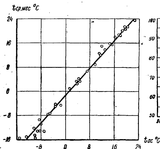
Рис. 5. График связи среднемесячной температуры воздуха ( t_{cp} ) и температуры воздуха в период выпадения осадков ( t_{oc} ).
