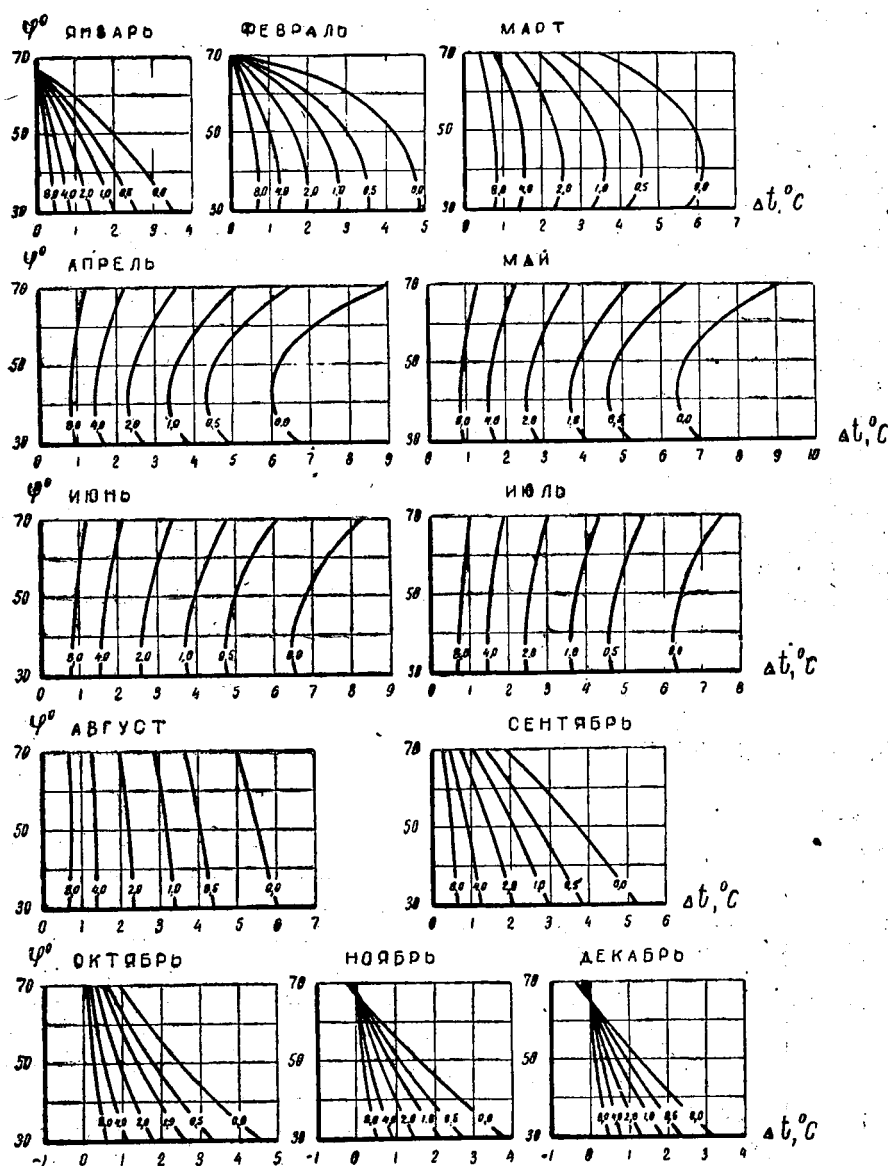
Рис. 4. Графики зависимости \Delta t от скорости ветра W_{200} , м/сек, широты местности ( \varphi^\circ ) и времени года.
