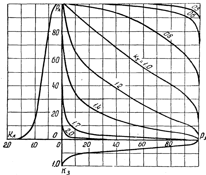
Рис. 3. Композиция кривых обеспеченности осадков летнего и зимнего периодов (м. с. Петропавловск).
