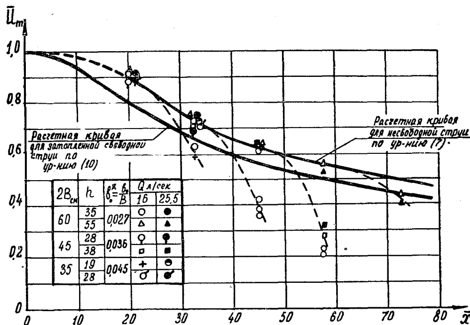
Рис. 4. Изменение безразмерной осевой скорости по длине тупика.
