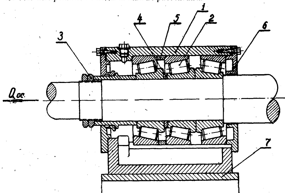
Рис. 1. Заводская конструкция радиально-упорного подшипникового узла.
