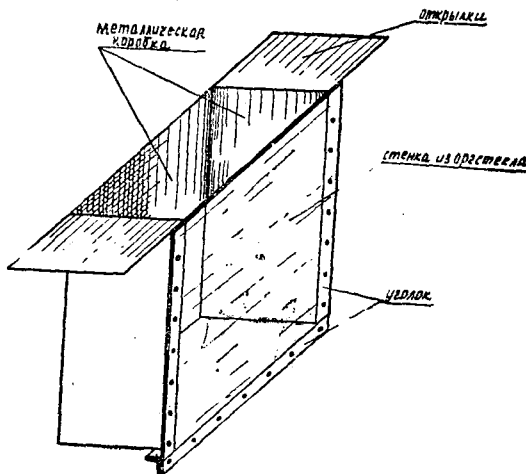
Рис. 2. Эскиз тупика.
