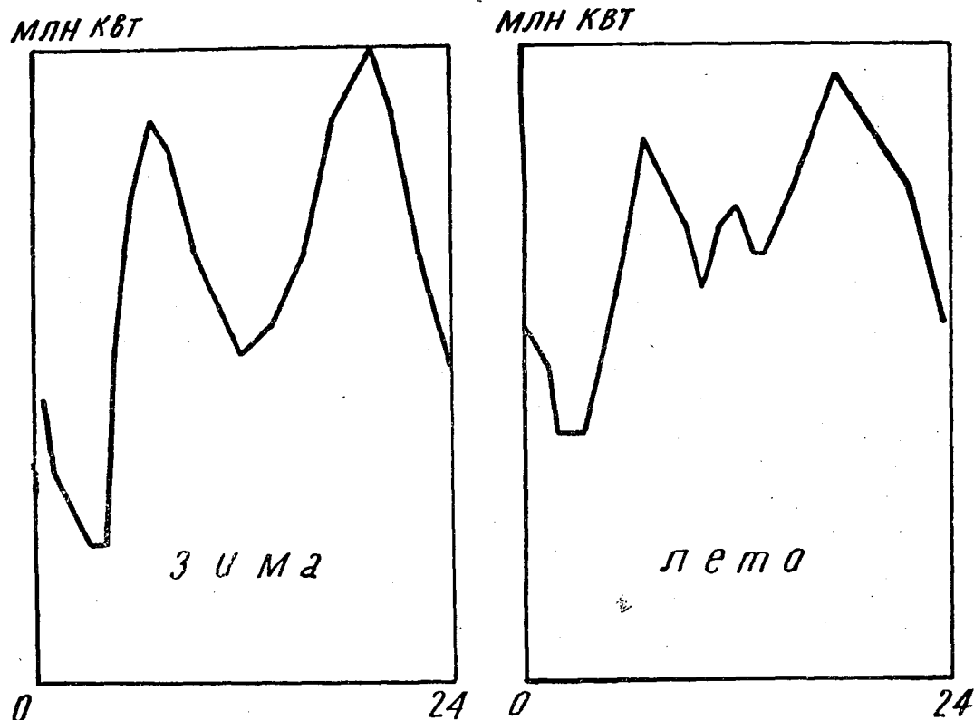
Рис. 1. Характерные графики нагрузки энергосистемы.
