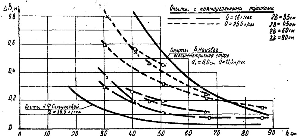
Рис. 2. Изменение осевого давления по длине тупика.
