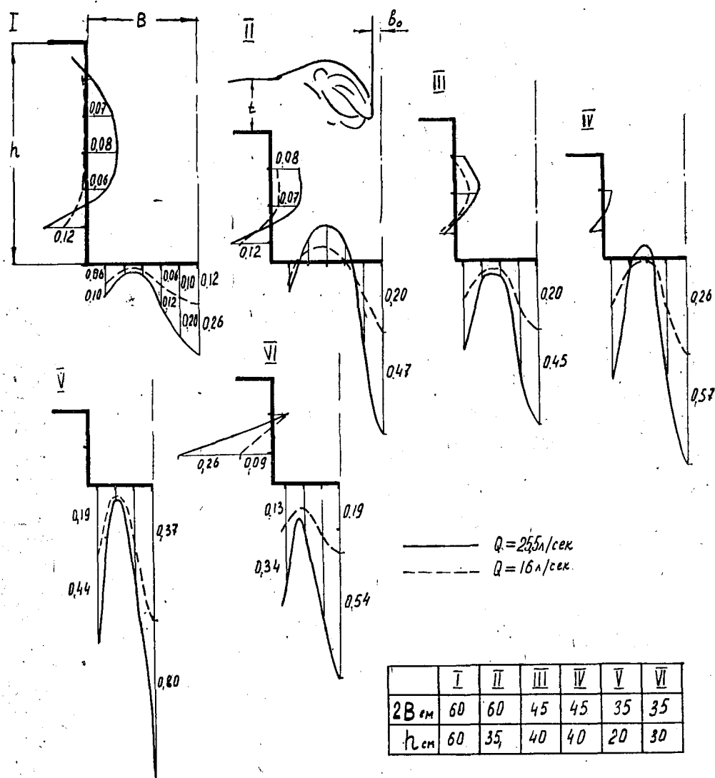
Рис. 1. Эпюры давления потока на дно и стенки тупика.
