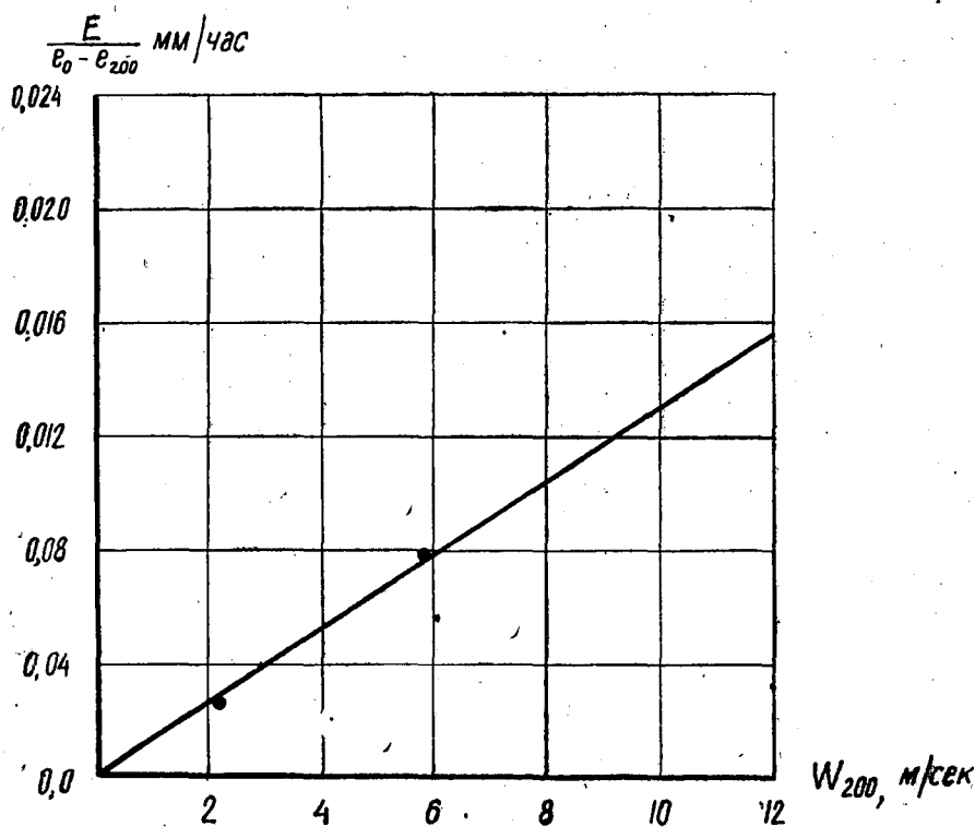
Рис. 1 Зависимость \frac{E}{e_0 - e_{200}} = f(W_{200}) для осадкомерного ведра осадкомера
