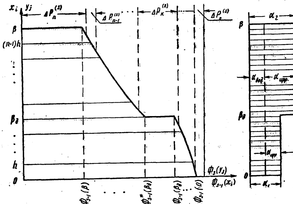
Рис. 1. К схеме регулирования стока на двух водопотребителей.
