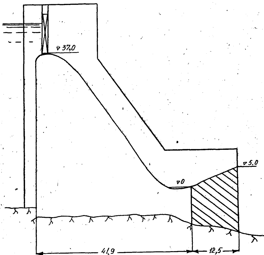
Рис. 1. Изменение конструкции носка водосливной плотины.
