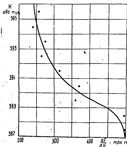
Рис. 6. Зависимость величины \frac{dF}{dH} от уровня воды в Бухтарминском водохранилище.
