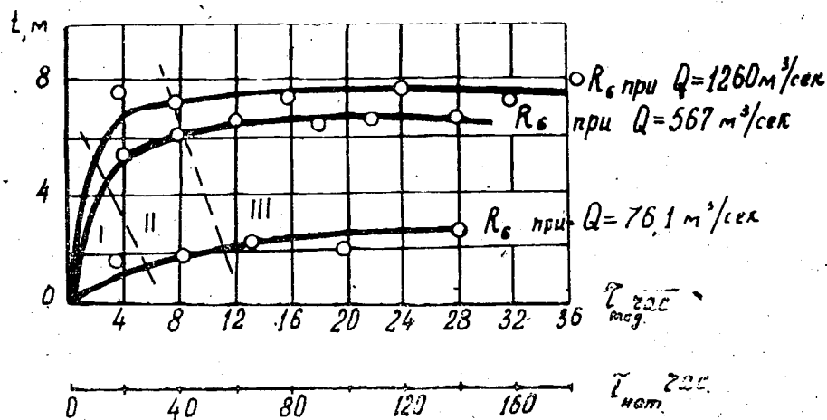
Рис. 3. Исследование на модели местного размыва скалы.
