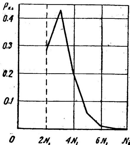
Рис. 3. Вероятность аварийного отключения потребителей электроэнергии, z=4 .
