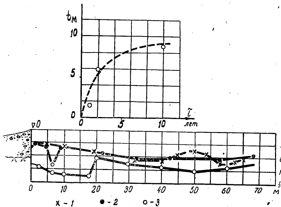
Рис. 4. Размыв скального дна в нижнем бьефе плотины. 1—1955, 2—1956, 3—1965 г.
