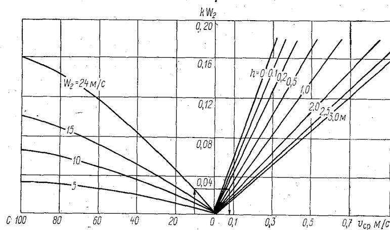
Рис. 5.2. Номограмма для определения v_{ср} ( C , W_2 , h ).
