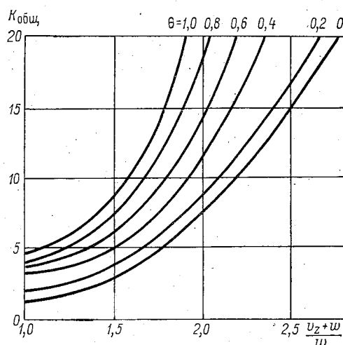
Рис. 4.4. Зависимость K_{общ} от безразмерных величин \Theta и \frac{v_z + w}{w} .
