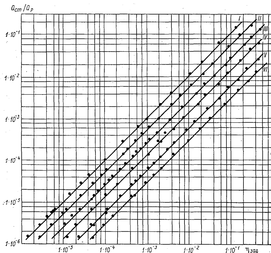
Рис. 4.8. Зависимость Q_{cm}/Q_p от \eta_{заг} .
